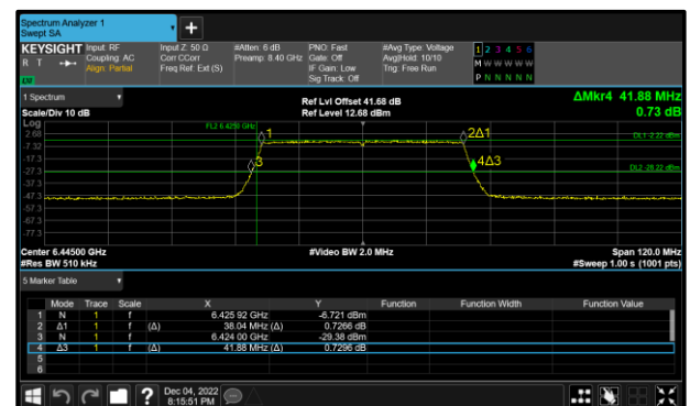
Figure 6 - 802.11ax HE40 SU Maximum 99% OBW
