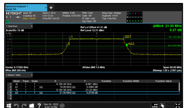
Figure 4 - 802.11ax HE20 SU Maximum 99% OBW
