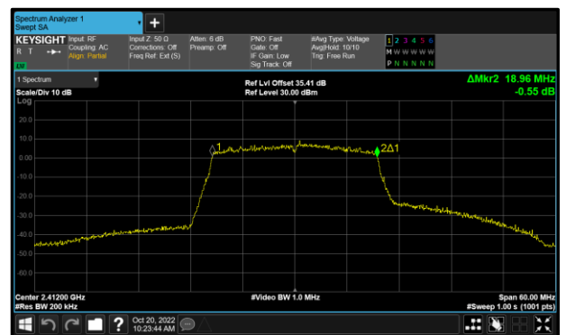
Figure 46 - 802.11ax HE20 SU Maximum 99% OBW
