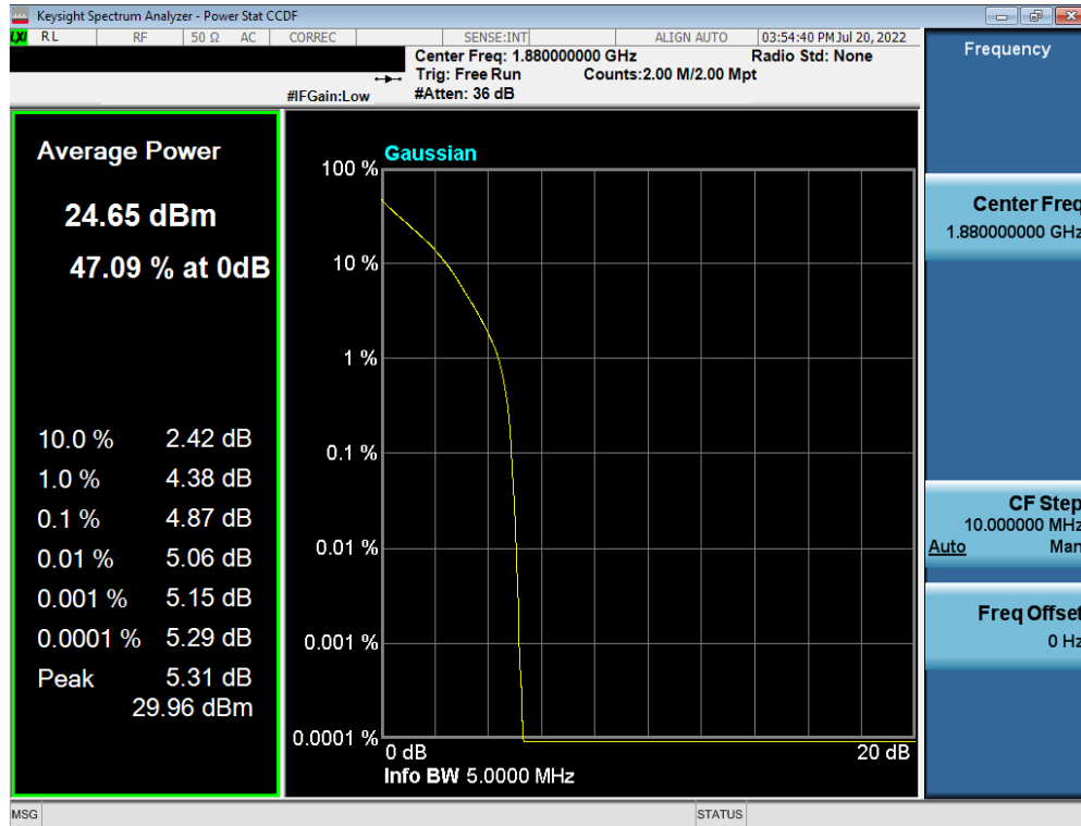
Plot 7-216. PAR Plot (LTE Band 2 - 5MHz QPSK - Full RB Configuration)
