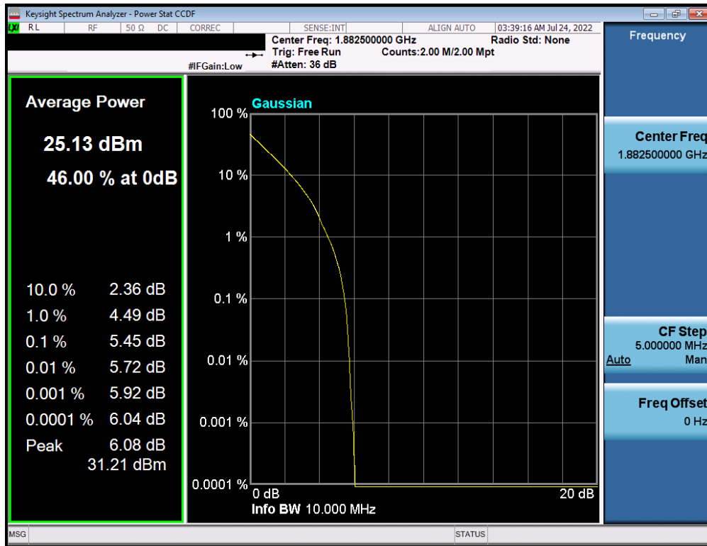
Plot 7-238. PAR Plot (NR Band n25 - 10.0MHz DFT-s-OFDM QPSK - Full RB)
