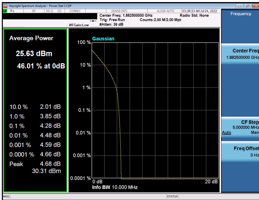
Plot 7-237. PAR Plot (NR Band n25 - 10.0MHz DFT-s-OFDM \pi/2 BPSK - Full RB)
