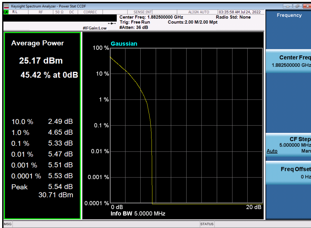
Plot 7-233. PAR Plot (NR Band n25 - 5.0MHz DFT-s-OFDM QPSK - Full RB)
