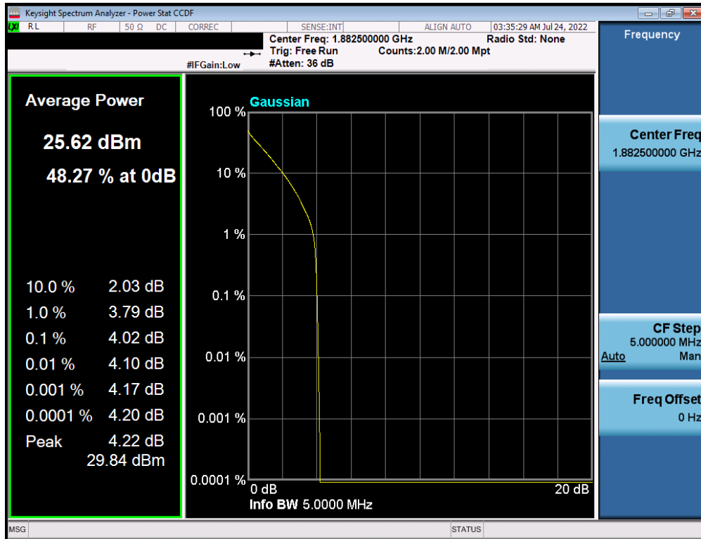
Plot 7-232. PAR Plot (NR Band n25 - 5.0MHz DFT-s-OFDM \pi/2 BPSK - Full RB)
