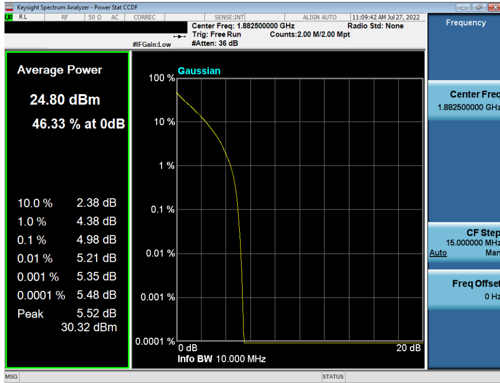
Plot 7-196. PAR Plot (LTE Band 25 - 10MHz QPSK - Full RB Configuration)
