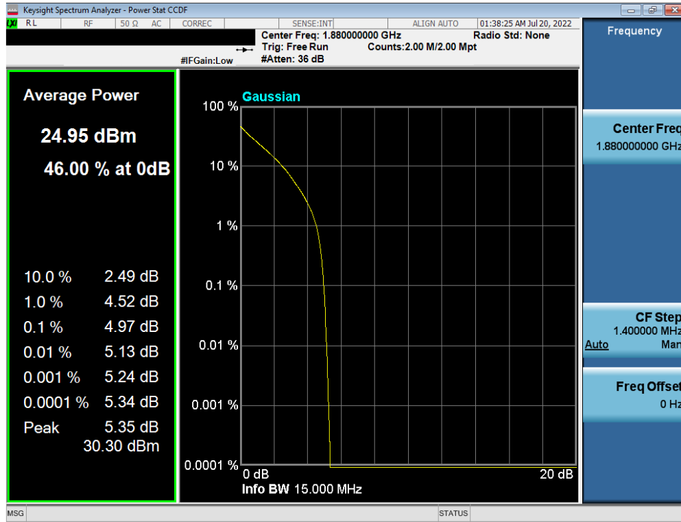
Plot 7-224. PAR Plot (LTE Band 2 - 15MHz QPSK - Full RB Configuration)
