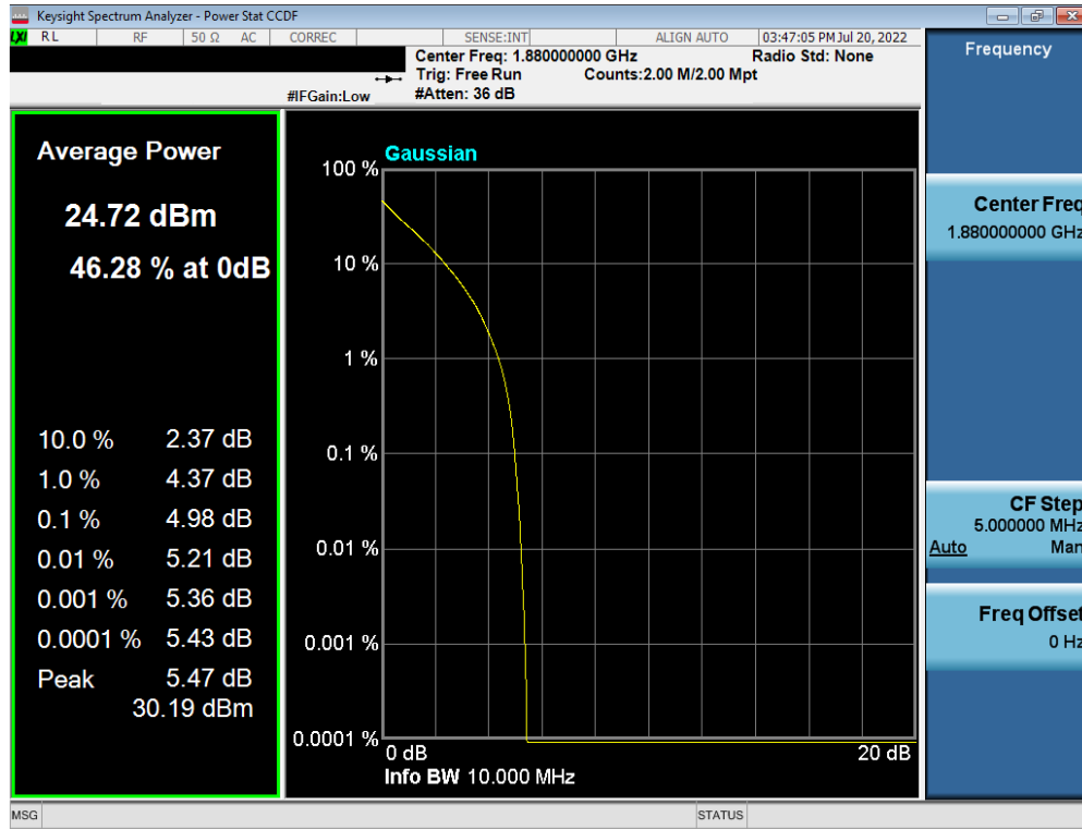
Plot 7-220. PAR Plot (LTE Band 2 - 10MHz QPSK - Full RB Configuration)
