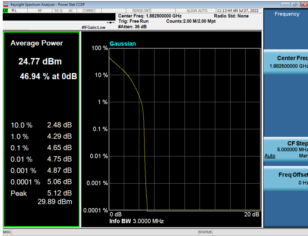
Plot 7-188. PAR Plot (LTE Band 25 - 3MHz QPSK - Full RB Configuration)
