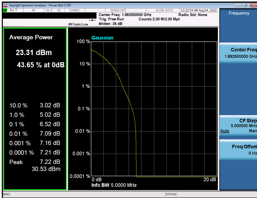
Plot 7-235. PAR Plot (NR Band n25 - 5.0MHz DFT-s-OFDM 64-QAM - Full RB)
