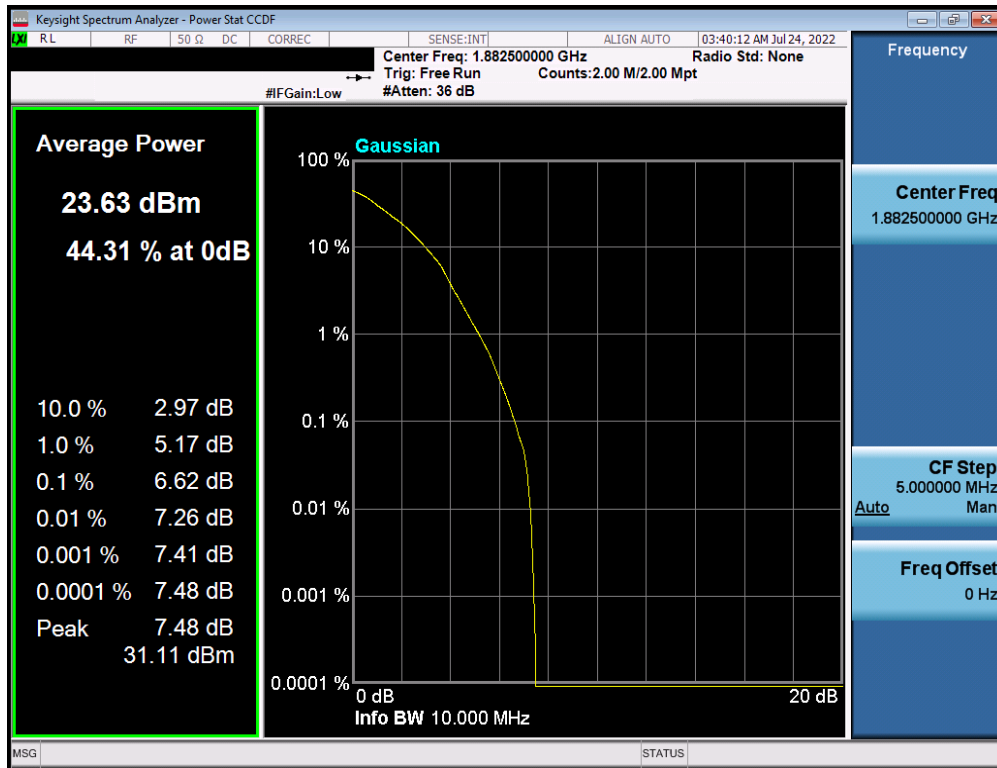
Plot 7-240. PAR Plot (NR Band n25 - 10.0MHz DFT-s-OFDM 64-QAM - Full RB)
