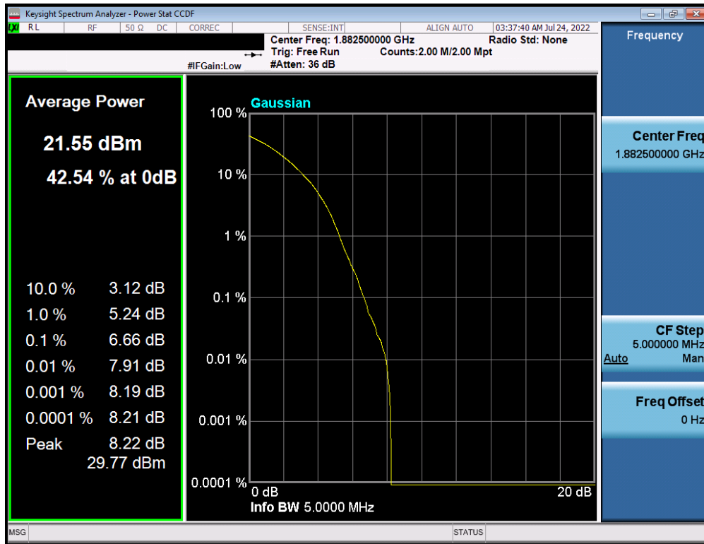
Plot 7-236. PAR Plot (NR Band n25 - 5.0MHz DFT-s-OFDM 256-QAM - Full RB)
