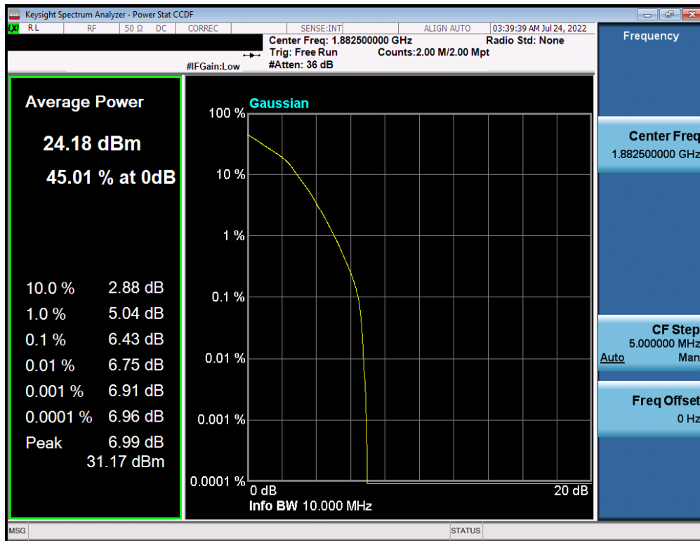
Plot 7-239. PAR Plot (NR Band n25 - 10.0MHz DFT-s-OFDM 16-QAM - Full RB)
