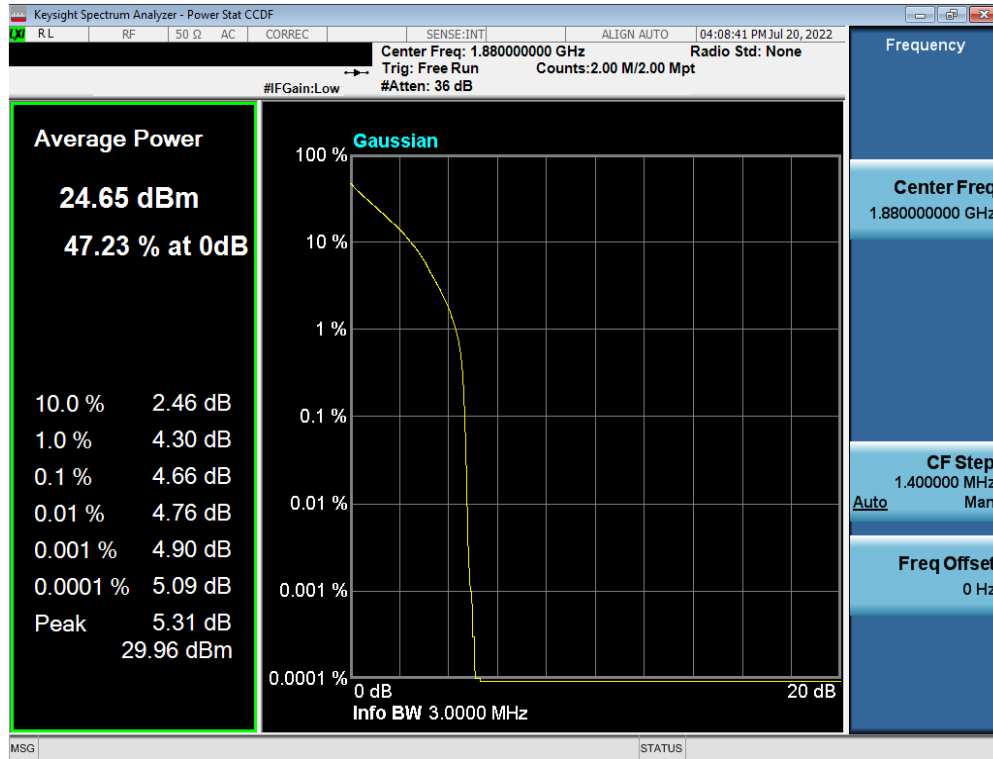
Plot 7-212. PAR Plot (LTE Band 2 - 3MHz QPSK - Full RB Configuration)
