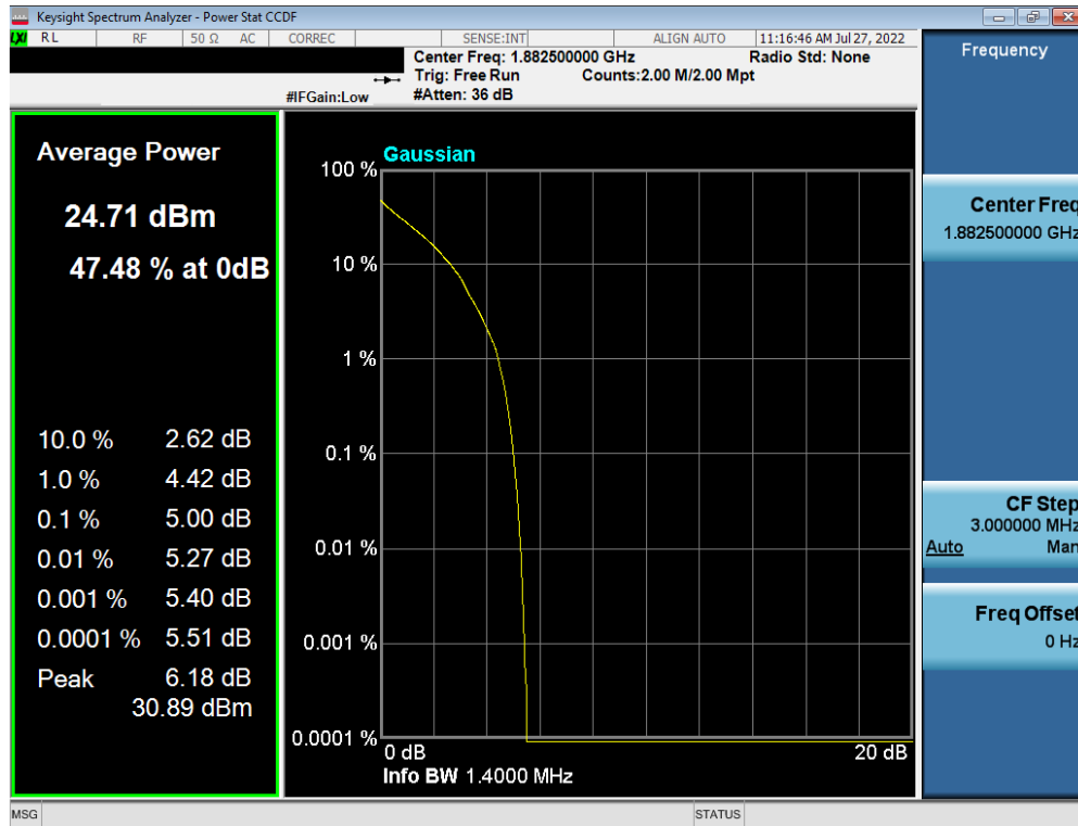
Plot 7-184. PAR Plot (LTE Band 25 - 1.4MHz QPSK - Full RB Configuration)
