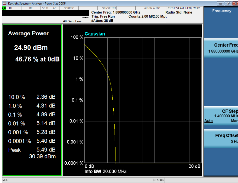
Plot 7-228. PAR Plot (LTE Band 2 - 20MHz QPSK - Full RB Configuration)
