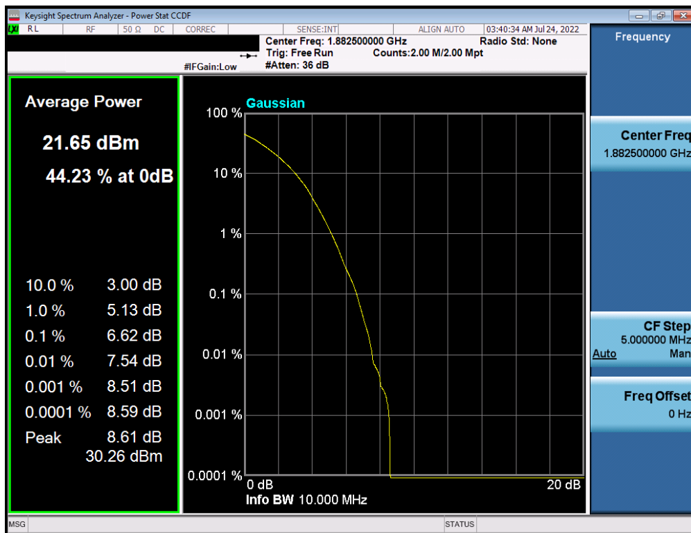
Plot 7-241. PAR Plot (NR Band n25 - 10.0MHz DFT-s-OFDM 256-QAM - Full RB)
