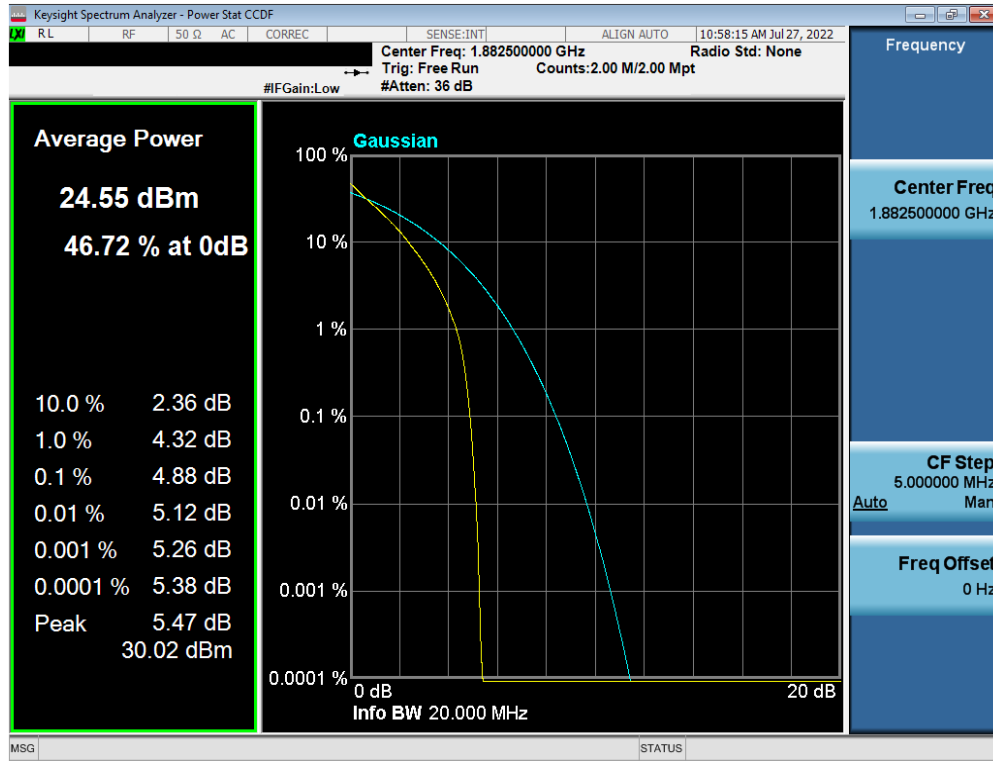
Plot 7-204. PAR Plot (LTE Band 25 - 20MHz QPSK - Full RB Configuration)
