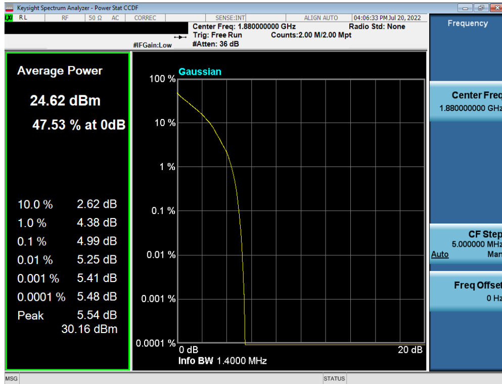
Plot 7-208. PAR Plot (LTE Band 2 - 1.4MHz QPSK - Full RB Configuration)
