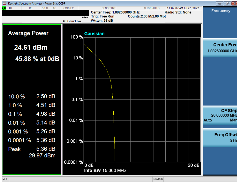
Plot 7-200. PAR Plot (LTE Band 25 - 15MHz QPSK - Full RB Configuration)
