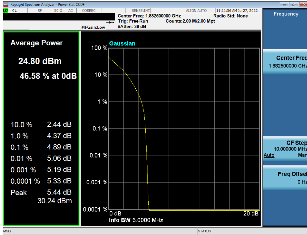
Plot 7-192. PAR Plot (LTE Band 25 - 5MHz QPSK - Full RB Configuration)
