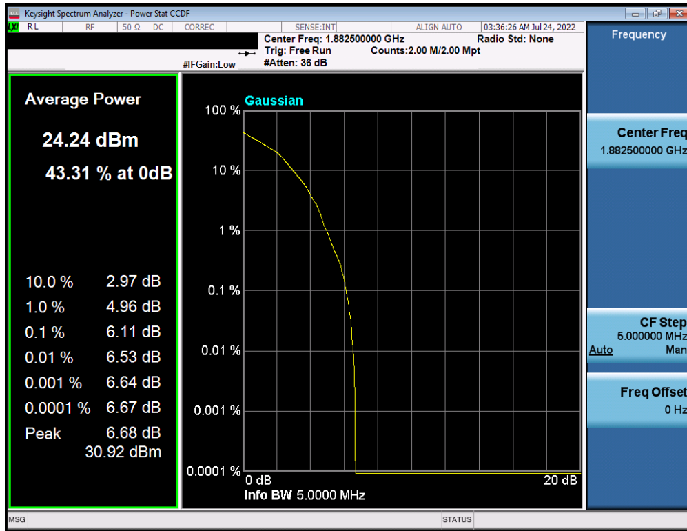
Plot 7-234. PAR Plot (NR Band n25 - 5.0MHz DFT-s-OFDM 16-QAM - Full RB)
