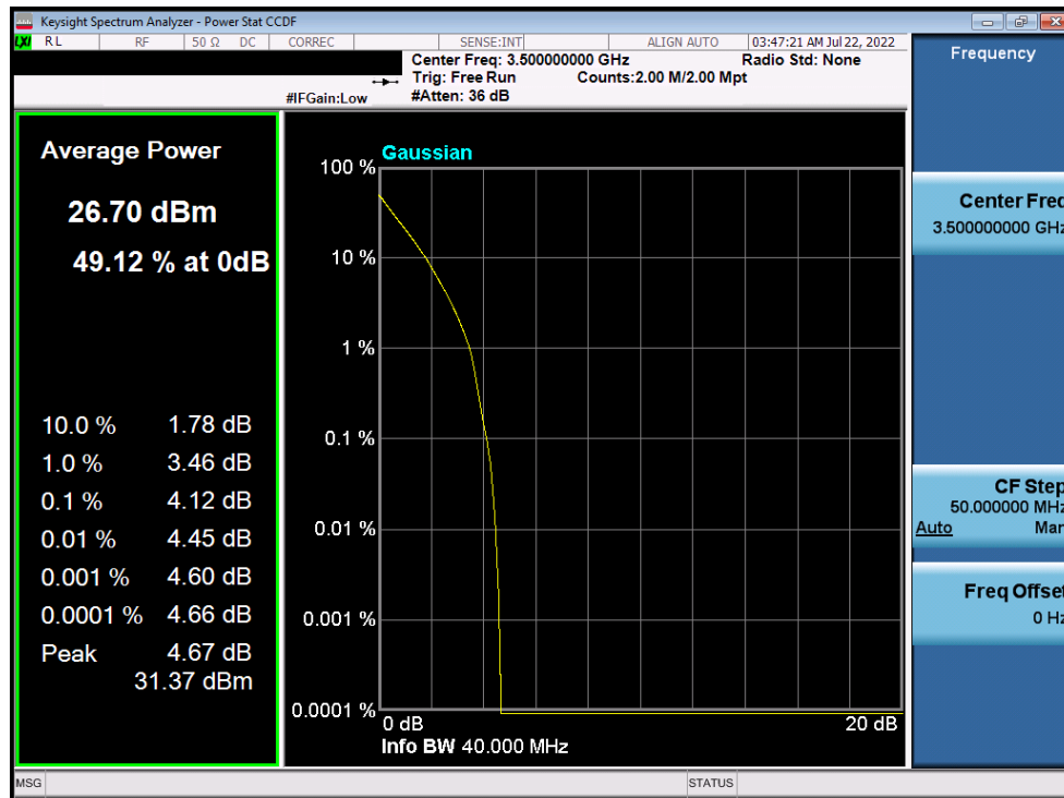
Plot 7-155. PAR Plot (NR Band n77 - 40MHz DFT-s-OFDM \pi/2 BPSK - Full RB)
