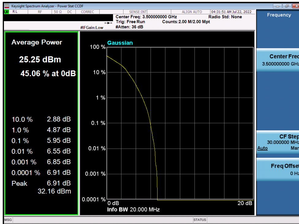
Plot 7-147. PAR Plot (NR Band n77 - 20MHz DFT-s-OFDM 16-QAM - Full RB)
