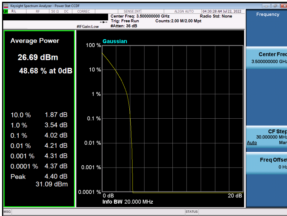
Plot 7-145. PAR Plot (NR Band n77 - 20MHz DFT-s-OFDM \pi/2 BPSK - Full RB)
