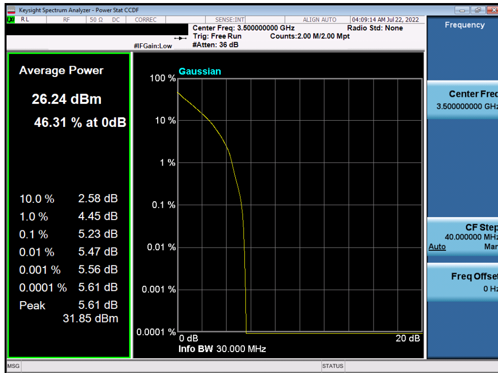
Plot 7-151. PAR Plot (NR Band n77 - 30MHz DFT-s-OFDM QPSK - Full RB)
