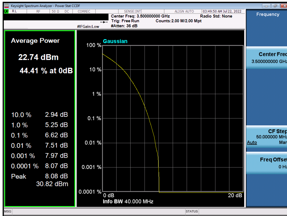
Plot 7-159. PAR Plot (NR Band n77 - 40MHz DFT-s-OFDM 256-QAM - Full RB)
