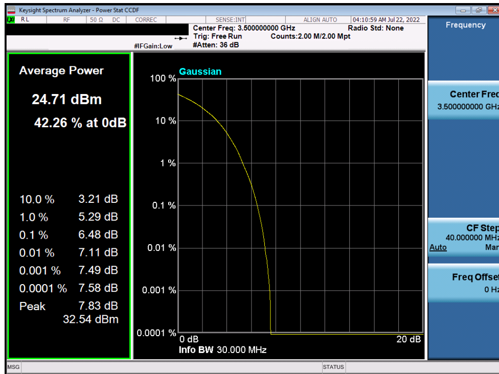
Plot 7-153. PAR Plot (NR Band n77 - 30MHz DFT-s-OFDM 64-QAM - Full RB)
