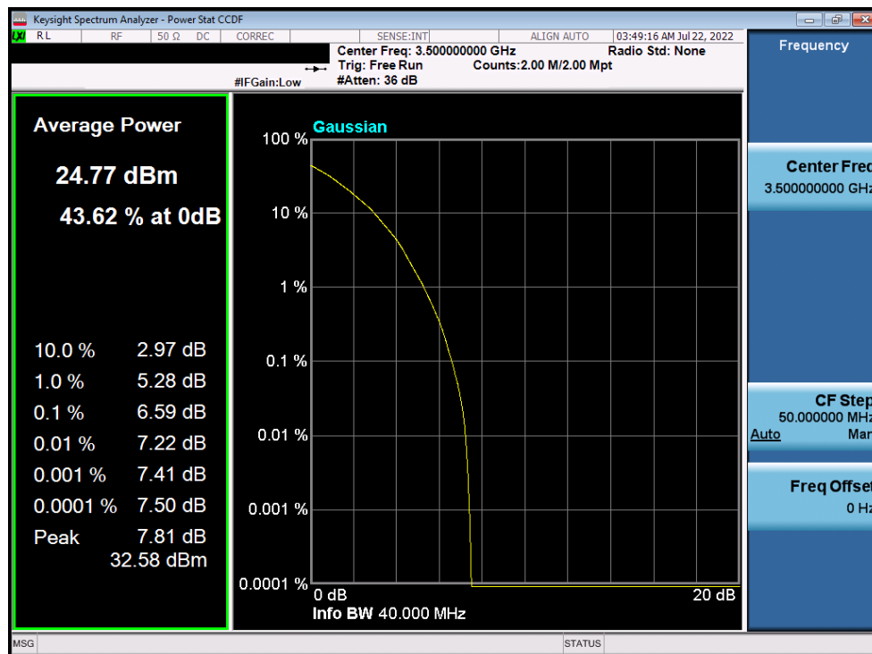
Plot 7-158. PAR Plot (NR Band n77 - 40MHz DFT-s-OFDM 64-QAM - Full RB)
