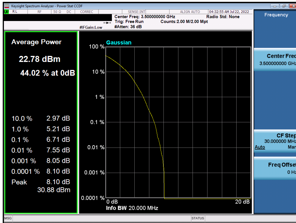
Plot 7-149. PAR Plot (NR Band n77 - 20MHz DFT-s-OFDM 256-QAM - Full RB)
