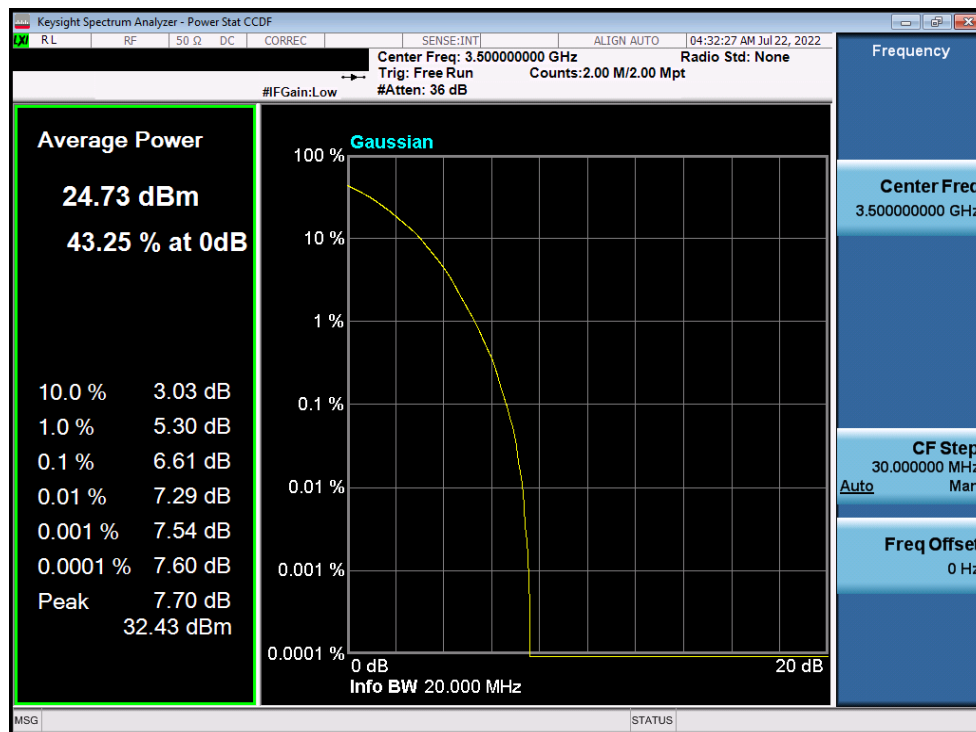
Plot 7-148. PAR Plot (NR Band n77 - 20MHz DFT-s-OFDM 64-QAM - Full RB)
