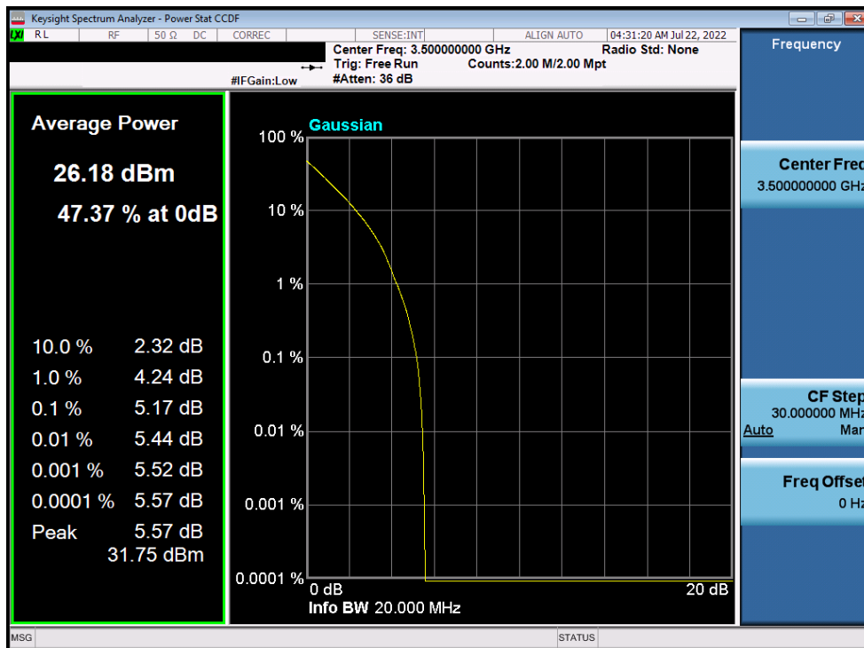
Plot 7-146. PAR Plot (NR Band n77 - 20MHz DFT-s-OFDM QPSK - Full RB)
