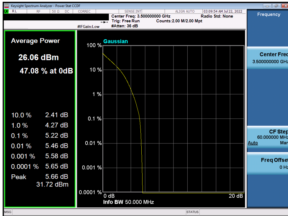
Plot 7-161. PAR Plot (NR Band n77 - 50MHz DFT-s-OFDM QPSK - Full RB)
