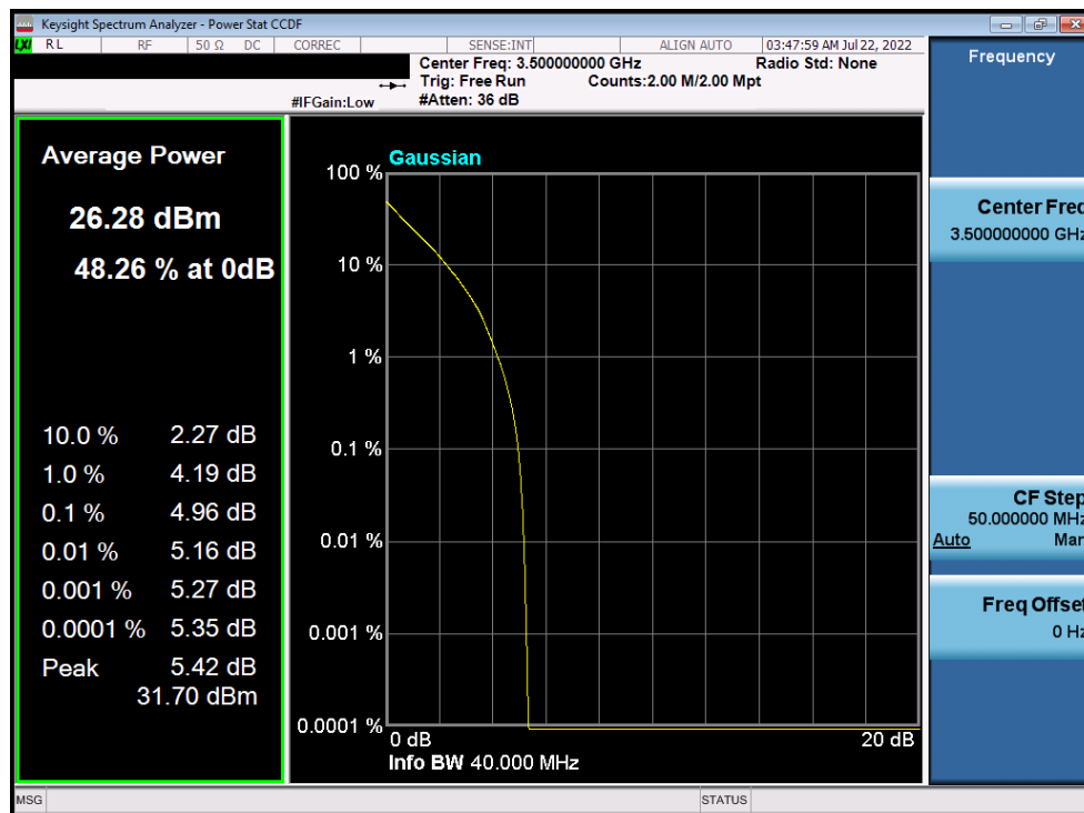
Plot 7-156. PAR Plot (NR Band n77 - 40MHz DFT-s-OFDM QPSK - Full RB)
