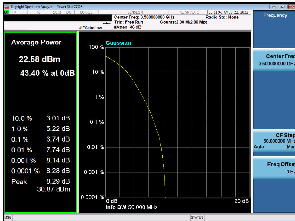
Plot 7-164. PAR Plot (NR Band n77 - 50MHz DFT-s-OFDM 256-QAM - Full RB)
