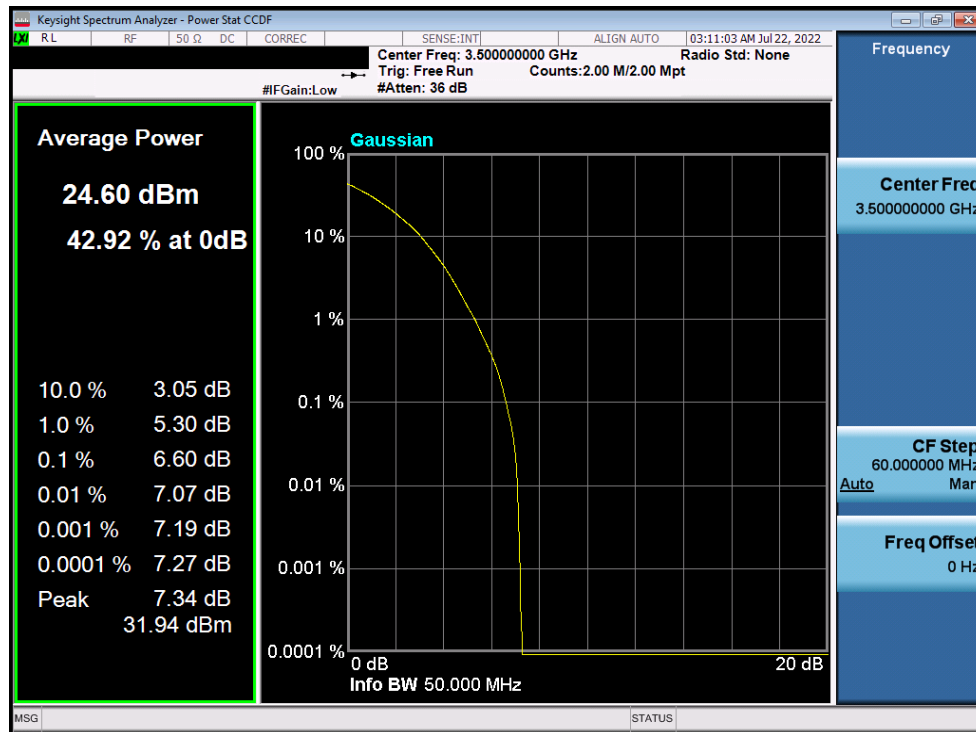
Plot 7-163. PAR Plot (NR Band n77 - 50MHz DFT-s-OFDM 64-QAM - Full RB)
