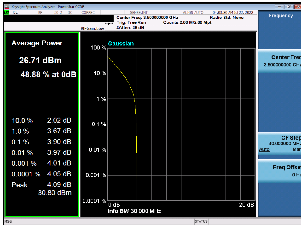
Plot 7-150. PAR Plot (NR Band n77 - 30MHz DFT-s-OFDM \pi/2 BPSK - Full RB)
