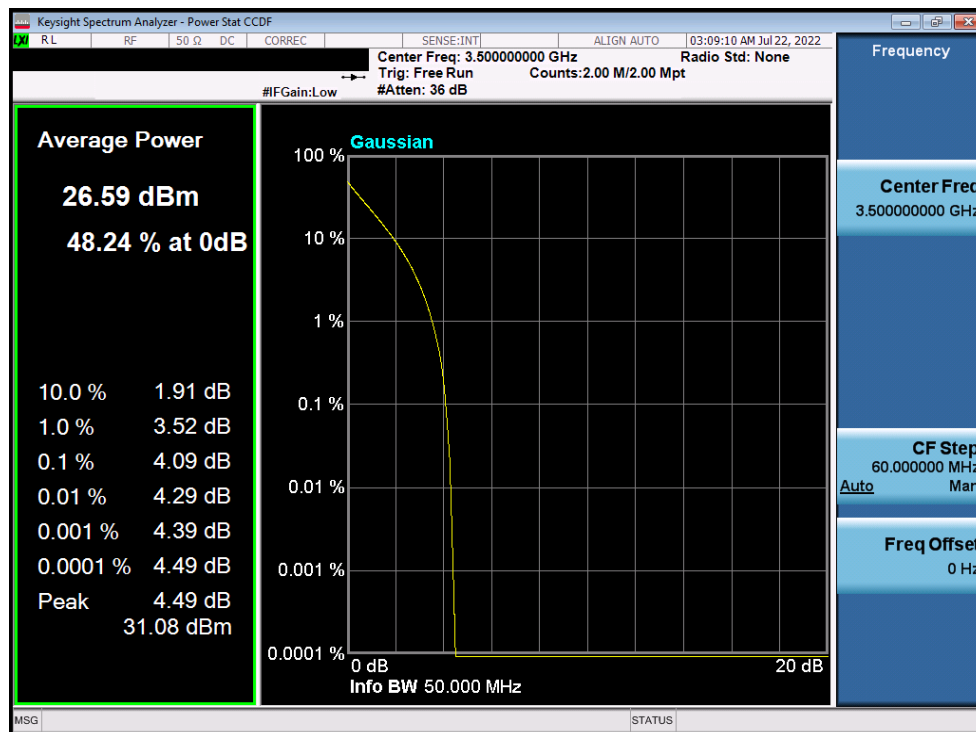
Plot 7-160. PAR Plot (NR Band n77 - 50MHz DFT-s-OFDM \pi/2 BPSK - Full RB)
