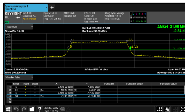
Figure 156 - 802.11ax HE20 SU Maximum 99% OBW
