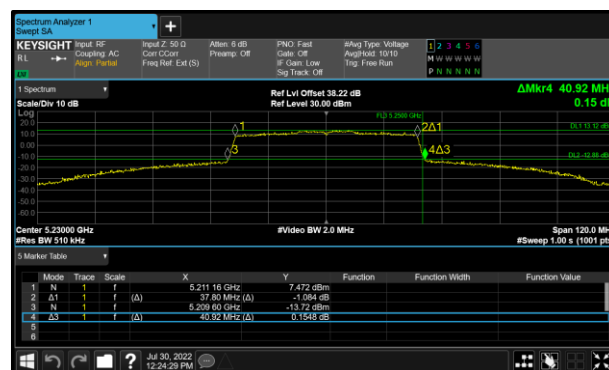
Figure 158 - 802.11ax HE40 SU Maximum 99% OBW
