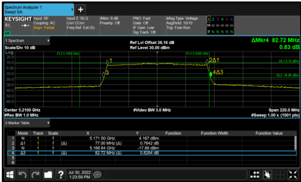
Figure 111 - 802.11ax HE80 SU Minimum 99% OBW
