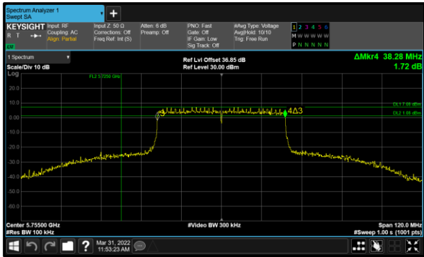
Figure 121 - 802.11ax HE40 SU Minimum 6 dB EBW
