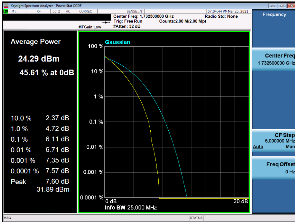
Plot 7-199. PAR Plot (LTE Band 4 - 15MHz QPSK - Full RB Configuration)
