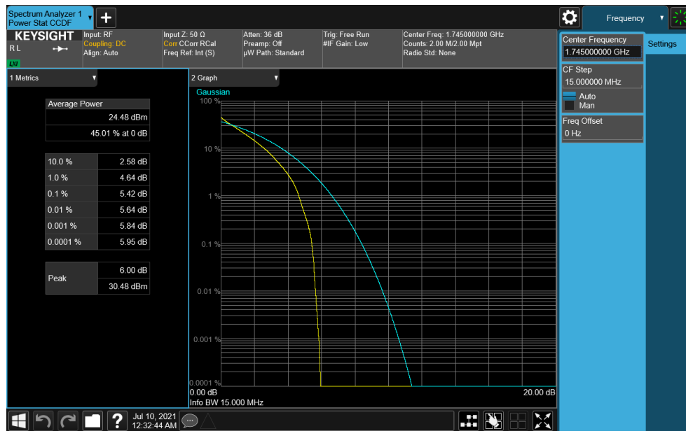
Plot 7-387. PAR Plot (NR Band n66- 15MHz DFT-s-OFDM QPSK - Full RB)
