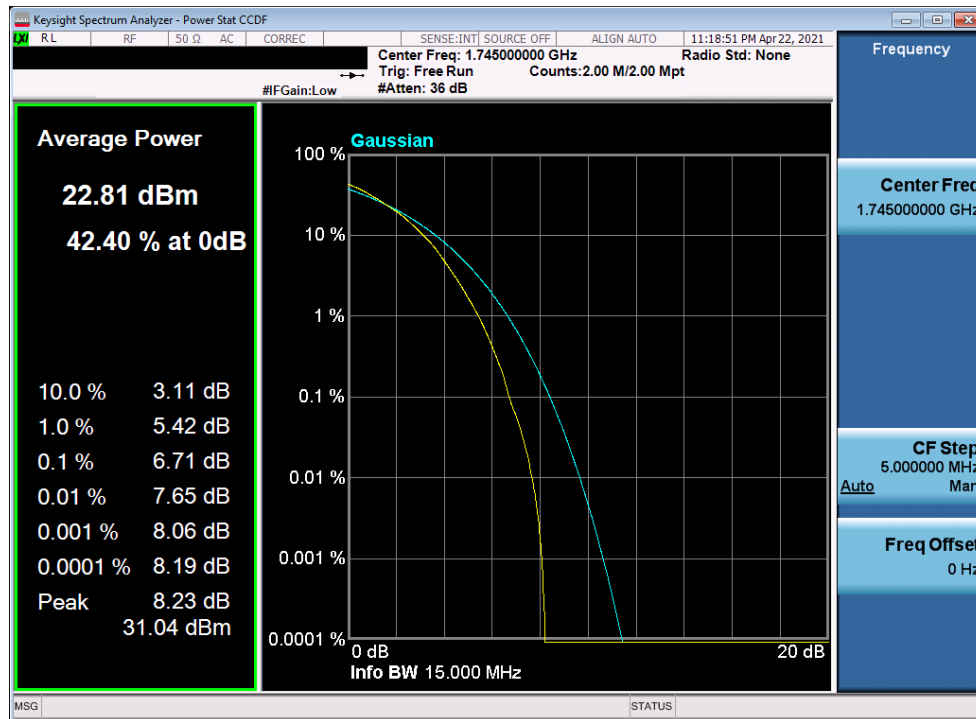
Plot 7-346. PAR Plot (LTE Band 66 - 15MHz 64-QAM - Full RB)
