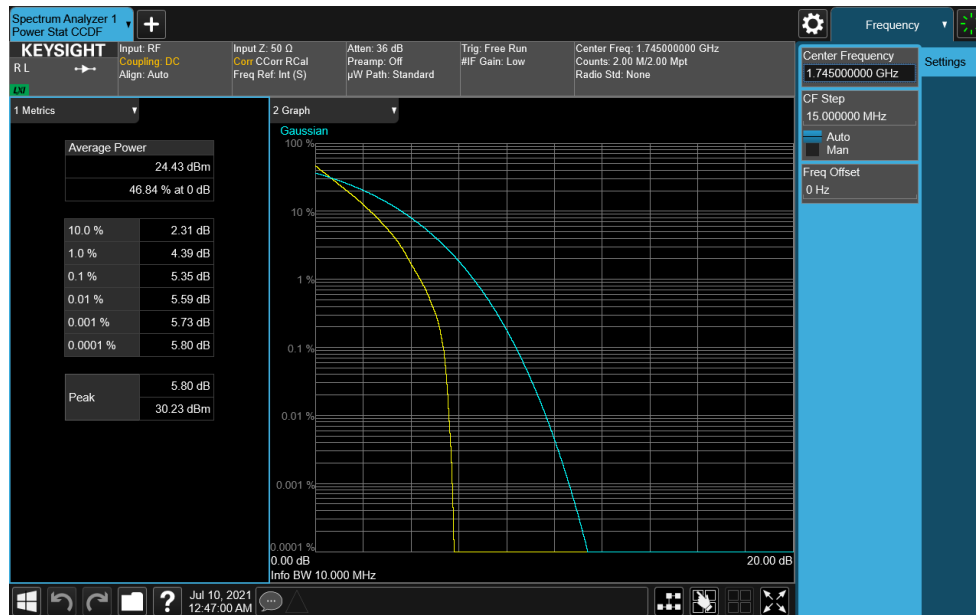
Plot 7-382. PAR Plot (NR Band n66- 10MHz DFT-s-OFDM QPSK - Full RB)
