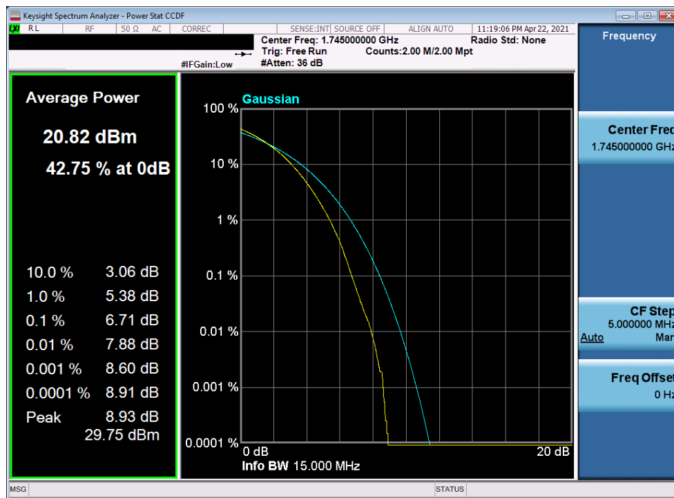
Plot 7-347. PAR Plot (LTE Band 66 - 15MHz 256-QAM - Full RB)
