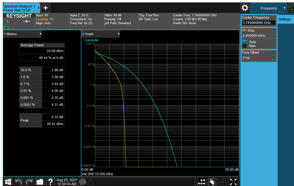
Plot 7-381. PAR Plot (NR Band n66- 10MHz DFT-s-OFDM \pi/2 BPSK - Full RB)
