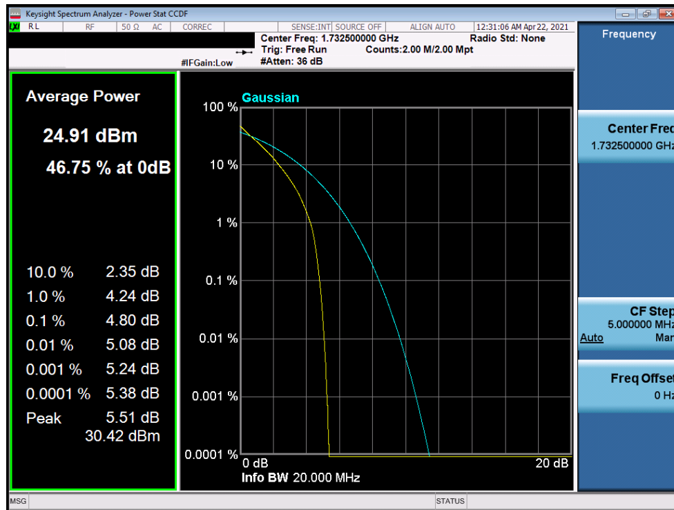
Plot 7-372. PAR Plot (LTE Band 4 - 20MHz QPSK - Full RB)
