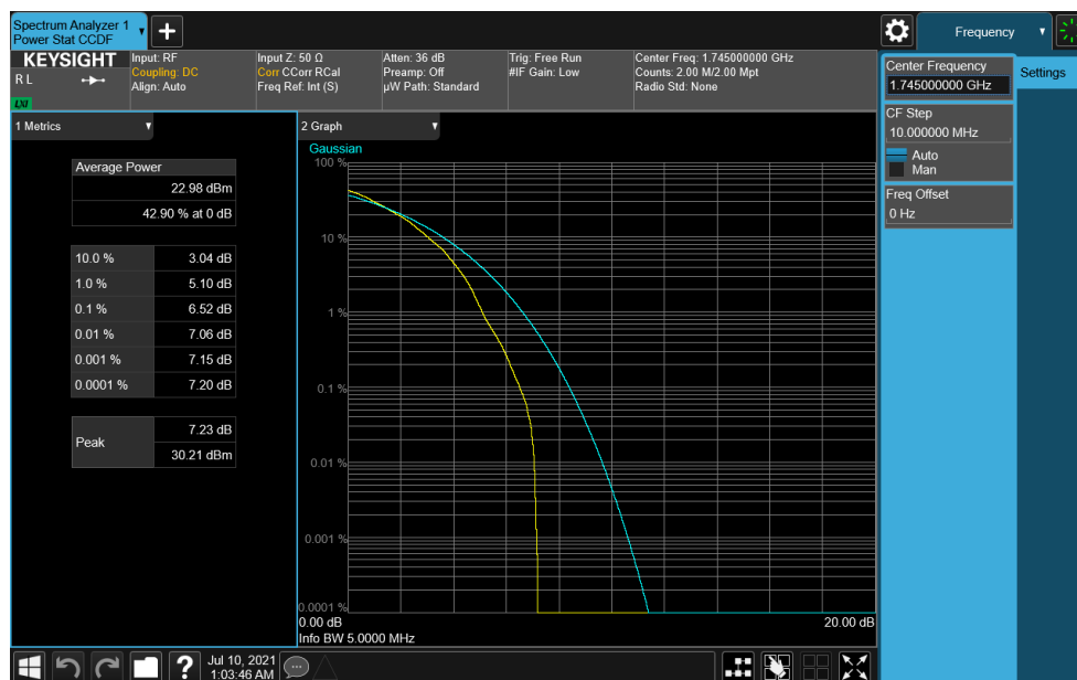
Plot 7-379. PAR Plot (NR Band n66- 5MHz DFT-s-OFDM 64-QAM - Full RB)
