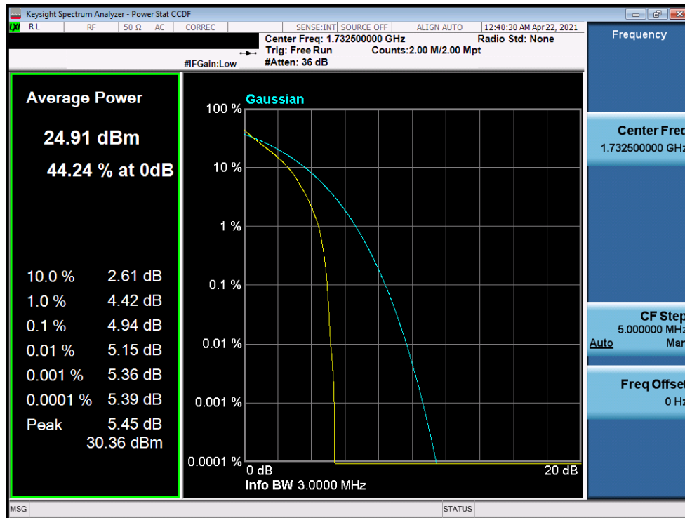
Plot 7-356. PAR Plot (LTE Band 4 - 3MHz QPSK - Full RB)
