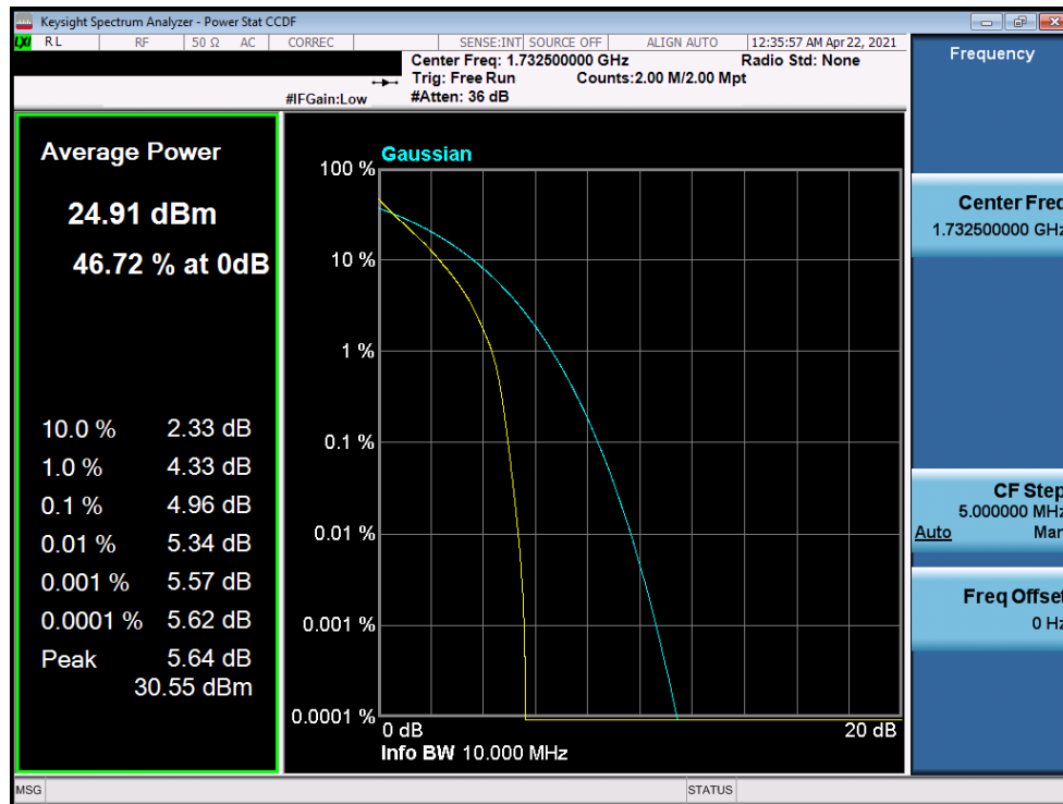
Plot 7-364. PAR Plot (LTE Band 4 - 10MHz QPSK - Full RB)
