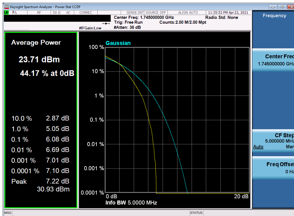
Plot 7-337. PAR Plot (LTE Band 66 - 5MHz 16-QAM - Full RB)
