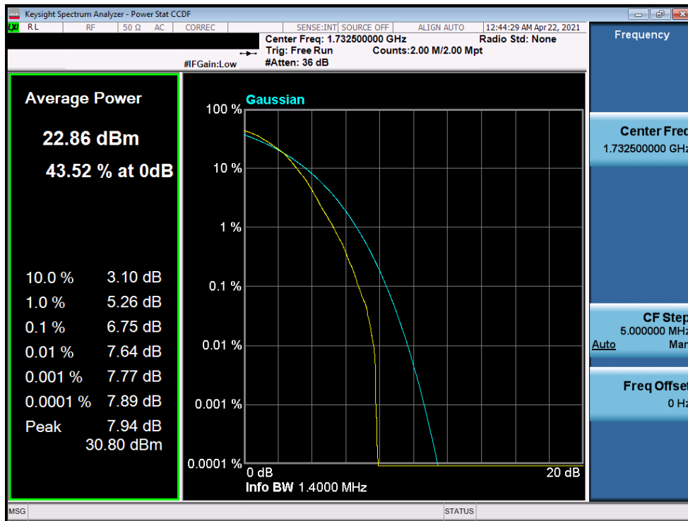
Plot 7-354. PAR Plot (LTE Band 4 - 1.4MHz 64-QAM - Full RB)
