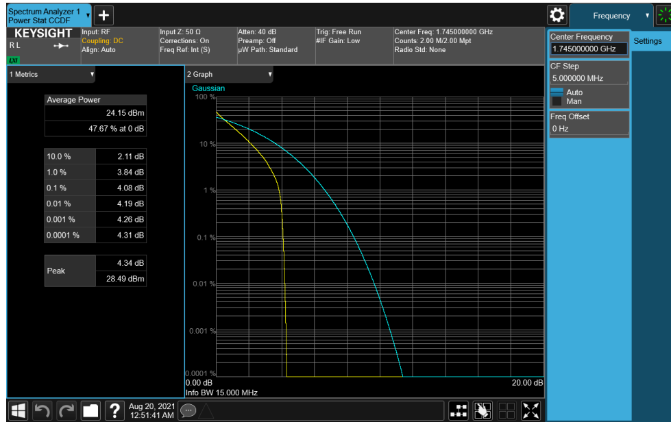
Plot 7-386. PAR Plot (NR Band n66- 15MHz DFT-s-OFDM \pi/2 BPSK - Full RB)
