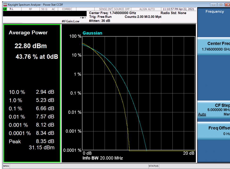
Plot 7-350. PAR Plot (LTE Band 66 - 20MHz 64-QAM - Full RB)
