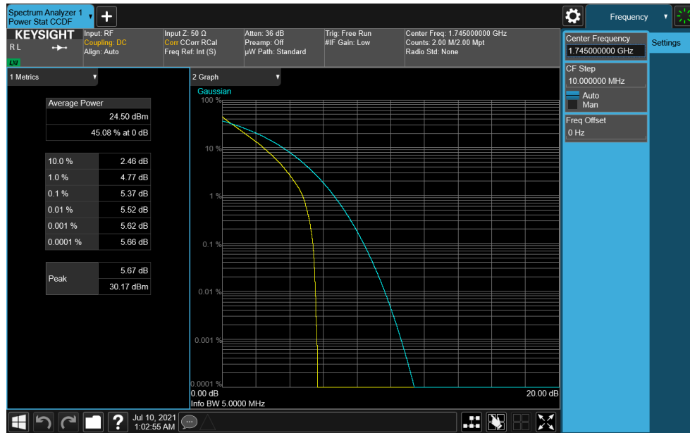
Plot 7-377. PAR Plot (NR Band n66- 5MHz DFT-s-OFDM QPSK - Full RB)
