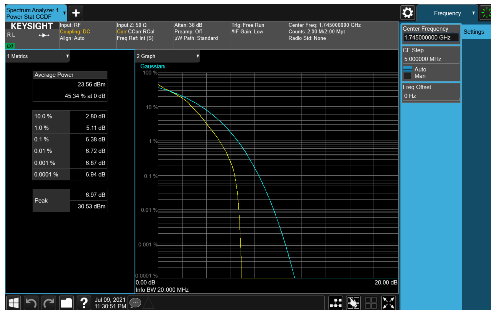
Plot 7-393. PAR Plot (NR Band n66- 20MHz DFT-s-OFDM 16-QAM - Full RB)
