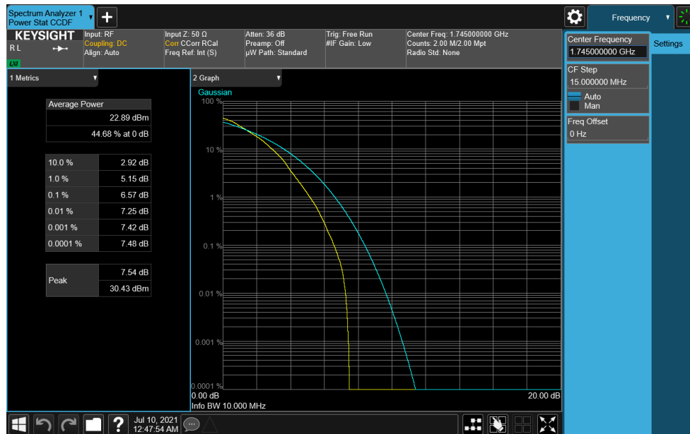
Plot 7-384. PAR Plot (NR Band n66- 10MHz DFT-s-OFDM 64-QAM - Full RB)
