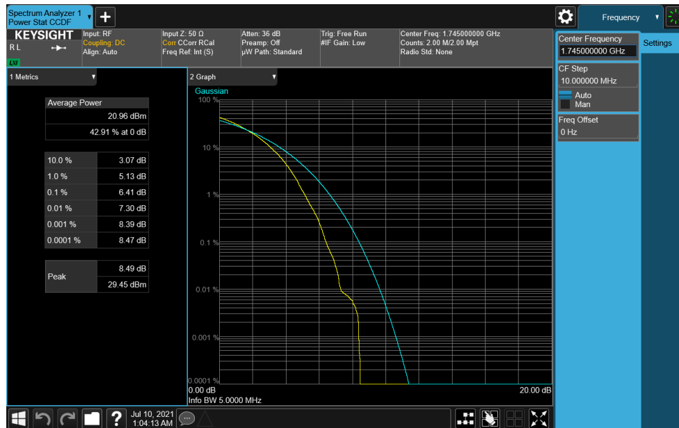
Plot 7-380. PAR Plot (NR Band n66- 5MHz DFT-s-OFDM 256-QAM - Full RB)
