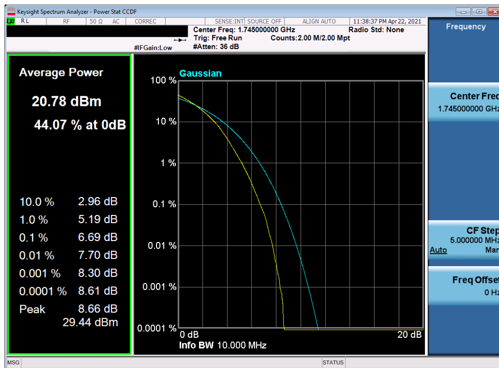
Plot 7-343. PAR Plot (LTE Band 66 - 10MHz 256-QAM - Full RB)
