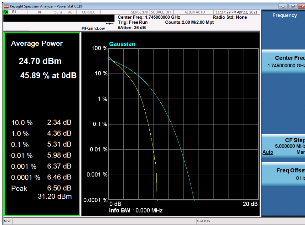
Plot 7-340. PAR Plot (LTE Band 66 - 10MHz QPSK - Full RB)
