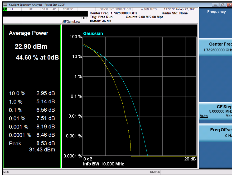
Plot 7-366. PAR Plot (LTE Band 4 - 10MHz 64-QAM - Full RB)
