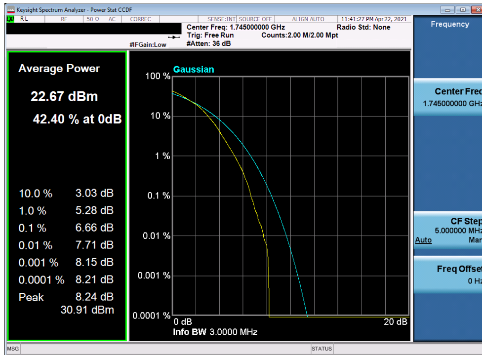
Plot 7-334. PAR Plot (LTE Band 66 - 3MHz 64-QAM - Full RB)
