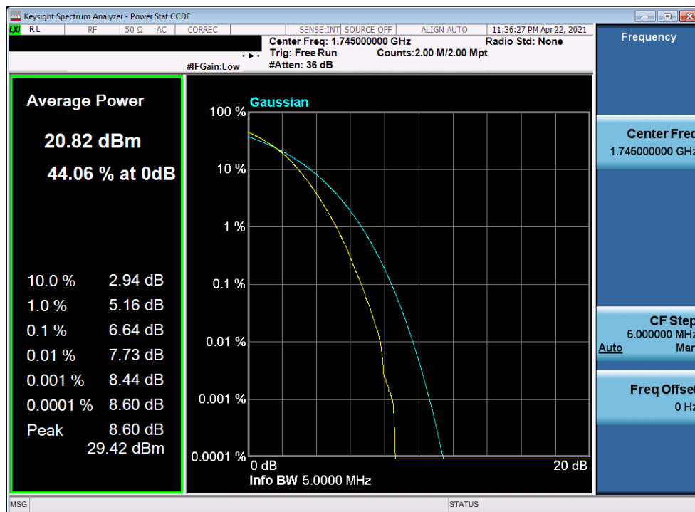
Plot 7-339. PAR Plot (LTE Band 66 - 5MHz 256-QAM - Full RB)
