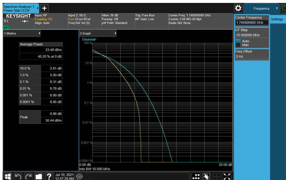
Plot 7-383. PAR Plot (NR Band n66- 10MHz DFT-s-OFDM 16-QAM - Full RB)
