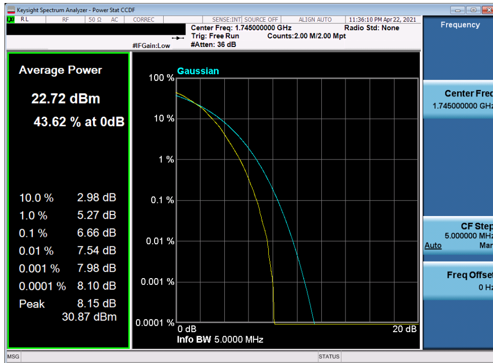
Plot 7-338. PAR Plot (LTE Band 66 - 5MHz 64-QAM - Full RB)
