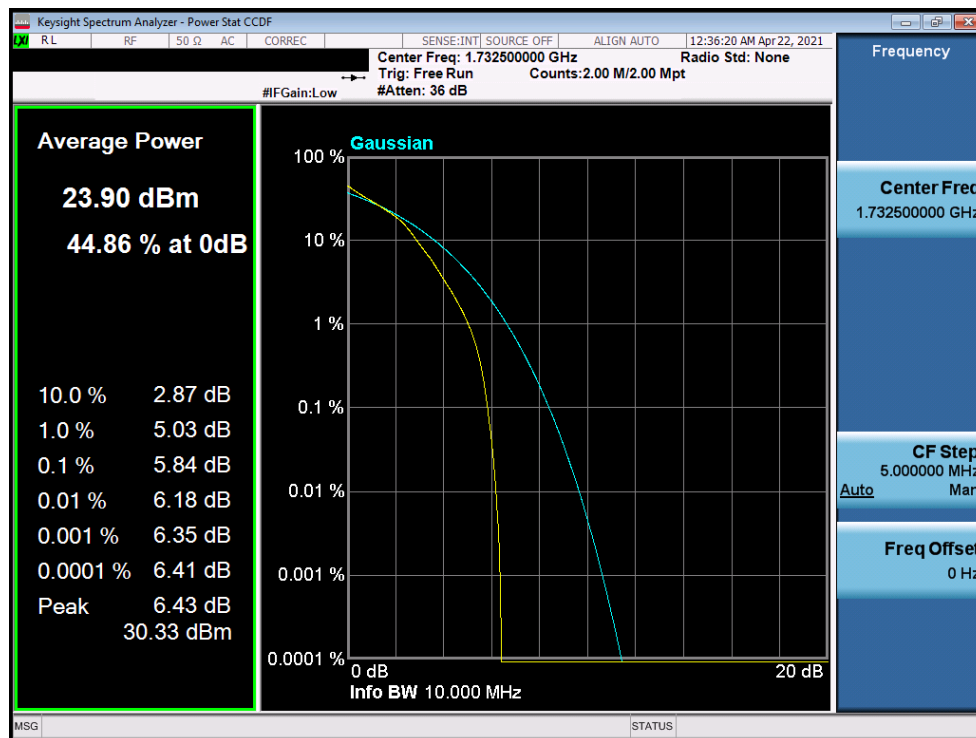
Plot 7-365. PAR Plot (LTE Band 4 - 10MHz 16-QAM - Full RB)
