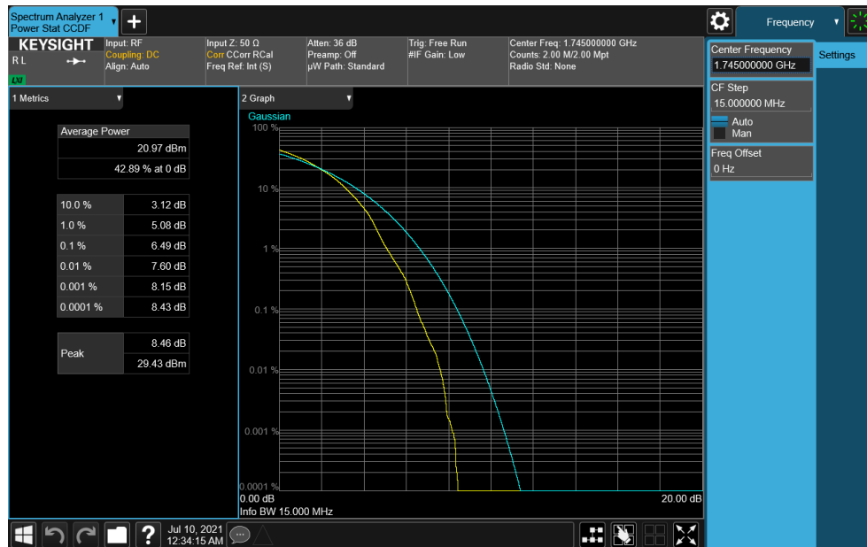
Plot 7-390. PAR Plot (NR Band n66- 15MHz DFT-s-OFDM 256-QAM - Full RB)
