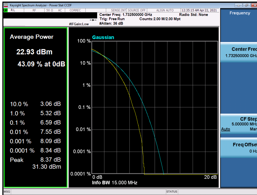
Plot 7-370. PAR Plot (LTE Band 4 - 15MHz 64-QAM - Full RB)
