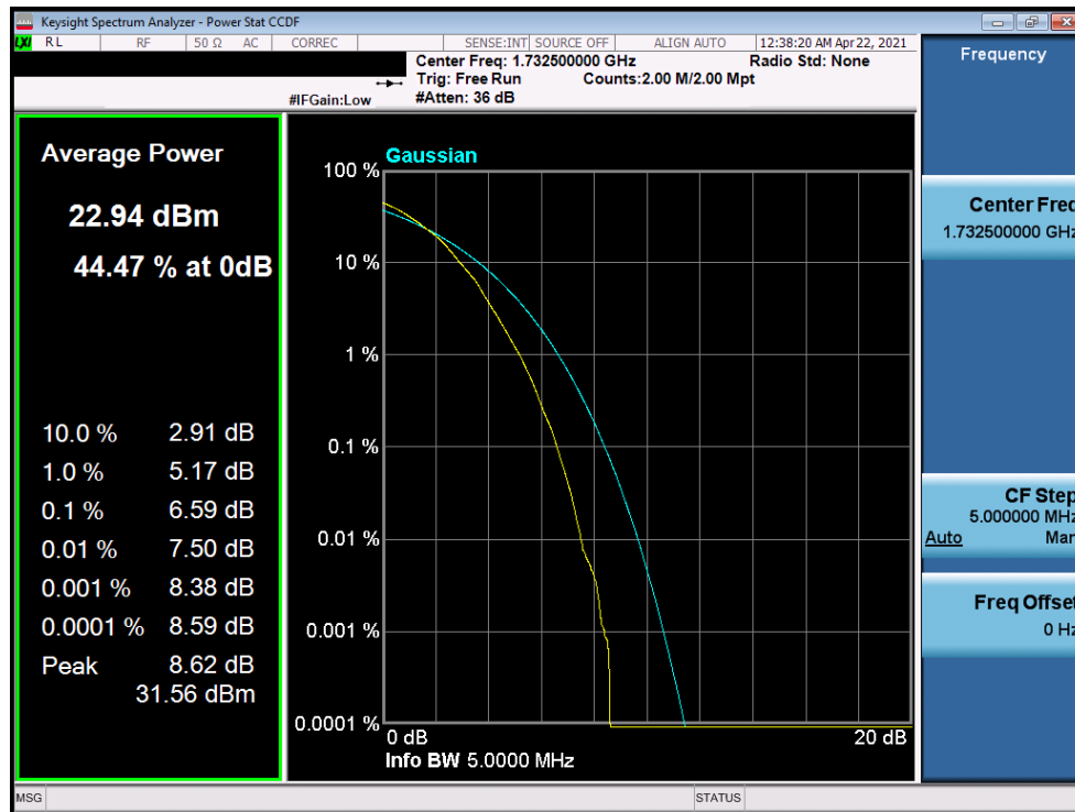
Plot 7-362. PAR Plot (LTE Band 4 - 5MHz 64-QAM - Full RB)
