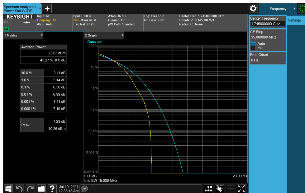
Plot 7-389. PAR Plot (NR Band n66- 15MHz DFT-s-OFDM 64-QAM - Full RB)
