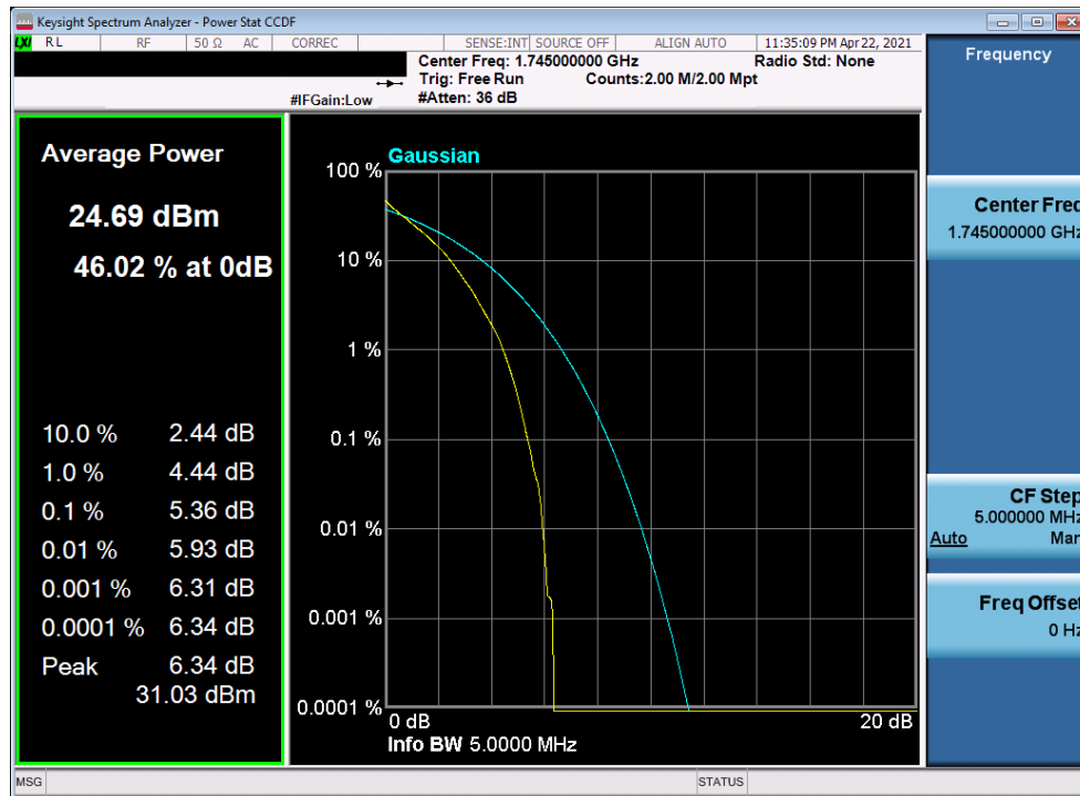
Plot 7-336. PAR Plot (LTE Band 66 - 5MHz QPSK - Full RB)
