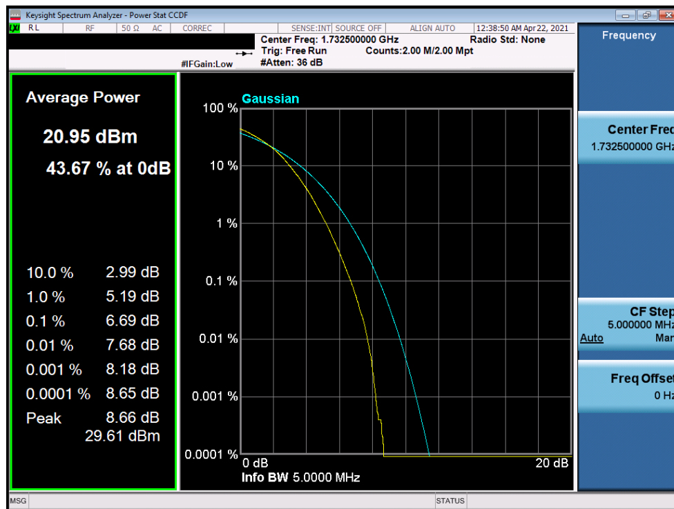
Plot 7-363. PAR Plot (LTE Band 4 - 5MHz 256-QAM - Full RB)
