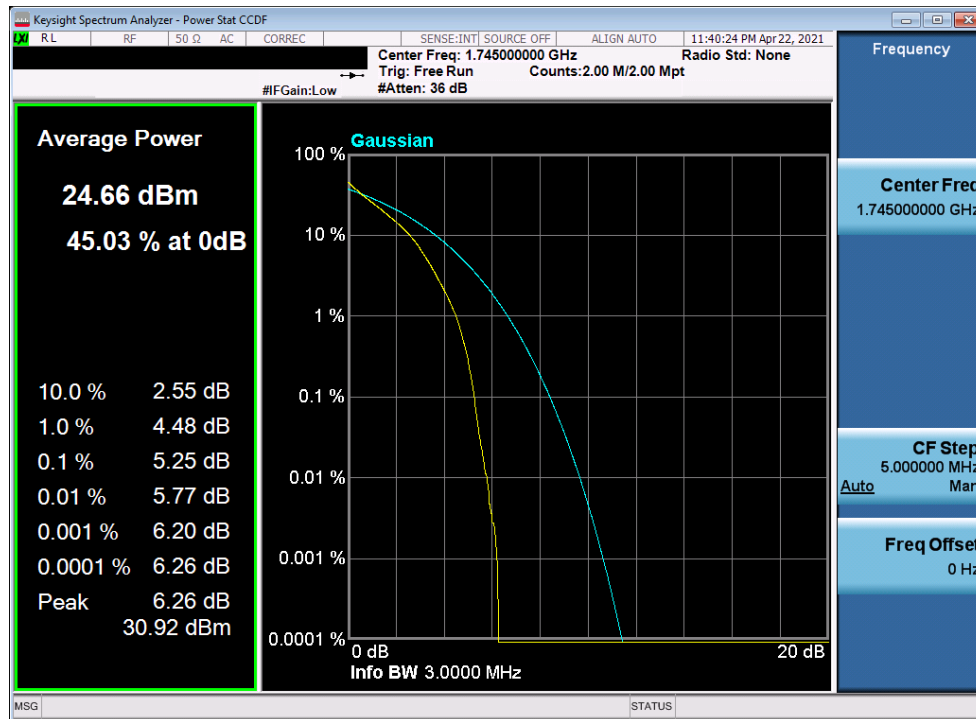
Plot 7-332. PAR Plot (LTE Band 66 - 3MHz QPSK - Full RB)
