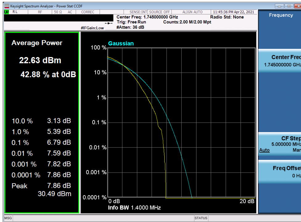
Plot 7-330. PAR Plot (LTE Band 66 - 1.4MHz 64-QAM - Full RB)
