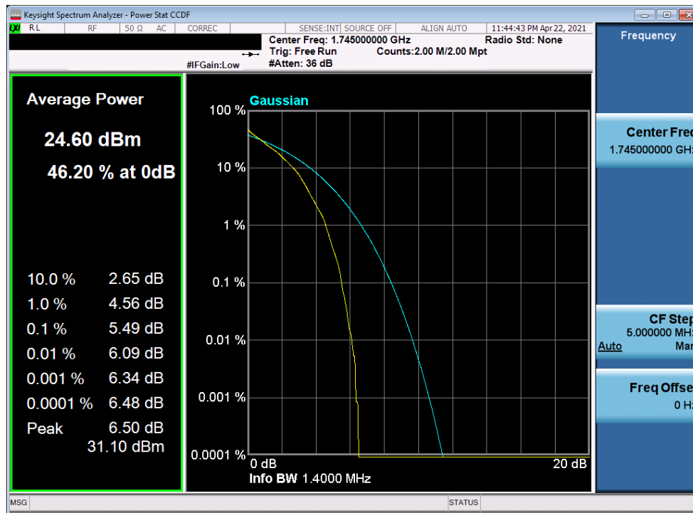
Plot 7-328. PAR Plot (LTE Band 66 - 1.4MHz QPSK - Full RB)
