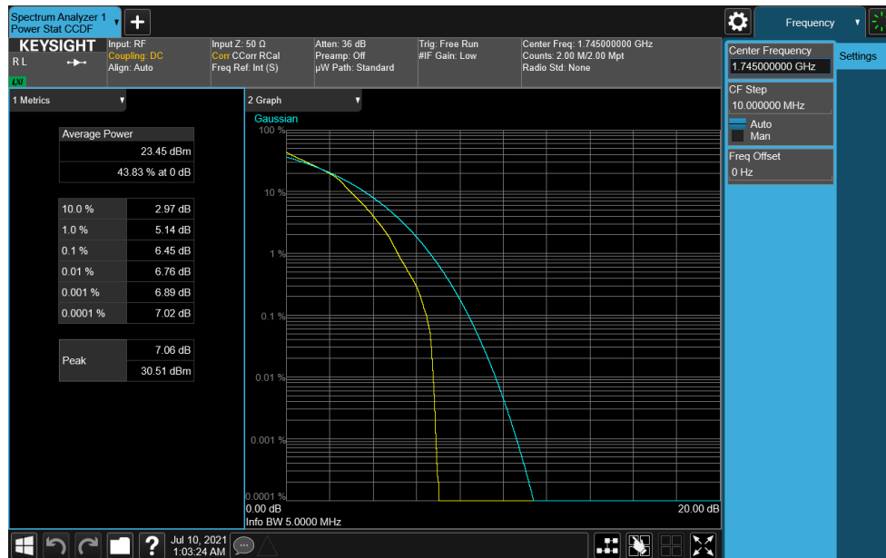
Plot 7-378. PAR Plot (NR Band n66- 5MHz DFT-s-OFDM 16-QAM - Full RB)
