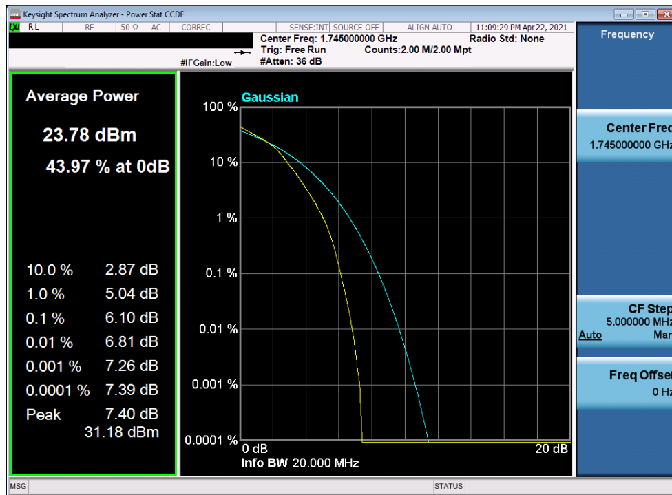
Plot 7-349. PAR Plot (LTE Band 66 - 20MHz 16-QAM - Full RB)
