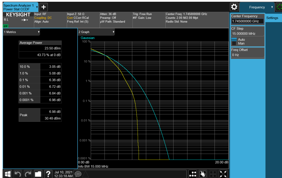
Plot 7-388. PAR Plot (NR Band n66- 15MHz DFT-s-OFDM 16-QAM - Full RB)
