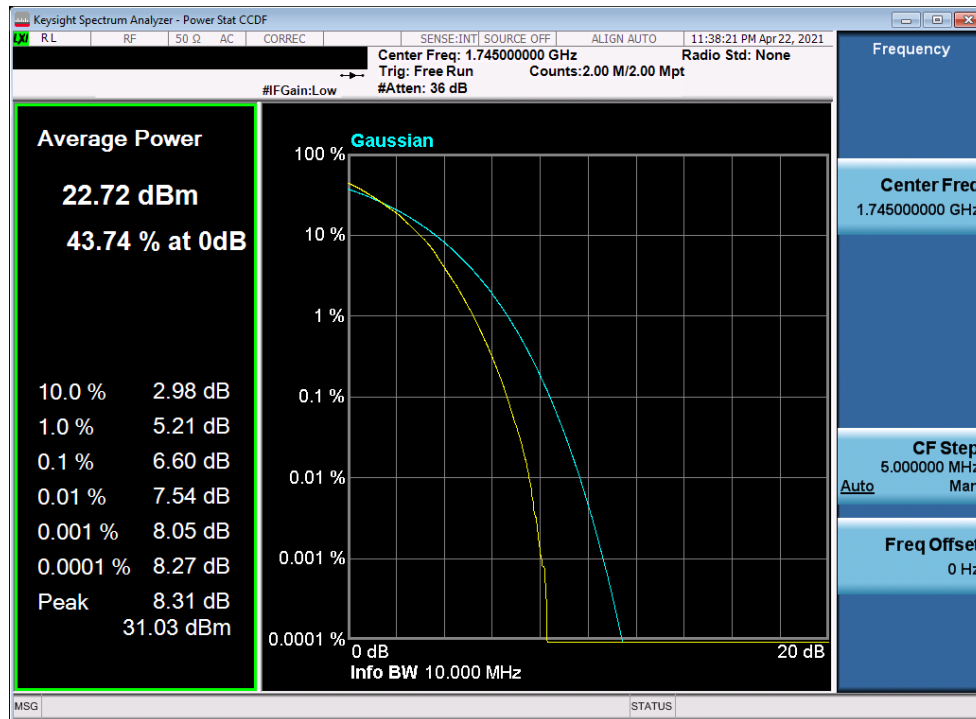
Plot 7-342. PAR Plot (LTE Band 66 - 10MHz 64-QAM - Full RB)
