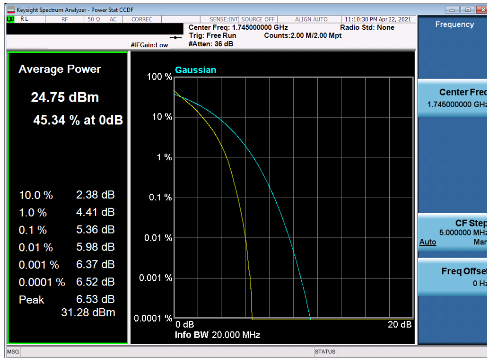
Plot 7-348. PAR Plot (LTE Band 66 - 20MHz QPSK - Full RB)
