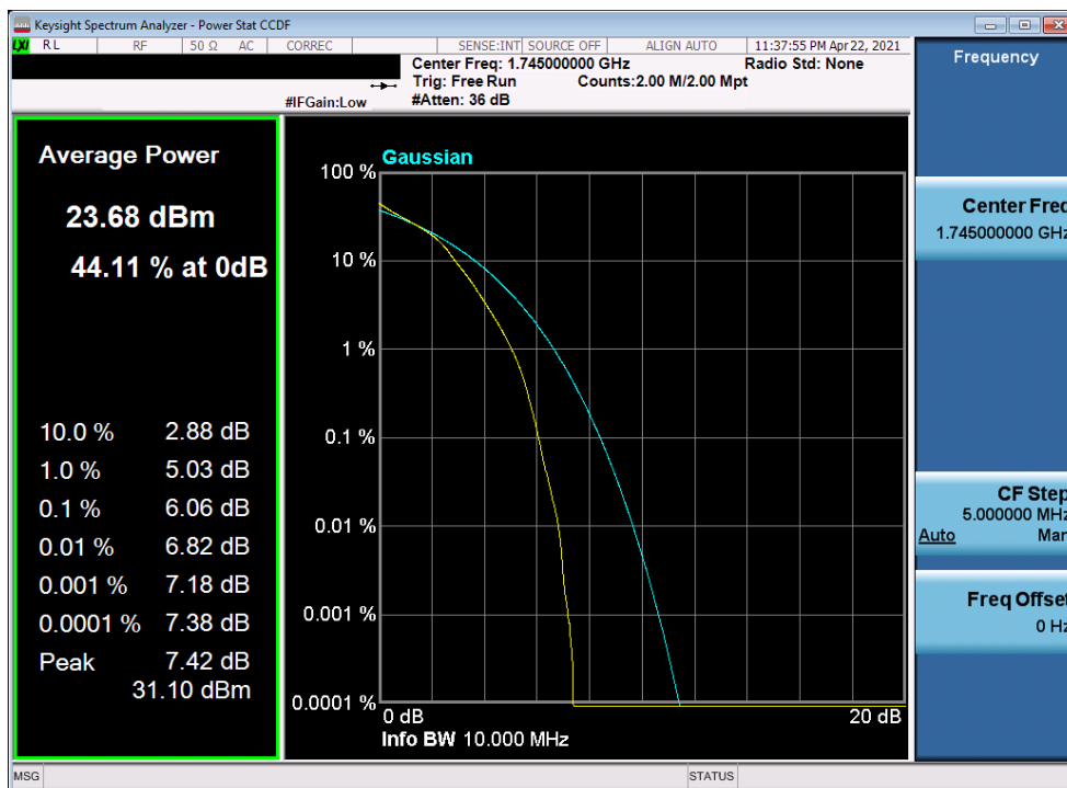
Plot 7-341. PAR Plot (LTE Band 66 - 10MHz 16-QAM - Full RB)
