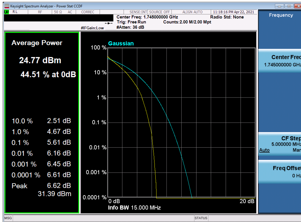
Plot 7-344. PAR Plot (LTE Band 66 - 15MHz QPSK - Full RB)
