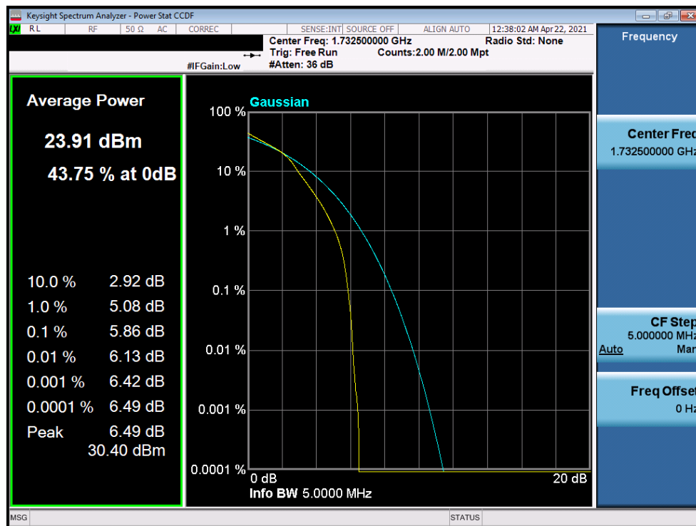
Plot 7-361. PAR Plot (LTE Band 4 - 5MHz 16-QAM - Full RB)
