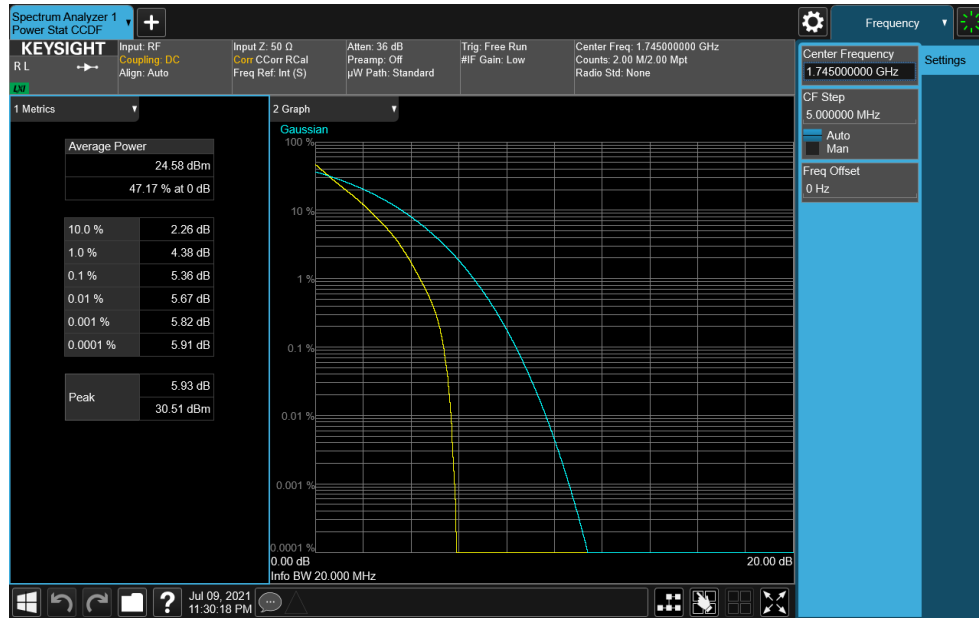
Plot 7-392. PAR Plot (NR Band n66- 20MHz DFT-s-OFDM QPSK - Full RB)
