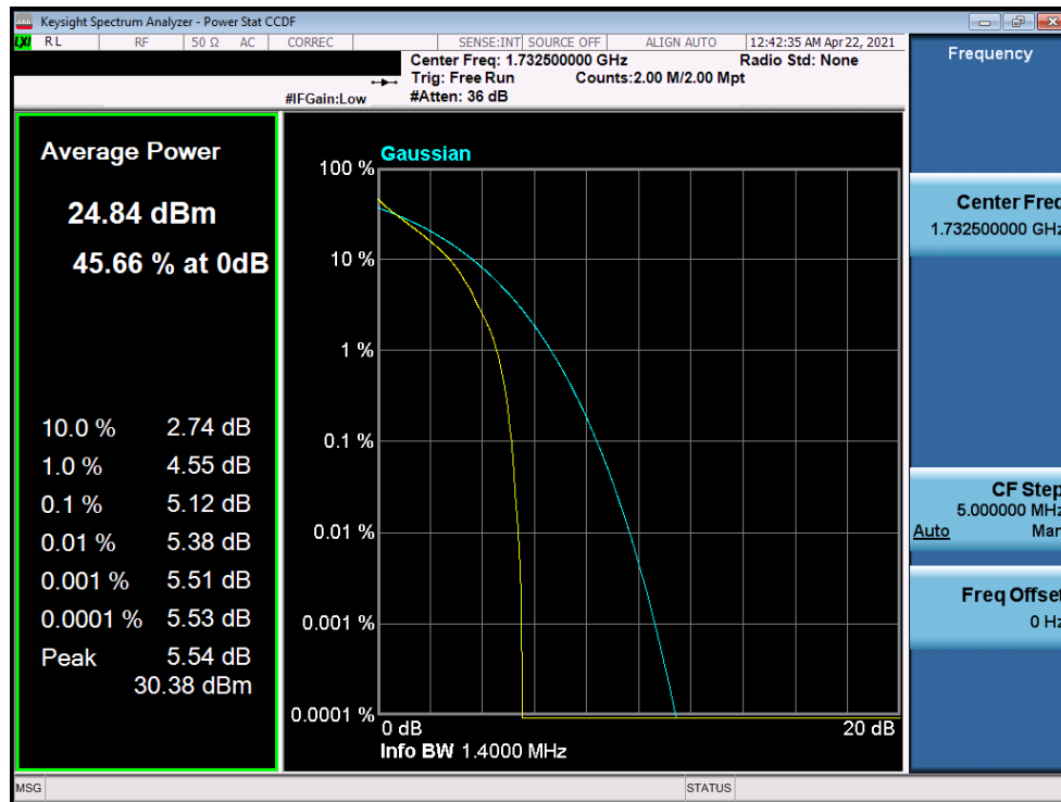
Plot 7-352. PAR Plot (LTE Band 4 - 1.4MHz QPSK - Full RB)
