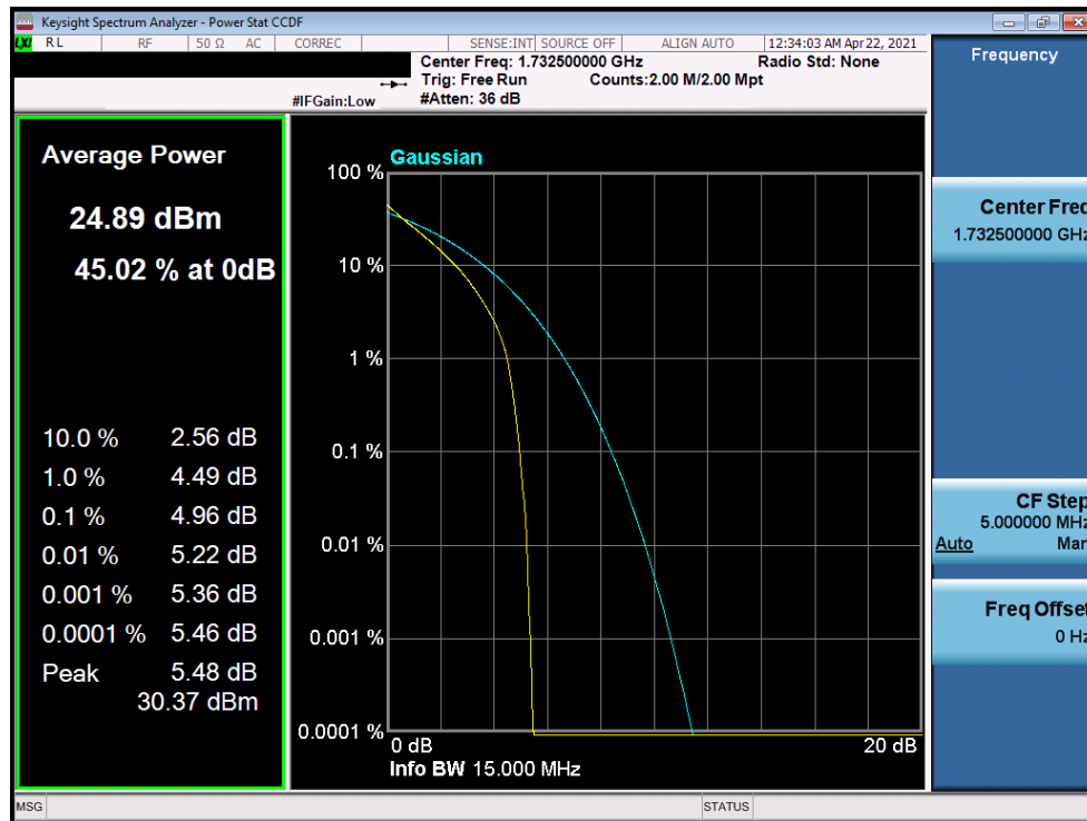
Plot 7-368. PAR Plot (LTE Band 4 - 15MHz QPSK - Full RB)
