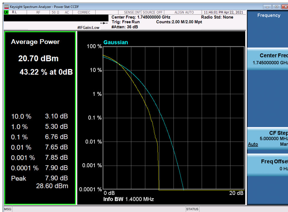
Plot 7-331. PAR Plot (LTE Band 66 - 1.4MHz 256-QAM - Full RB)
