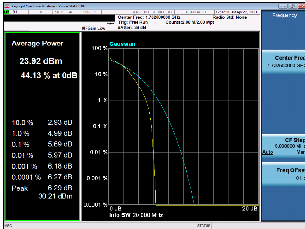
Plot 7-373. PAR Plot (LTE Band 4 - 20MHz 16-QAM - Full RB)
