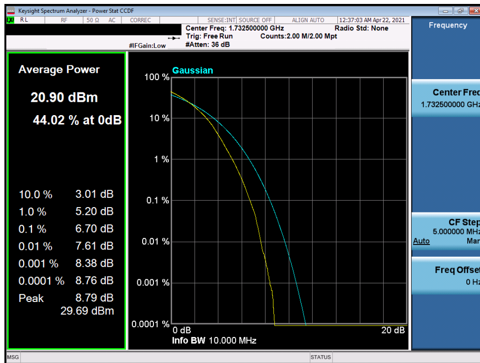
Plot 7-367. PAR Plot (LTE Band 4 - 10MHz 256-QAM - Full RB)
