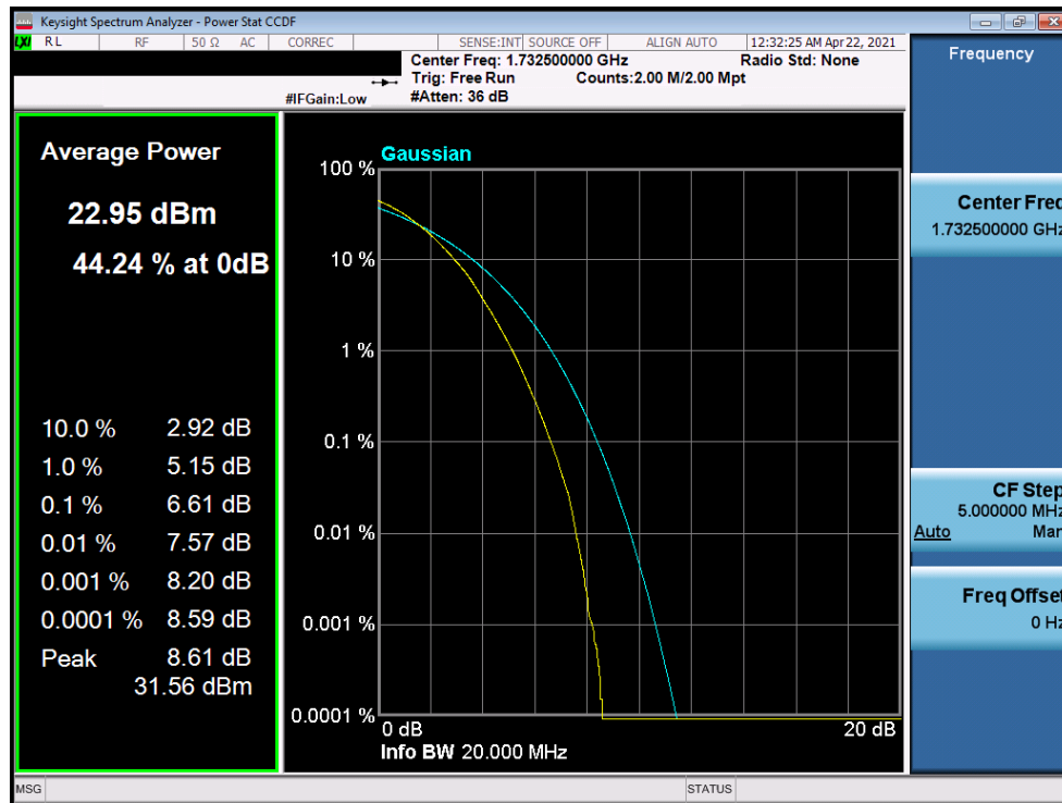
Plot 7-374. PAR Plot (LTE Band 4 - 20MHz 64-QAM - Full RB)
