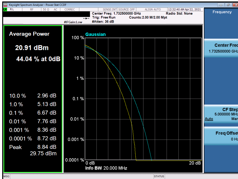
Plot 7-375. PAR Plot (LTE Band 4 - 20MHz 256-QAM - Full RB)
