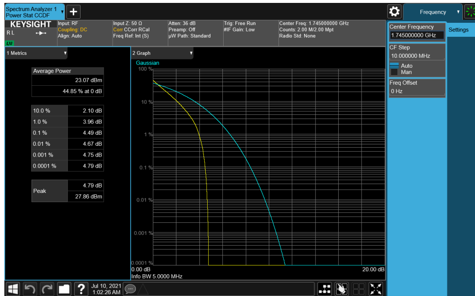
Plot 7-376. PAR Plot (NR Band n66- 5MHz DFT-s-OFDM \pi/2 BPSK - Full RB)
