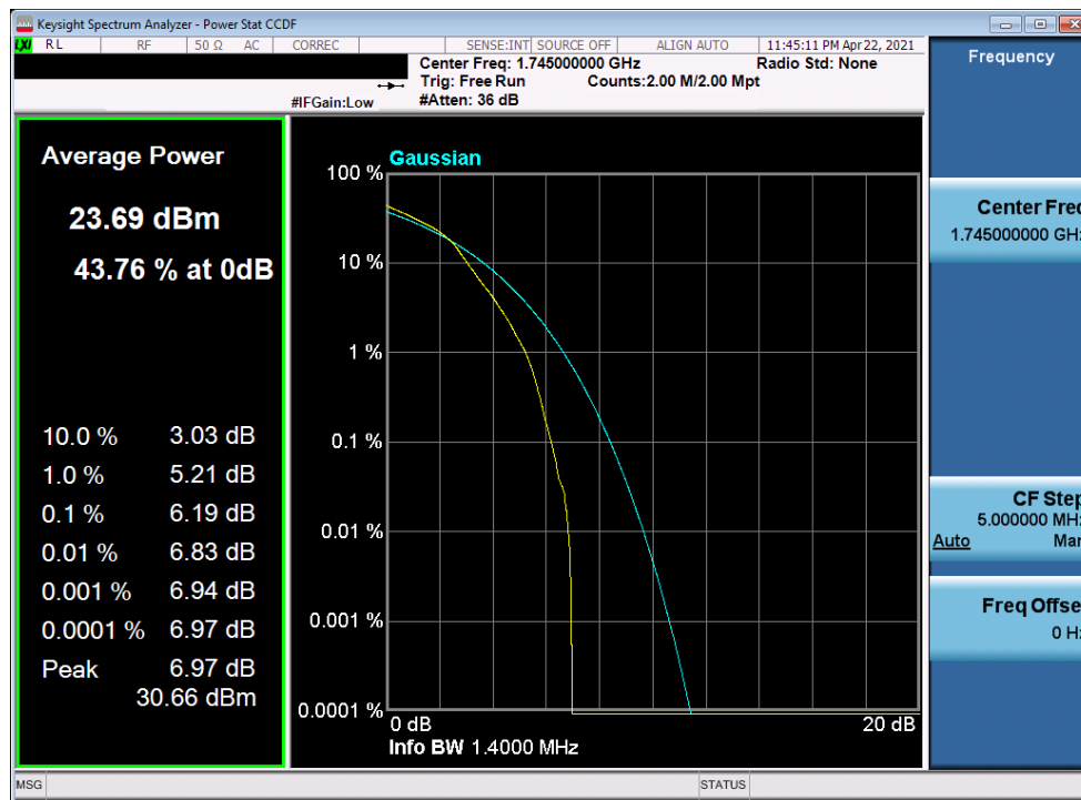
Plot 7-329. PAR Plot (LTE Band 66 - 1.4MHz 16-QAM - Full RB)
