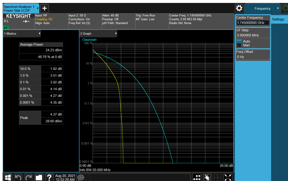
Plot 7-391. PAR Plot (NR Band n66- 20MHz DFT-s-OFDM \pi/2 BPSK - Full RB)
