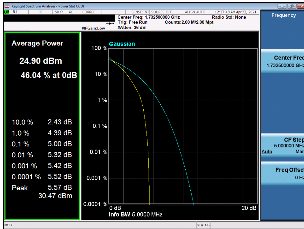
Plot 7-360. PAR Plot (LTE Band 4 - 5MHz QPSK - Full RB)
