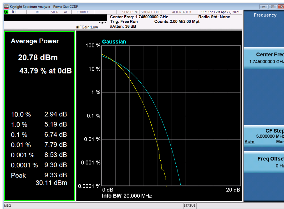
Plot 7-351. PAR Plot (LTE Band 66 - 20MHz 256-QAM - Full RB)
