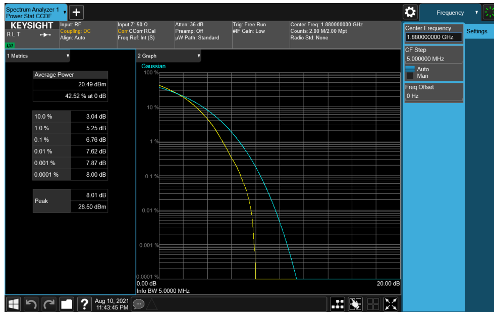
Plot 7-245. PAR Plot (NR Band n2 - 5.0MHz CP-OFDM 256-QAM - Full RB)
