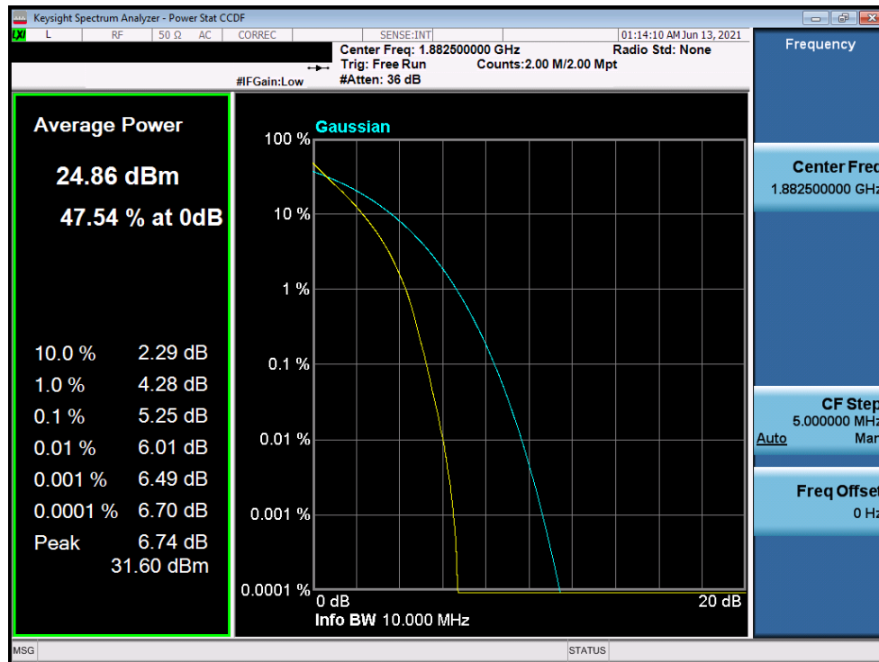
Plot 7-229. PAR Plot (LTE Band 25/2 - 10MHz QPSK - Full RB Configuration)
