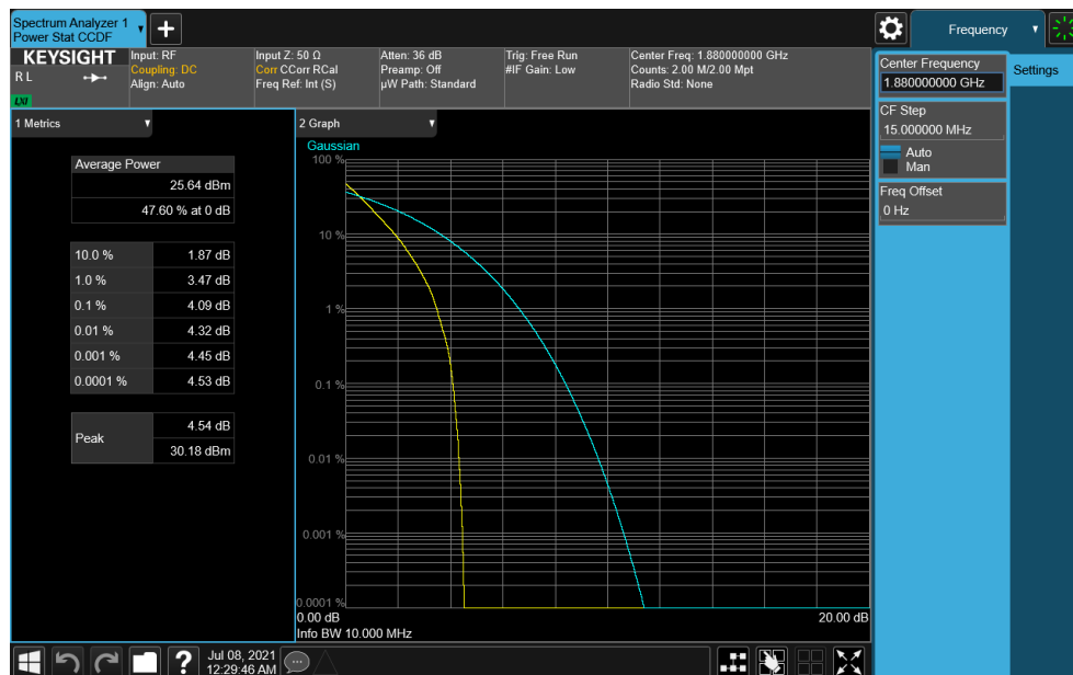
Plot 7-246. PAR Plot (NR Band n2 - 10.0MHz DFT-s-OFDM \pi/2 BPSK - Full RB)
