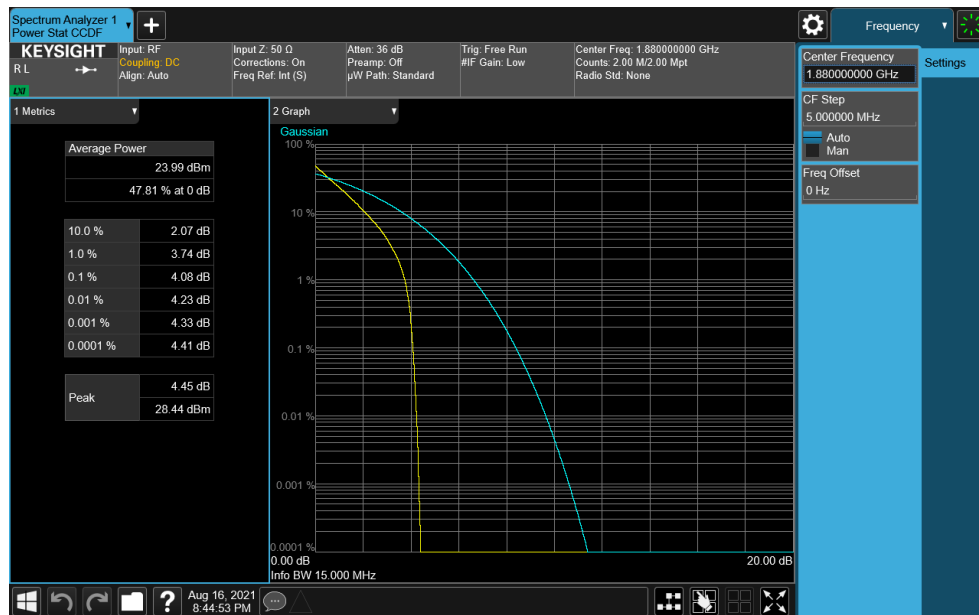
Plot 7-251. PAR Plot (NR Band n2 - 15.0MHz DFT-s-OFDM \pi/2 BPSK - Full RB)
