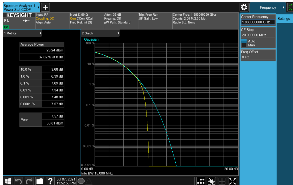
Plot 7-253. PAR Plot (NR Band n2 - 15.0MHz CP-OFDM 16-QAM - Full RB)
