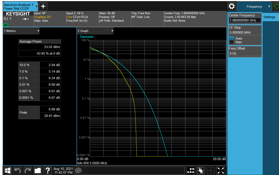
Plot 7-243. PAR Plot (NR Band n2 - 5.0MHz CP-OFDM 16-QAM - Full RB)
