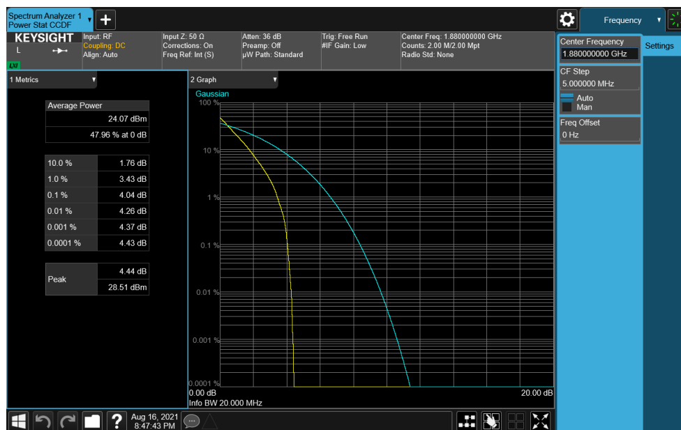
Plot 7-256. PAR Plot (NR Band n2 - 20.0MHz DFT-s-OFDM \pi/2 BPSK - Full RB)
