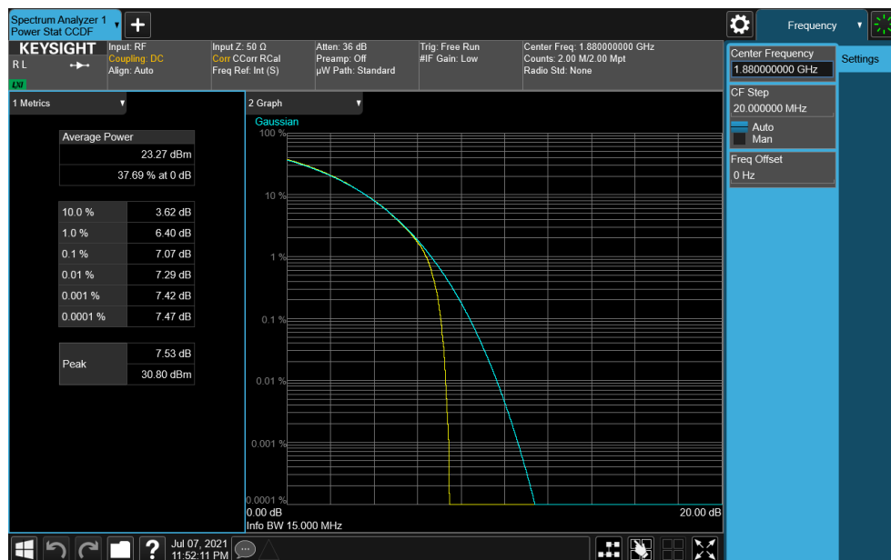
Plot 7-252. PAR Plot (NR Band n2 - 15.0MHz CP-OFDM QPSK - Full RB)
