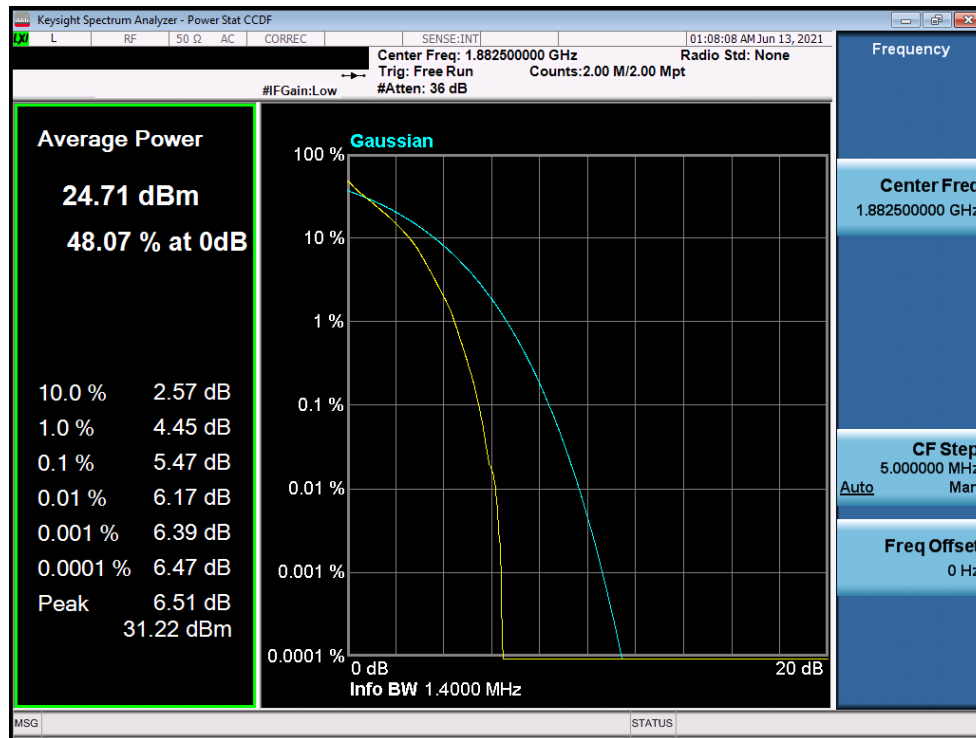
Plot 7-217. PAR Plot (LTE Band 25/2 - 1.4MHz QPSK - Full RB Configuration)
