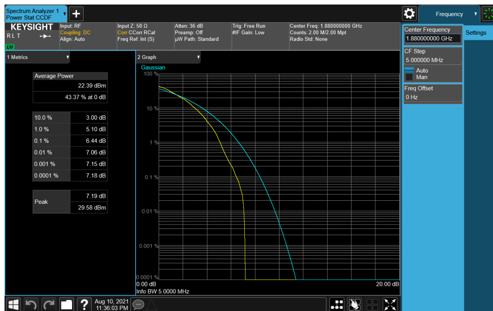
Plot 7-244. PAR Plot (NR Band n2 - 5.0MHz CP-OFDM 64-QAM - Full RB)
