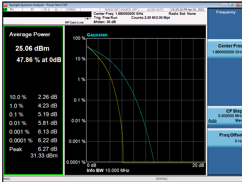
Plot 7-205. PAR Plot (LTE Band 2 - 10MHz QPSK - Full RB Configuration)
