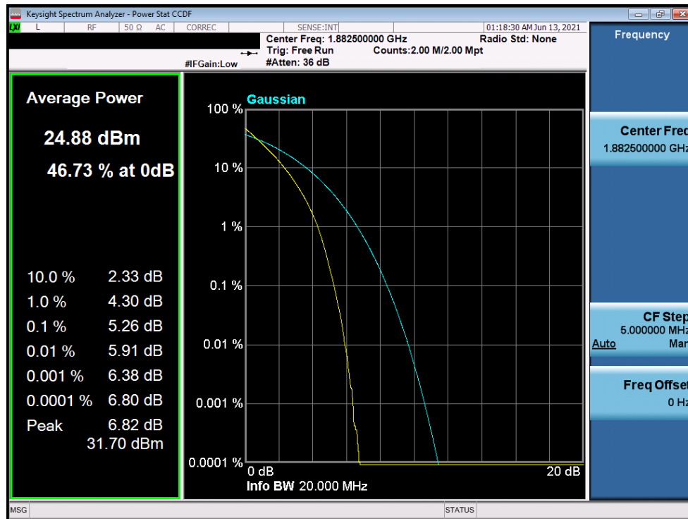
Plot 7-237. PAR Plot (LTE Band 25/2 - 20MHz QPSK - Full RB Configuration)
