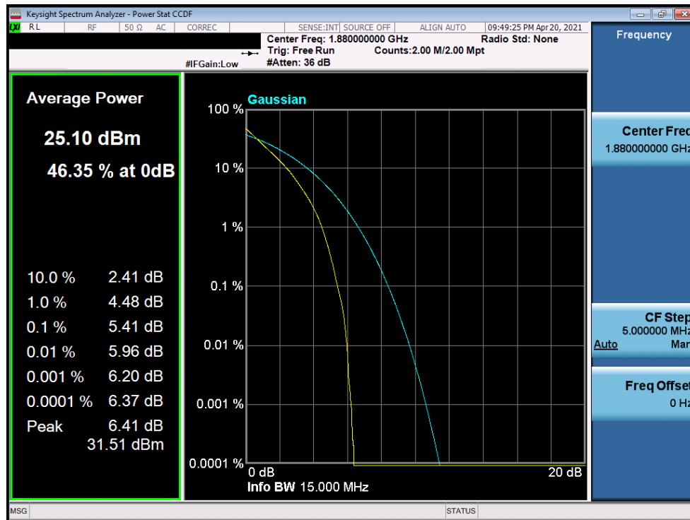
Plot 7-209. PAR Plot (LTE Band 2 - 15MHz QPSK - Full RB Configuration)
