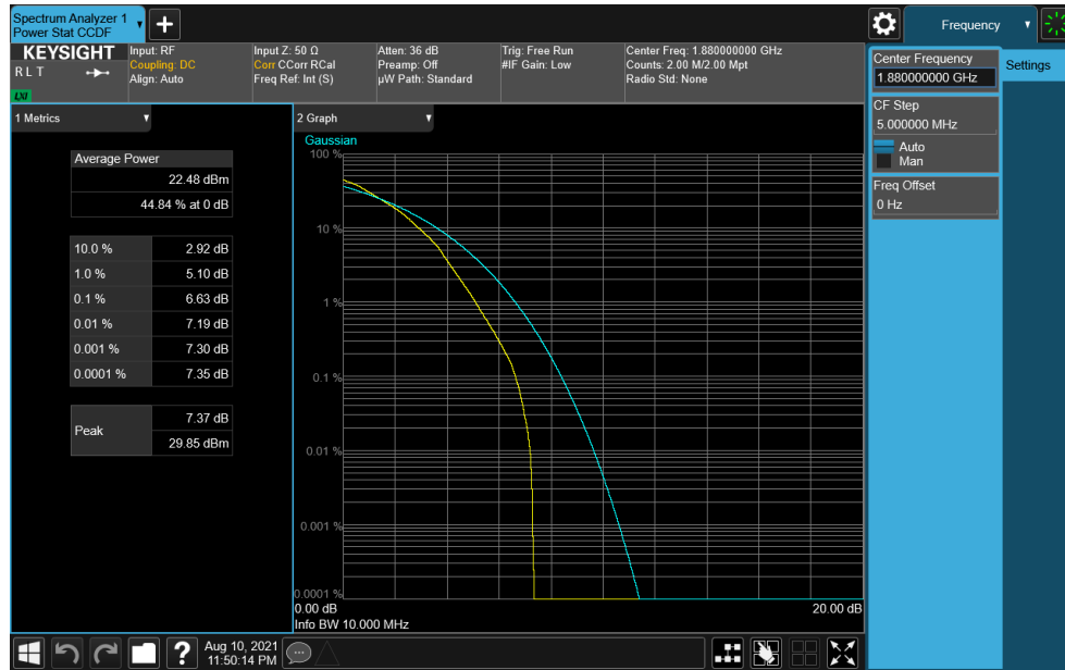
Plot 7-249. PAR Plot (NR Band n2 - 10.0MHz CP-OFDM 64-QAM - Full RB)
