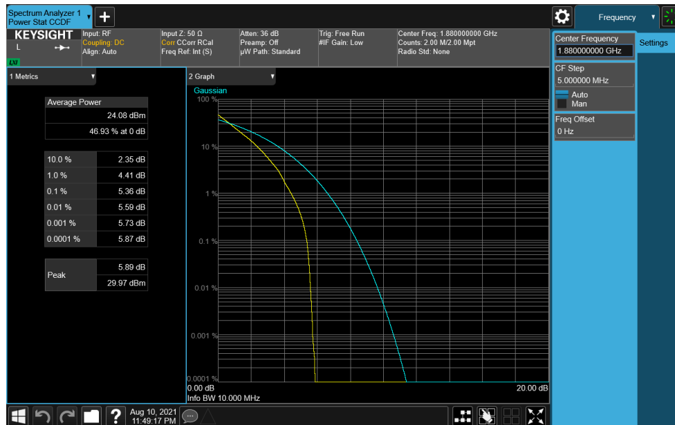
Plot 7-247. PAR Plot (NR Band n2 - 10.0MHz CP-OFDM QPSK - Full RB)
