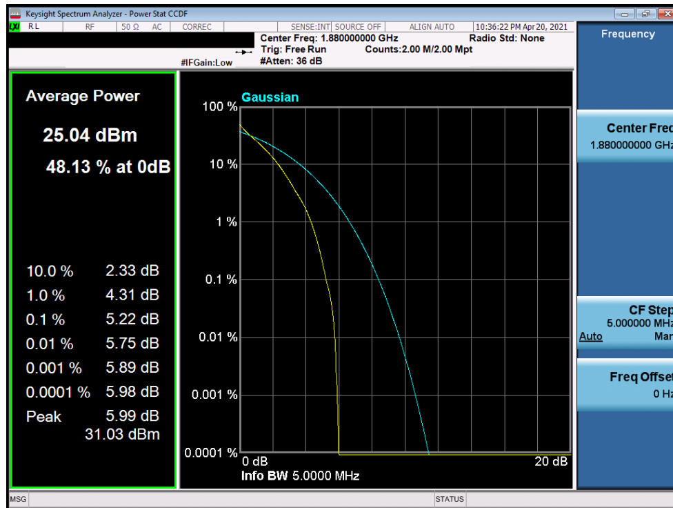
Plot 7-201. PAR Plot (LTE Band 2 - 5MHz QPSK - Full RB Configuration)
