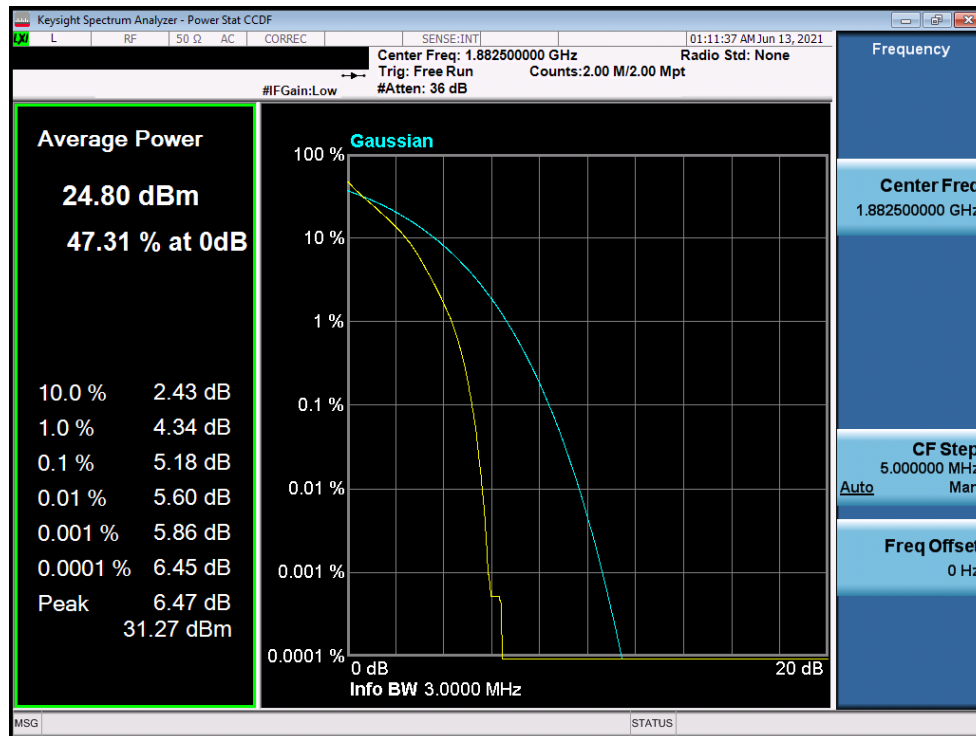
Plot 7-221. PAR Plot (LTE Band 25/2 - 3MHz QPSK - Full RB Configuration)
