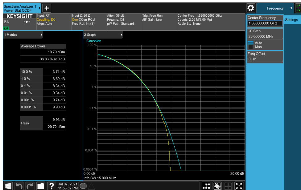
Plot 7-255. PAR Plot (NR Band n2 - 15.0MHz CP-OFDM 256-QAM - Full RB)
