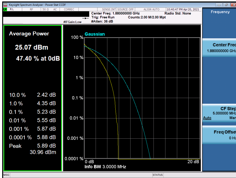
Plot 7-197. PAR Plot (LTE Band 2 - 3MHz QPSK - Full RB Configuration)
