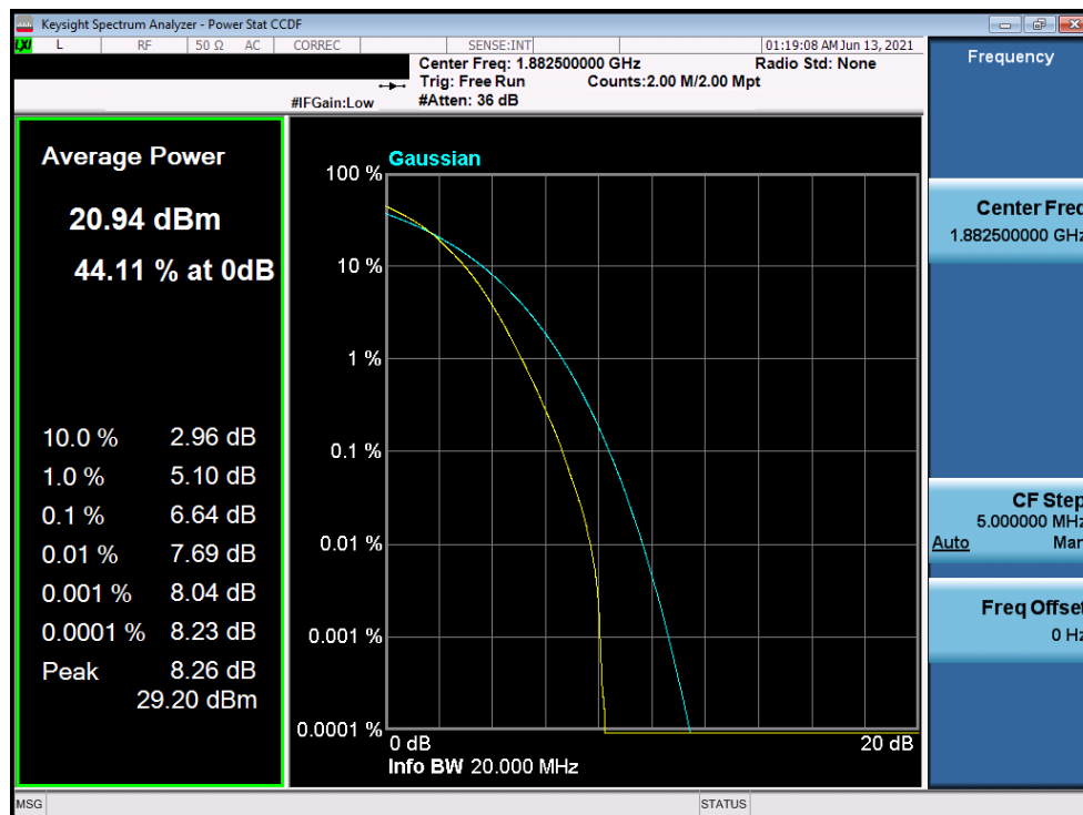
Plot 7-240. PAR Plot (LTE Band 25/2 - 20MHz 256-QAM - Full RB Configuration)
