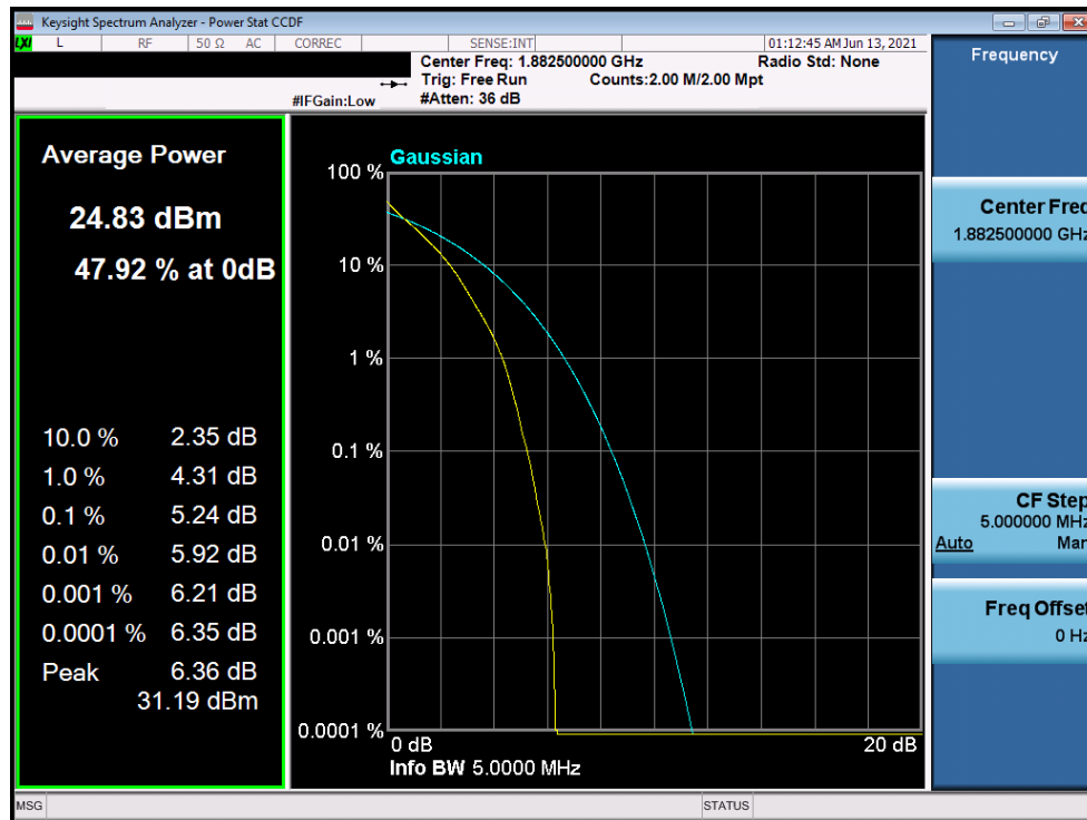
Plot 7-225. PAR Plot (LTE Band 25/2 - 5MHz QPSK - Full RB Configuration)
