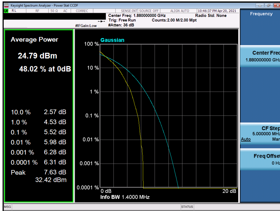
Plot 7-193. PAR Plot (LTE Band 2 - 1.4MHz QPSK - Full RB Configuration)
