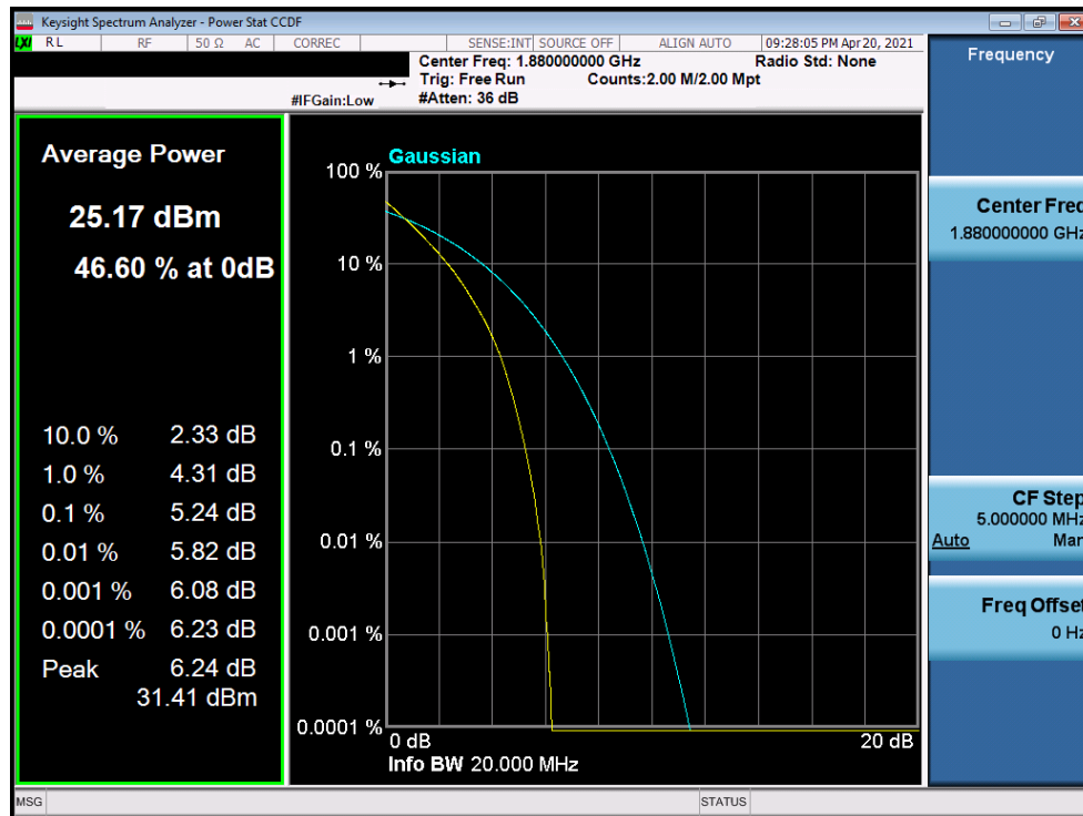
Plot 7-213. PAR Plot (LTE Band 2 - 20MHz QPSK - Full RB Configuration)
