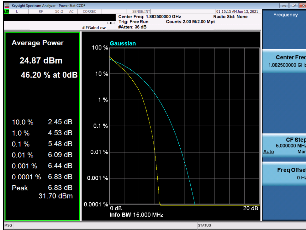
Plot 7-233. PAR Plot (LTE Band 25/2 - 15MHz QPSK - Full RB Configuration)
