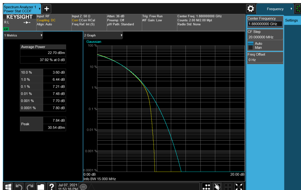
Plot 7-254. PAR Plot (NR Band n2 - 15.0MHz CP-OFDM 64-QAM - Full RB)
