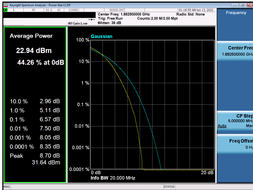
Plot 7-239. PAR Plot (LTE Band 25/2 - 20MHz 64-QAM - Full RB Configuration)
