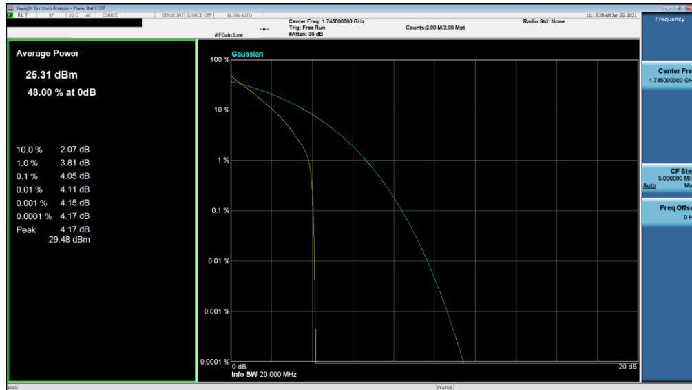
Plot 7-360. PAR Plot (NR Band n66 - 5.0MHz DFT-s-OFDM π/2 BPSK - Full RB)
