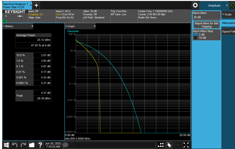
Plot 7-399. PAR Plot (NR Band n66 - 5.0MHz DFT-s-OFDM \pi/2 BPSK - Full RB)
