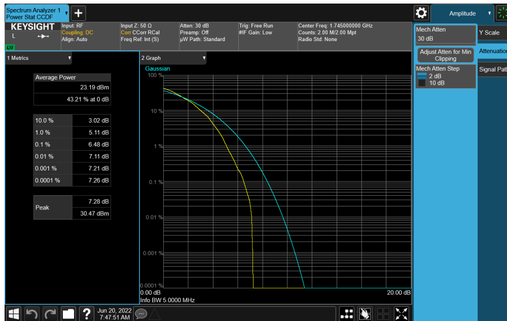
Plot 7-402. PAR Plot (NR Band n66 - 5.0MHz DFT-s-OFDM 64-QAM - Full RB)
