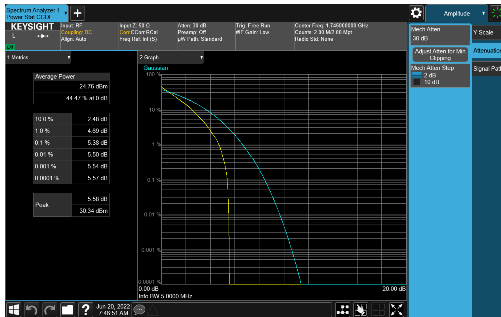
Plot 7-400. PAR Plot (NR Band n66 - 5.0MHz DFT-s-OFDM QPSK - Full RB)
