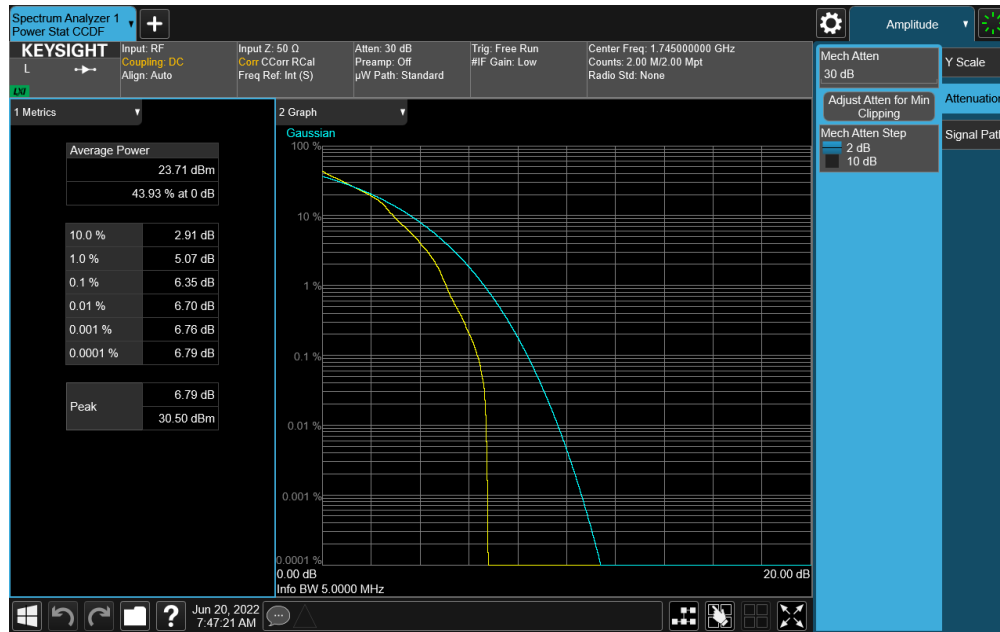
Plot 7-401. PAR Plot (NR Band n66 - 5.0MHz DFT-s-OFDM 16-QAM - Full RB)
