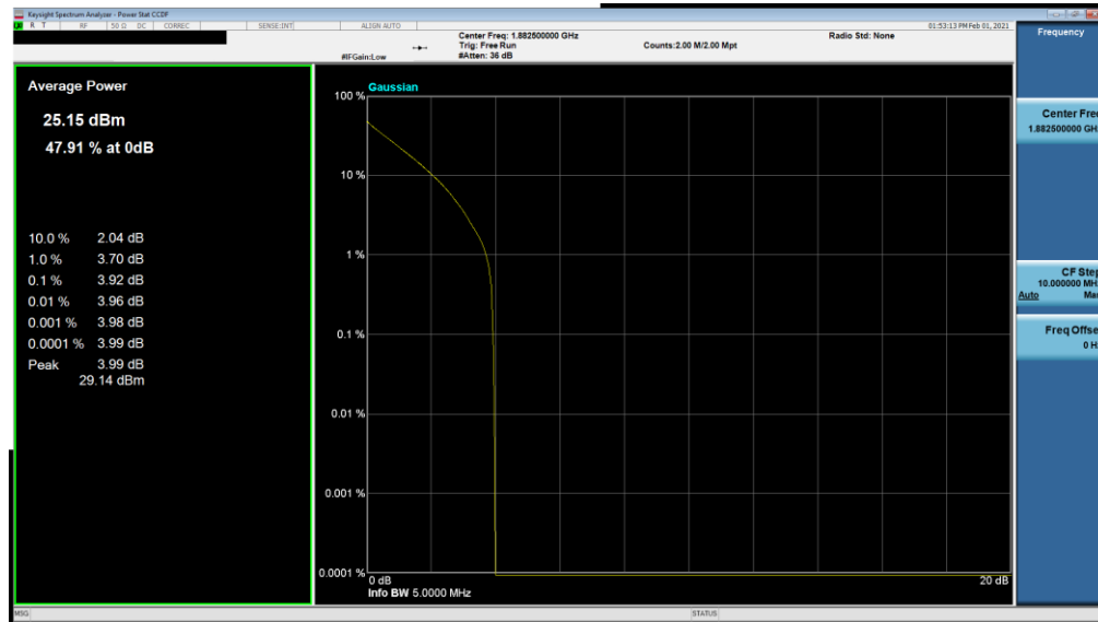
Plot 7-235. PAR Plot (NR Band n25 - 5.0MHz DFT-s-OFDM \pi/2 BPSK - Full RB)
