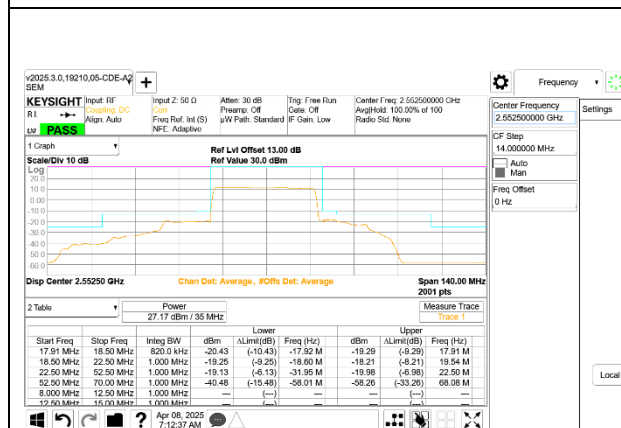
5G NR n7 35MHz BPSK High Channel RB180-0
