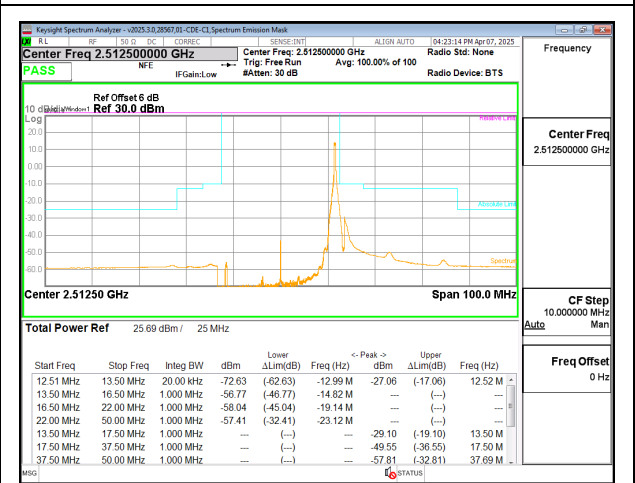
5G NR n41 25MHz BPSK Low Channel RB1-64
