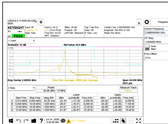
5G NR n41 10MHz BPSK High Channel RB1-0
