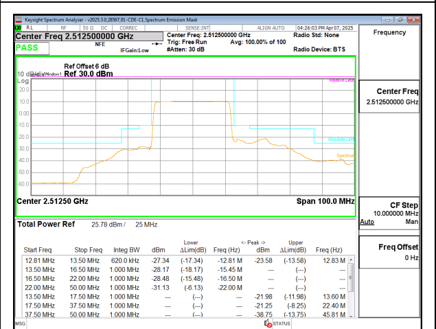
5G NR n41 25MHz BPSK Low Channel RB64-0
