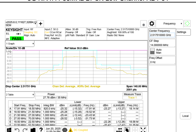
5G NR n41 35MHz BPSK Low Channel RB90-0
