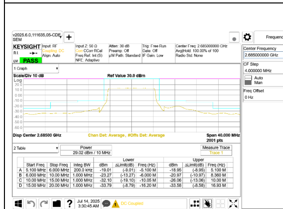
5G NR n41 10MHz BPSK High Channel RB24-0
