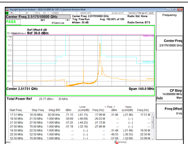
5G NR n41 35MHz BPSK Low Channel RB1-91
