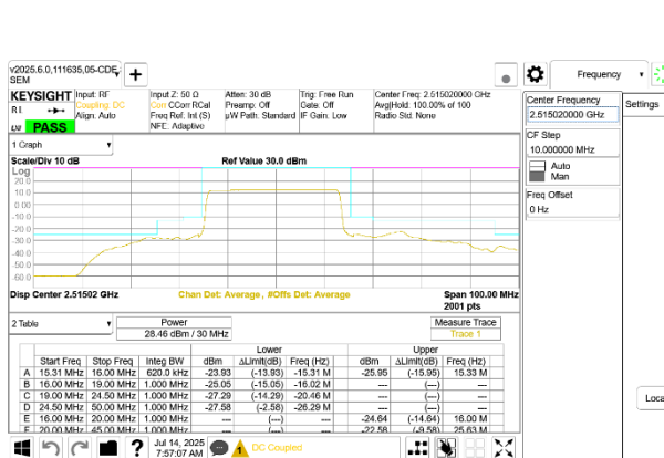
5G NR n41 30MHz BPSK Low Channel RB75-0
