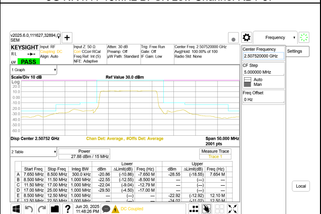
5G NR n41 15MHz BPSK Low Channel RB36-0
