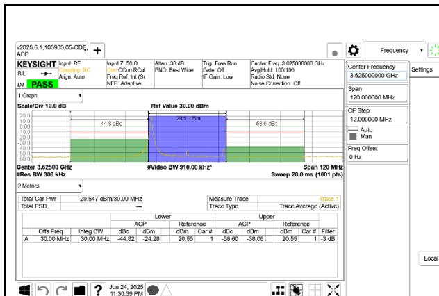
5G NR n48 30MHz QPSK Mid Channel RB1-0 Port A:
