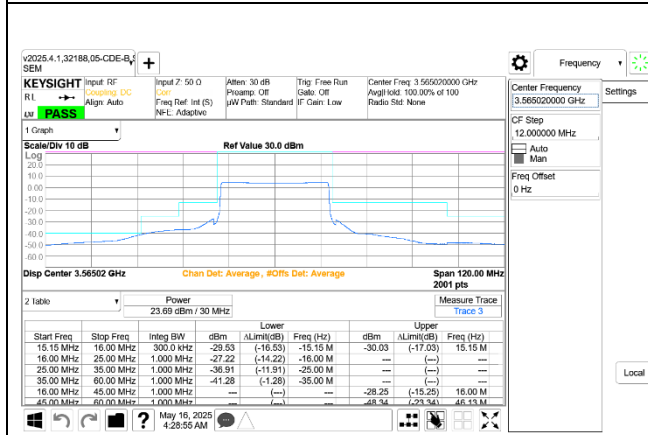
5G NR n48 30MHz QPSK Low Channel RB78-0 Ant 9+8
