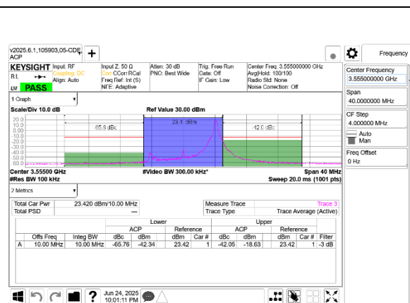
5G NR n48 10MHz QPSK Low Channel RB1-23 Port A+B
