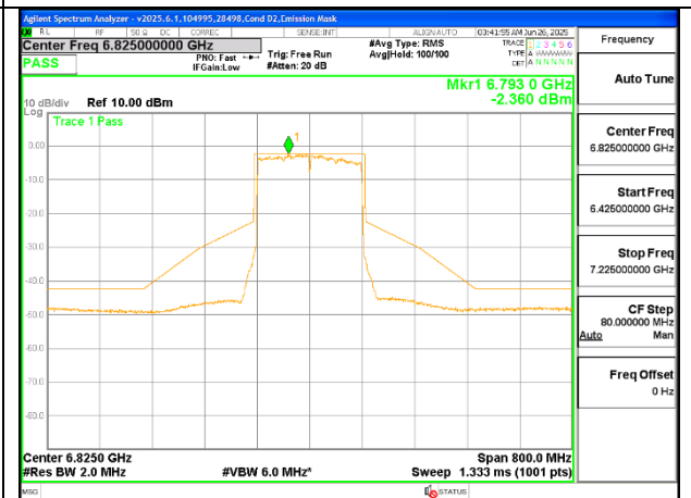
STRADDLE ANT 5 6825
