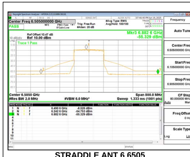
STRADDLE ANT 6 6505
