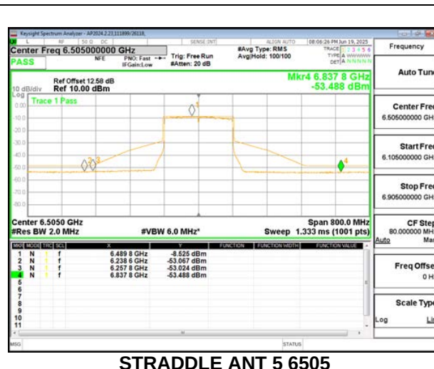
STRADDLE ANT 5 6505
