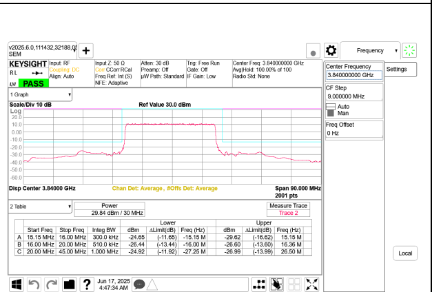
5G NR n77 30MHz BPSK Mid Channel RB75-0 Port B
