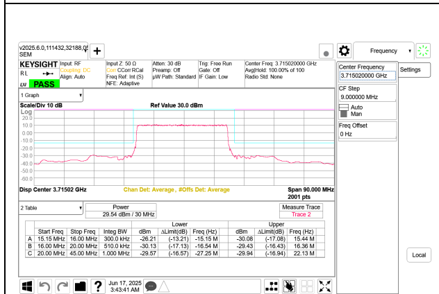
5G NR n77 30MHz BPSK Low Channel RB75-0 Port B
