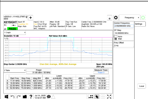
5G NR n41 35MHz BPSK Mid Channel RB90-0 Port A+B
