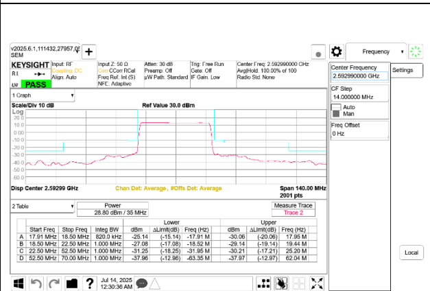
5G NR n41 35MHz BPSK Mid Channel RB90-0 Port B
