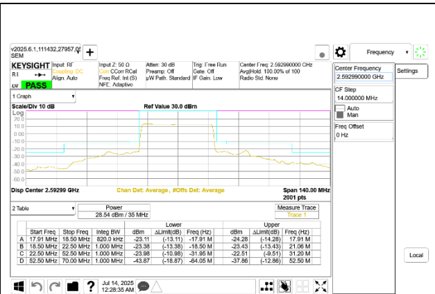
5G NR n41 35MHz BPSK Mid Channel RB90-0 Port A
