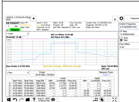
5G NR n41 35MHz BPSK Low Channel RB90-0 Port A+B
