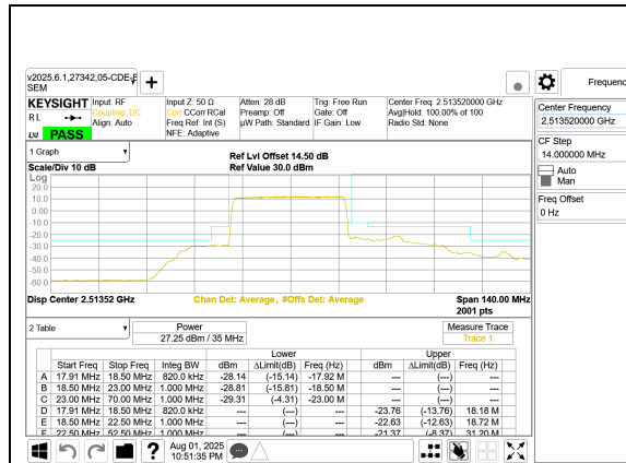
5G NR n41 35MHz BPSK Low Channel RB90-0 Port A
