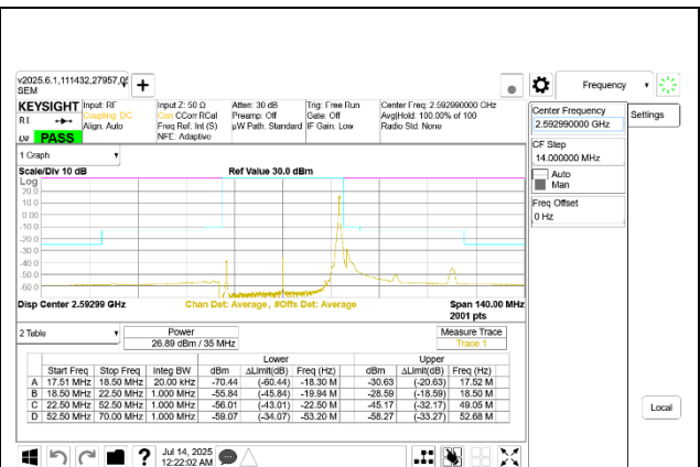
5G NR n41 35MHz BPSK Mid Channel RB1-91 Port A
