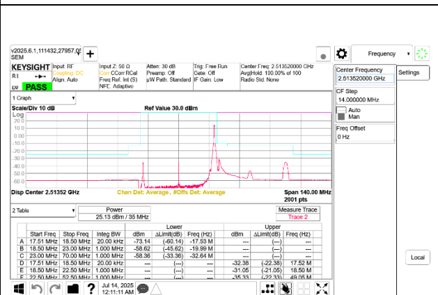
5G NR n41 35MHz BPSK Low Channel RB1-91 Port B
