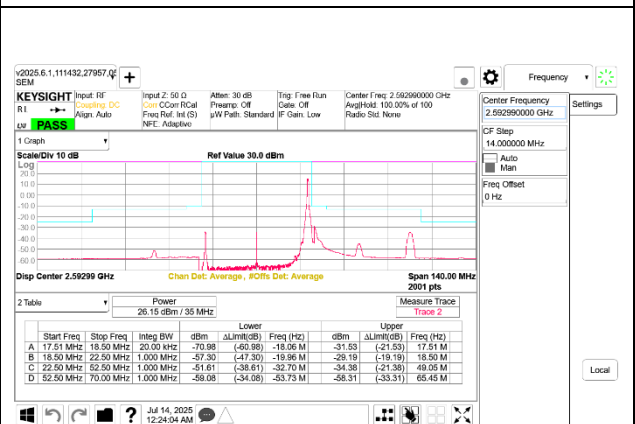
5G NR n41 35MHz BPSK Mid Channel RB1-91 Port B
