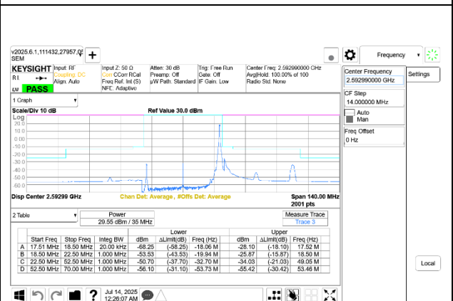
5G NR n41 35MHz BPSK Mid Channel RB1-91 Port A+B
