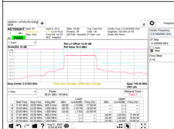
5G NR n41 35MHz BPSK Low Channel RB90-0 Port B
