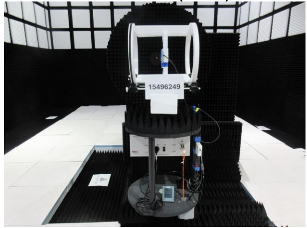
170 - 200 GHz (BACK)
