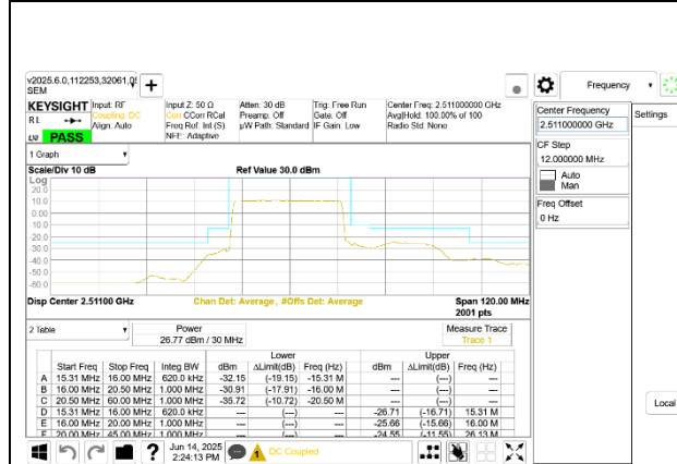
5G NR n41 30MHz BPSK Low Channel RB75-0
