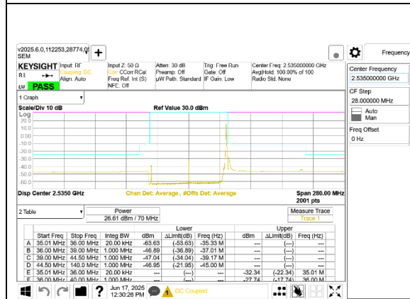
5G NR n41 70MHz BPSK Low Channel RB1-188
