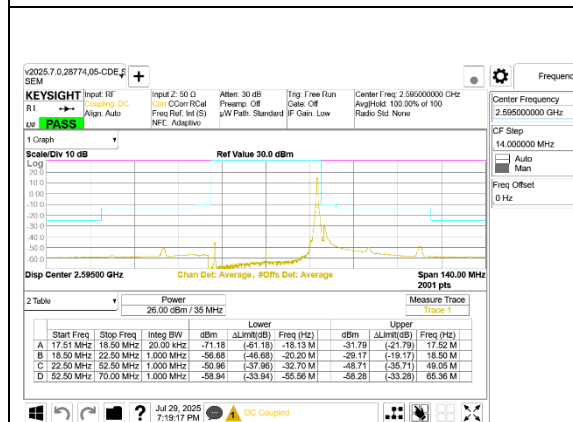
5G NR n41 35MHz BPSK Middle Channel RB1-91
