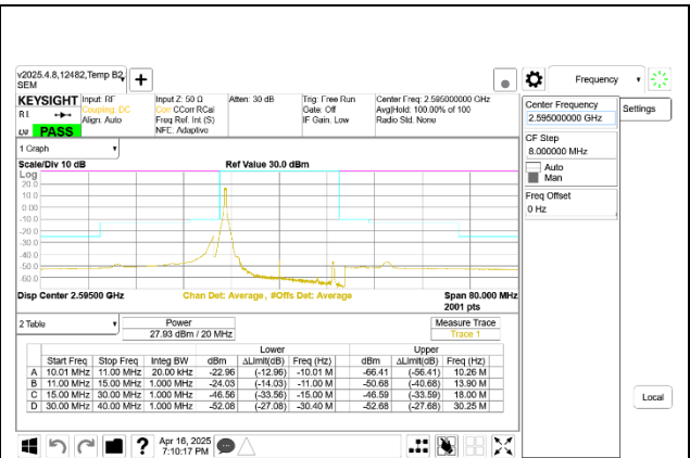
5G NR n41 20MHz BPSK Middle Channel RB1-0
