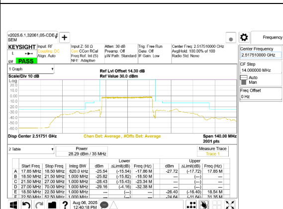
5G NR n41 35MHz BPSK Low Channel RB90-0
