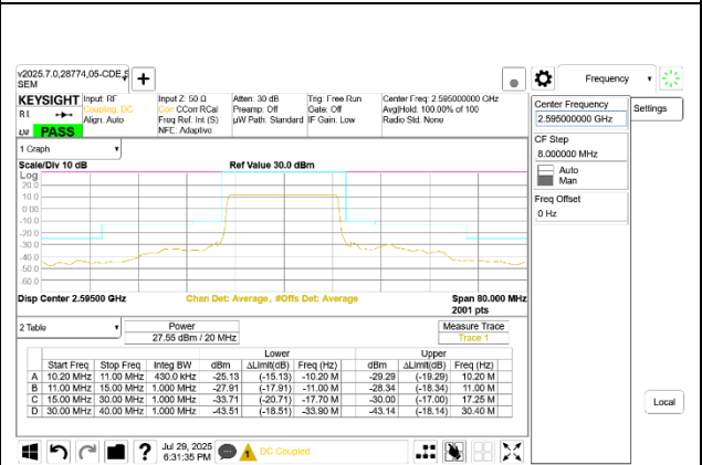
5G NR n41 20MHz BPSK Middle Channel RB50-0
