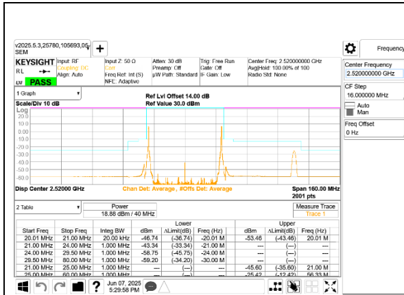
ULCA LTE B7 20MHz + 20MHz QPSK Low Ch RB1-0 + RB1-99
