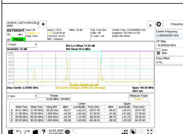
ULCA LTE B7 20MHz + 20MHz QPSK High Ch RB1-0 + RB1-99
