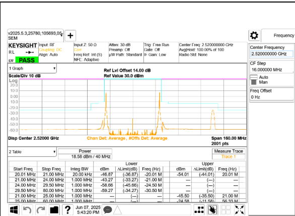
ULCA LTE B7 20MHz + 20MHz 16QAM Low Ch RB1-0 + RB1-99
