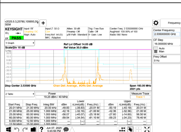
ULCA LTE B7 20MHz + 20MHz 16QAM Mid Ch RB1-0 + RB1-99
