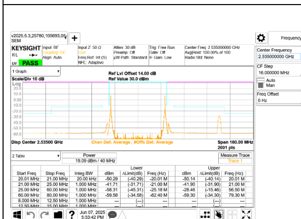
ULCA LTE B7 20MHz + 20MHz QPSK Mid Ch RB1-0 + RB1-99
