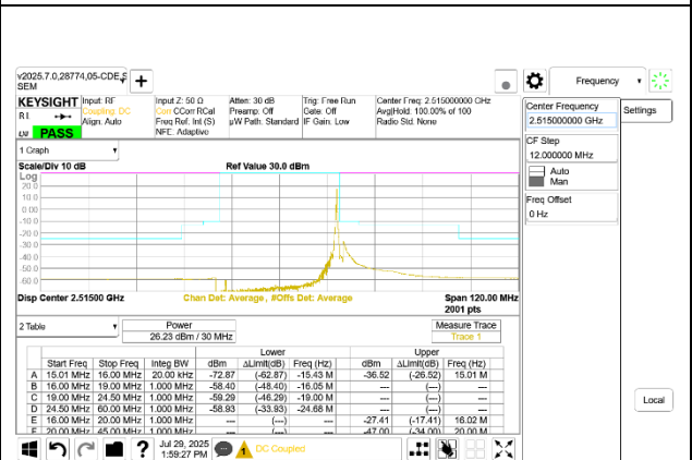
5G NR n7 30MHz BPSK Low Channel RB1-159
