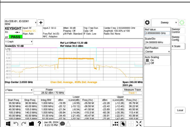
5G NR n41 70MHz BPSK High Channel RB180-0
