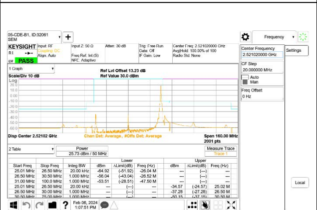
5G NR n41 50MHz BPSK Low Channel RB1-132
