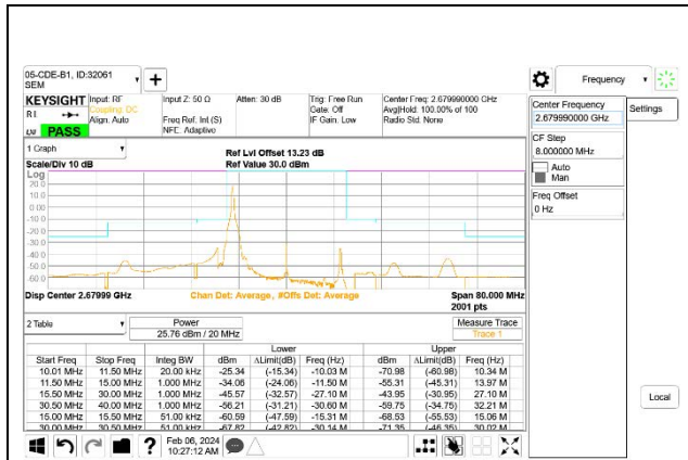
5G NR n41 20MHz BPSK High Channel RB1-0
