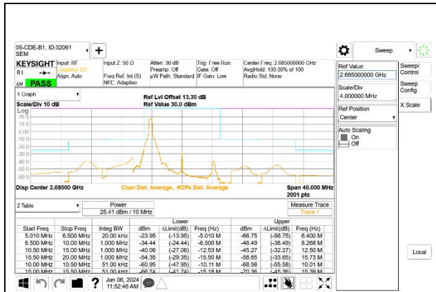
5G NR n41 10MHz BPSK High Channel RB1-0
