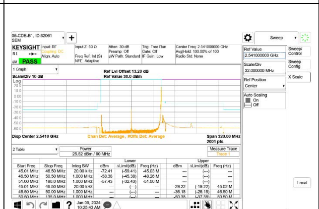
5G NR n41 90MHz BPSK Low Channel RB1-244
