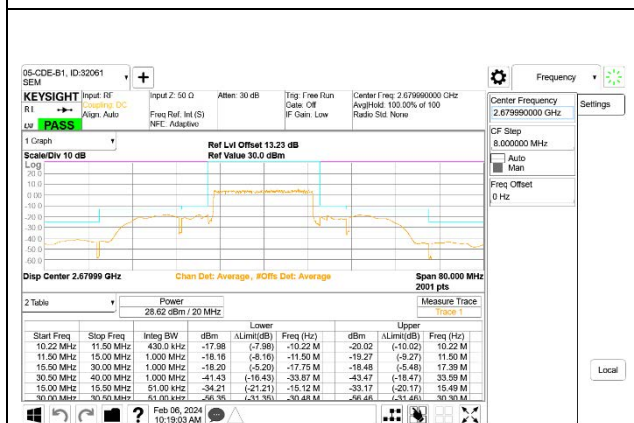
5G NR n41 20MHz BPSK High Channel RB50-0
