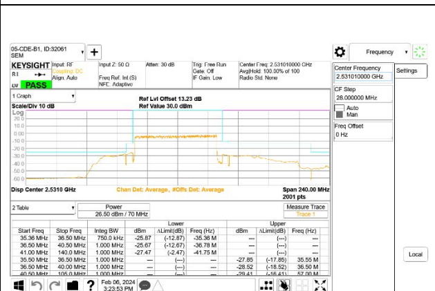
5G NR n41 70MHz BPSK Low Channel RB180-0
