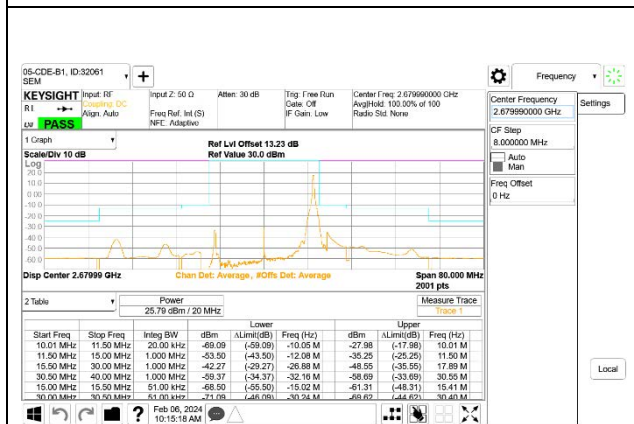
5G NR n41 20MHz BPSK High Channel RB1-50
