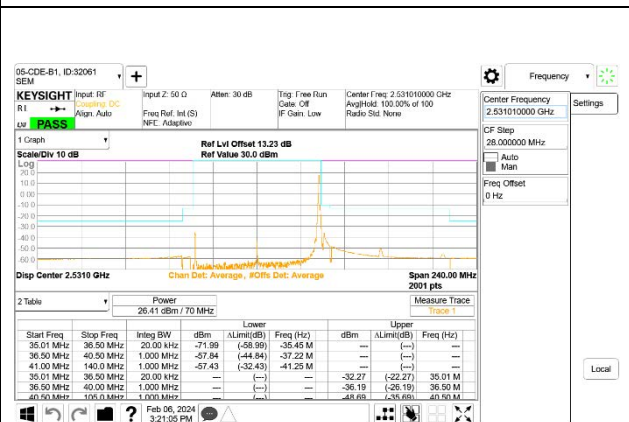
5G NR n41 70MHz BPSK Low Channel RB1-188
