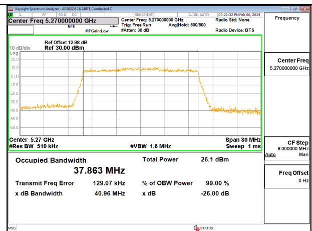
40MHz - Low Channel - SU (UNII-2a) - Ant 2
