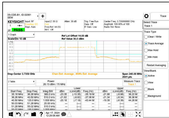
5G NR n77 70MHz BPSK Low Channel RB180-0 Port A
