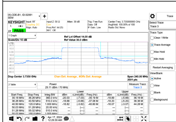
5G NR n77 70MHz BPSK Low Channel RB180-0 Port A+B
