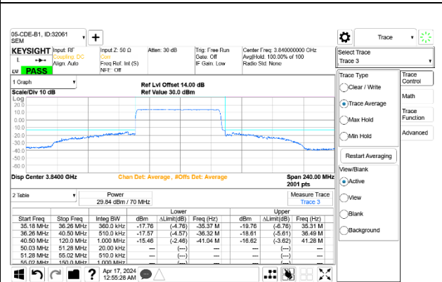
5G NR n77 70MHz BPSK Mid Channel RB180-0 Port A+B
