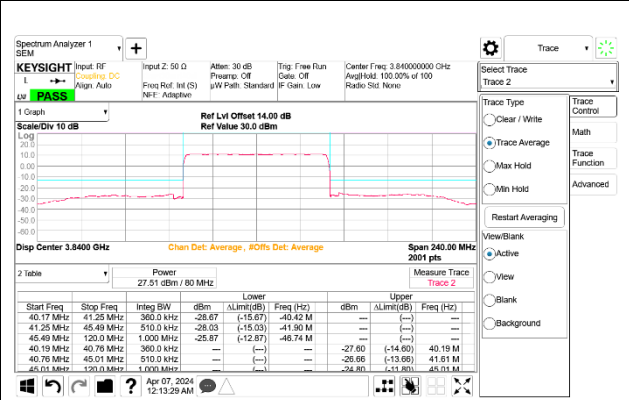
5G NR n77 80MHz BPSK Mid Channel RB216-0 Port B ID 27342
