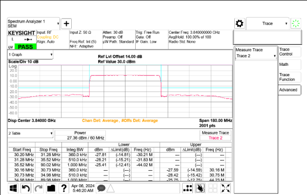
5G NR n77 60MHz BPSK Mid Channel RB162-0 Port B
