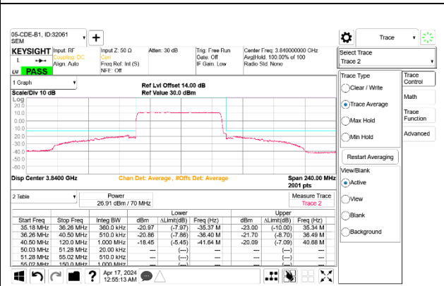
5G NR n77 70MHz BPSK Mid Channel RB180-0 Port B
