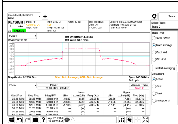
5G NR n77 70MHz BPSK Low Channel RB180-0 Port B
