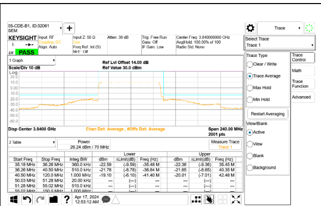
5G NR n77 70MHz BPSK Mid Channel RB180-0 Port A
