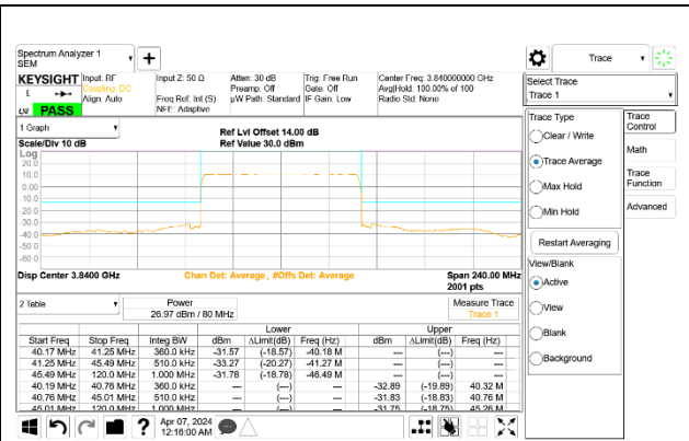
5G NR n77 80MHz BPSK Mid Channel RB216 -0 Port A ID 27342
