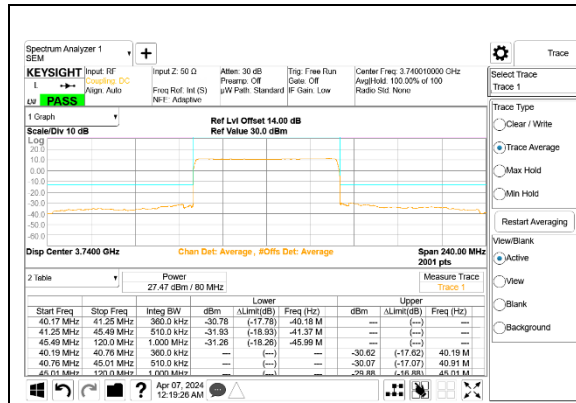
5G NR n77 80MHz BPSK Low Channel RB216 -0 Port A ID 27342
