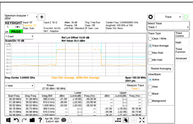
5G NR n77 60MHz BPSK Mid Channel RB162-0 Port A
