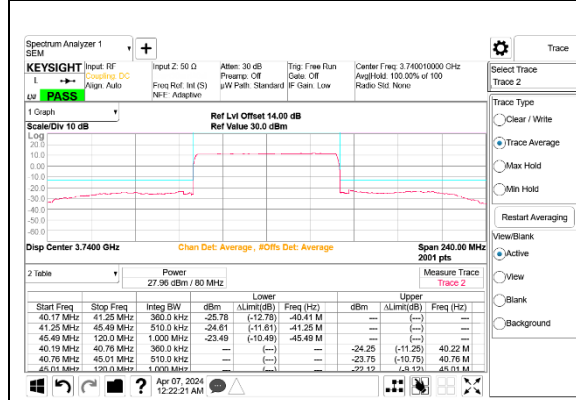
5G NR n77 80MHz BPSK Low Channel RB216-0 Port B ID 27342
