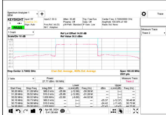
5G NR n77 60MHz BPSK Low Channel RB162-0 Port B
