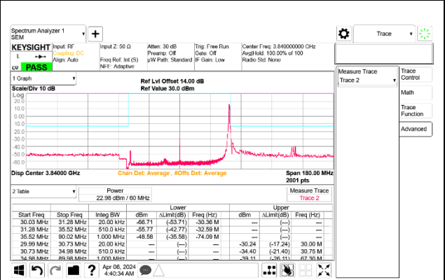
5G NR n77 60MHz BPSK Mid Channel RB1-161 Port B
