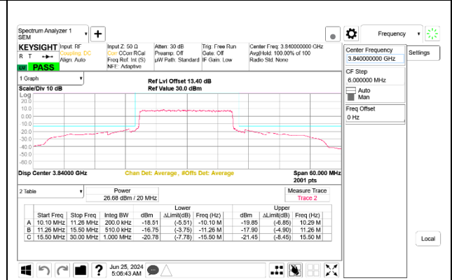
5G NR n77 20MHz BPSK Mid Channel RB50-0 Port B ID 27342
