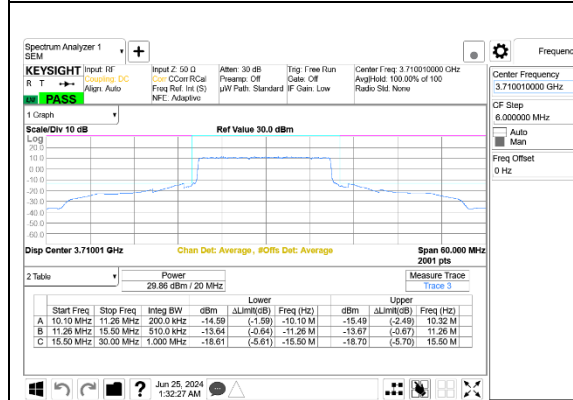
5G NR n77 20MHz BPSK Low Channel RB50-0 Port A+B ID 27342
