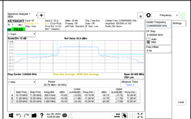
5G NR n77 20MHz BPSK Mid Channel RB50-0 Port A+B ID 27342
