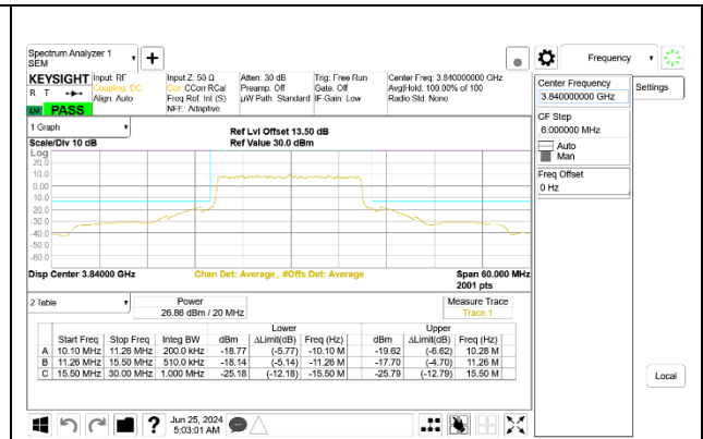
5G NR n77 20MHz BPSK Mid Channel RB50-0 Port A ID 27342
