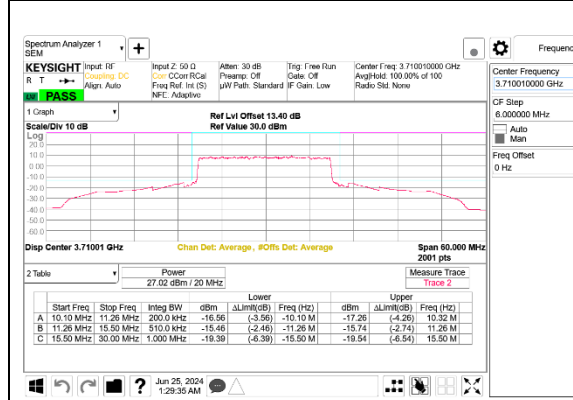
5G NR n77 20MHz BPSK Low Channel RB50-0 Port B ID 27342
