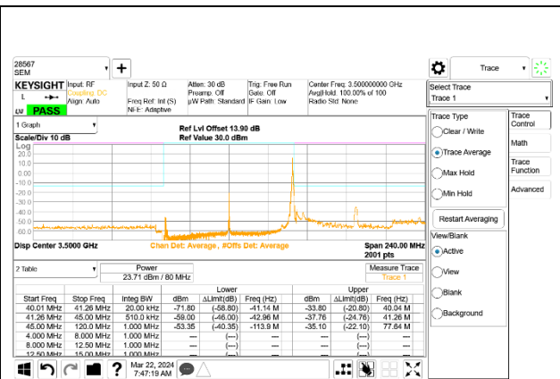
5G NR n77 80MHz BPSK Mid Channel RB1-216 Port A
