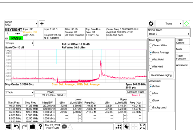
5G NR n77 80MHz BPSK Mid Channel RB1-216 Port B
