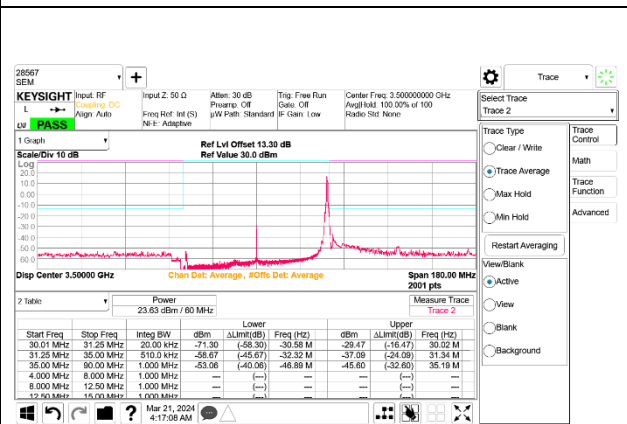
5G NR n77 60MHz BPSK Mid Channel RB1-161 Port B
