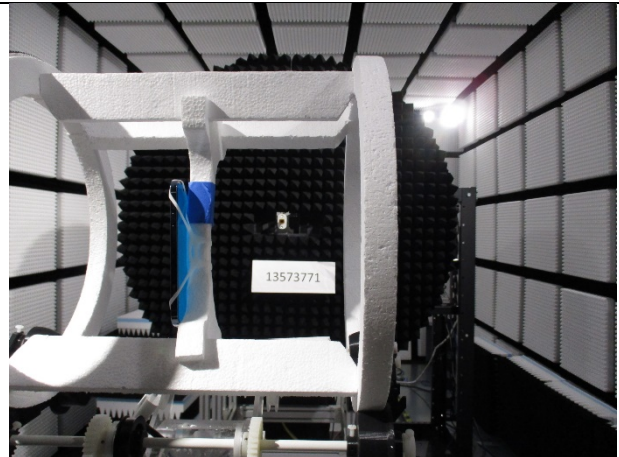
110 - 170 GHz (BACK)
