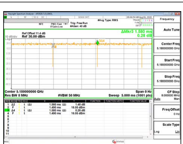
802.11ax HE20 1Tx, MCS11
