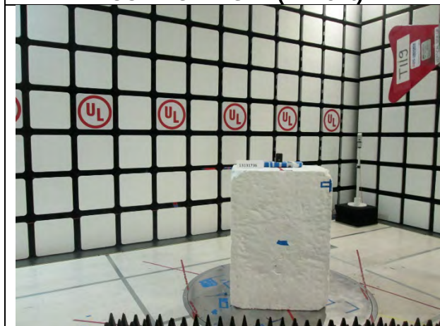
FCC ABOVE1GHz (Z Front)
