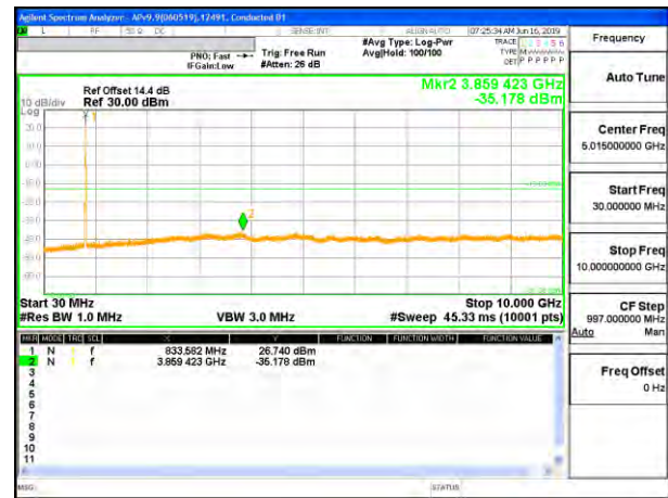
LTE B5 10MHz + 10MHz 16QAM Low Ch RB1-49 + RB1-0
