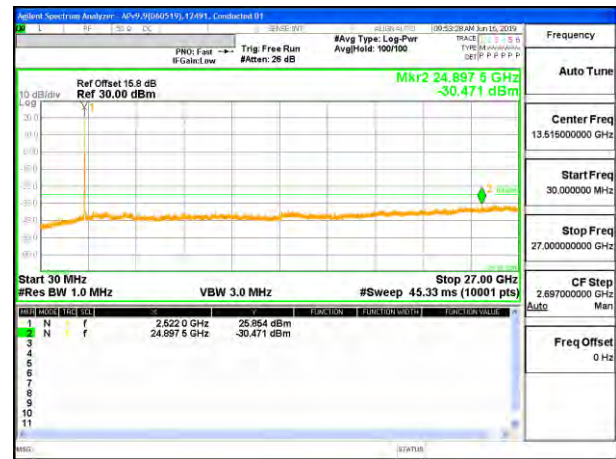
LTE B7 20MHz + 20MHz 16QAM Low Ch RB1-99 + RB1-0
