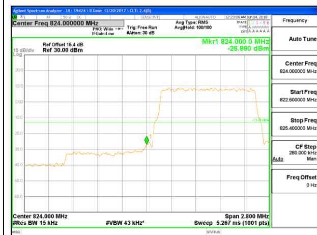
LTE B5 1.4MHz QPSK Low Channel RB6-0
