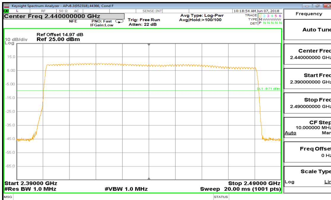
100MHz SPAN
