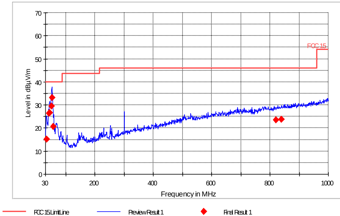
FCC 15 30-1000MHz
