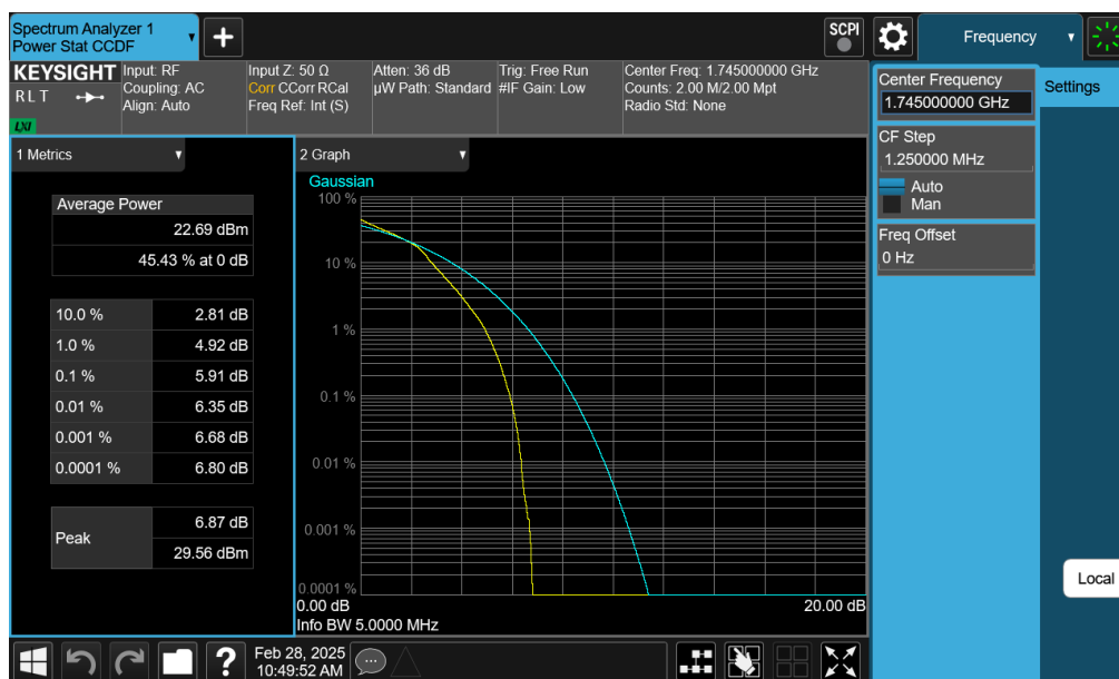
Plot 7-247. PAR Plot (LTE Band 66 - 5MHz 16-QAM - Full RB)
