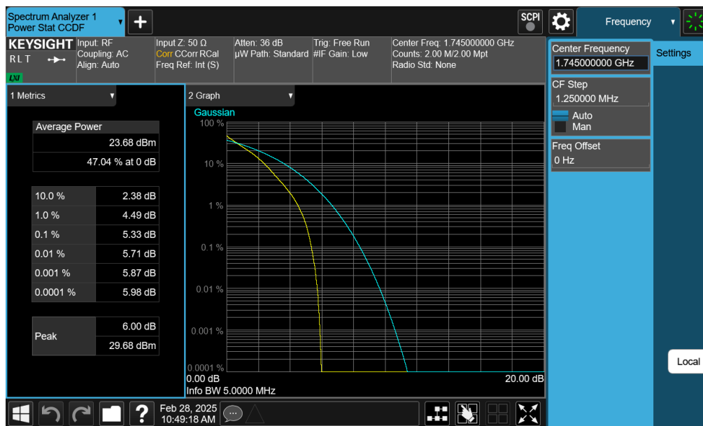
Plot 7-246. PAR Plot (LTE Band 66 - 5MHz QPSK - Full RB)
