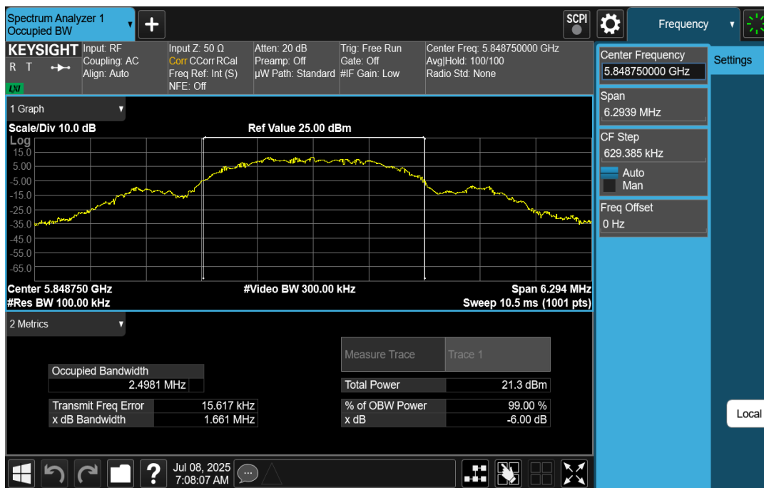
Plot 7-6. 6dB BW & 99% OBW (O-QPSK – 5848.75MHz, 500kbps)
