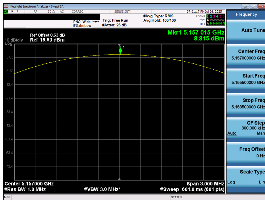
Plot 7-49. PSD (NB UNII LE2M - 5157MHz)
