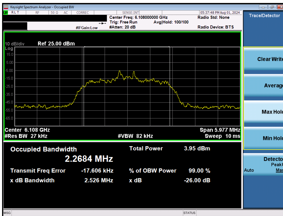
Plot 7-7. 26dB BW & 99% OBW (NB UNII HDR4 – 6108MHz)
