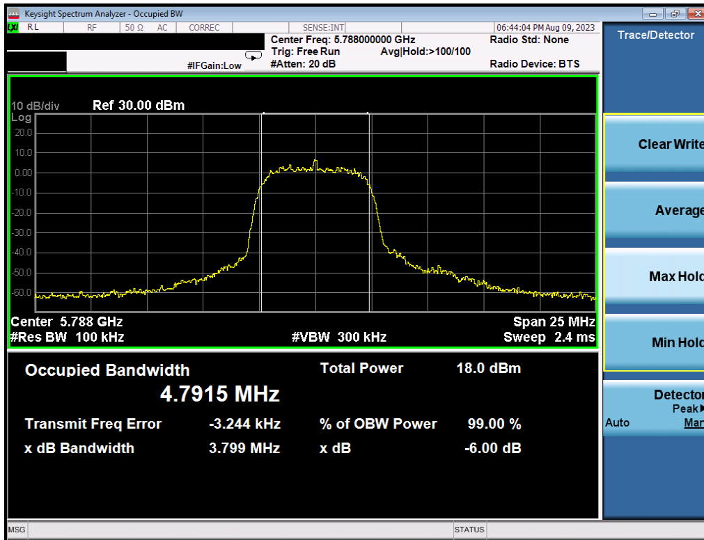
Plot 7-23. 6dB BW & 99% OBW (HDRp8, 5788MHz)
