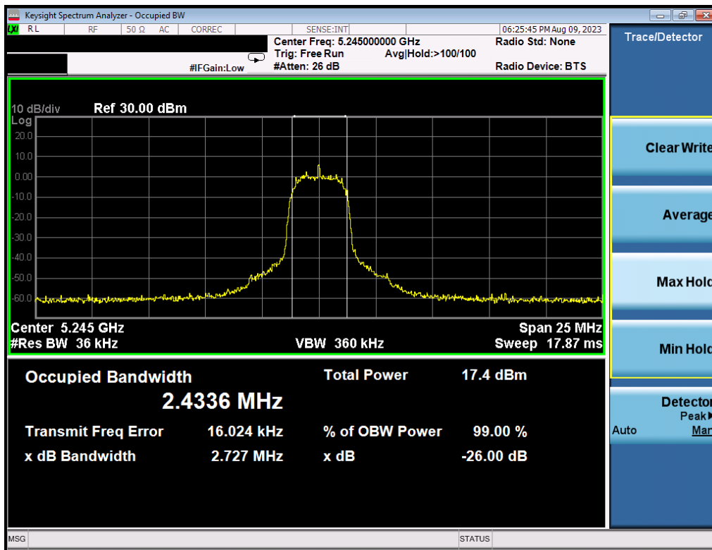
Plot 7-9. 26dB BW & 99% OBW (HDRp4, 5245MHz)
