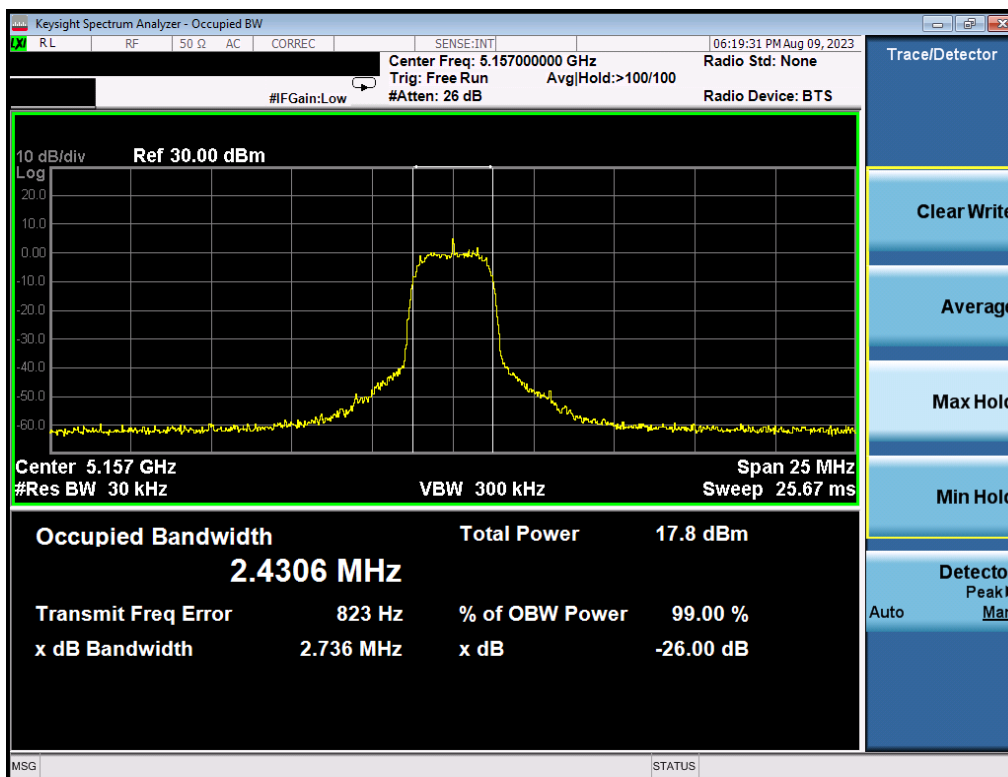
Plot 7-7. 26dB BW & 99% OBW (HDRp4, 5157MHz)
