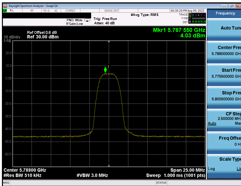
Plot 7-44. PSD (HDRp4, 5788MHz)
