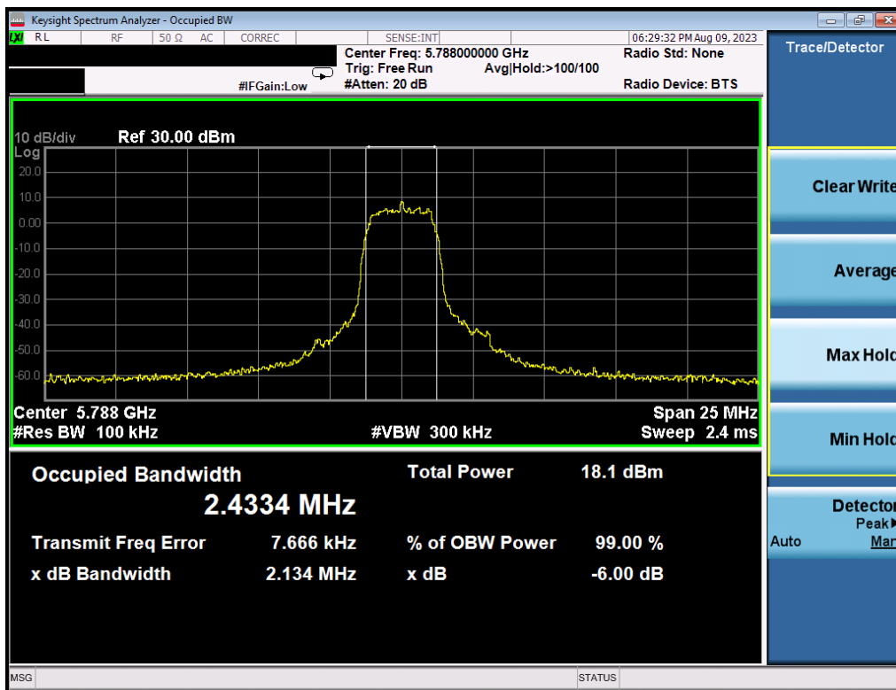
Plot 7-20. 6dB BW & 99% OBW (HDRp4, 5788MHz)
