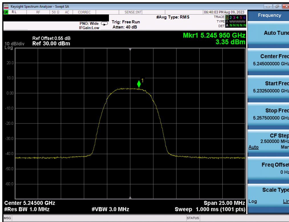
Plot 7-36. PSD (HDRp8, 5245MHz)
