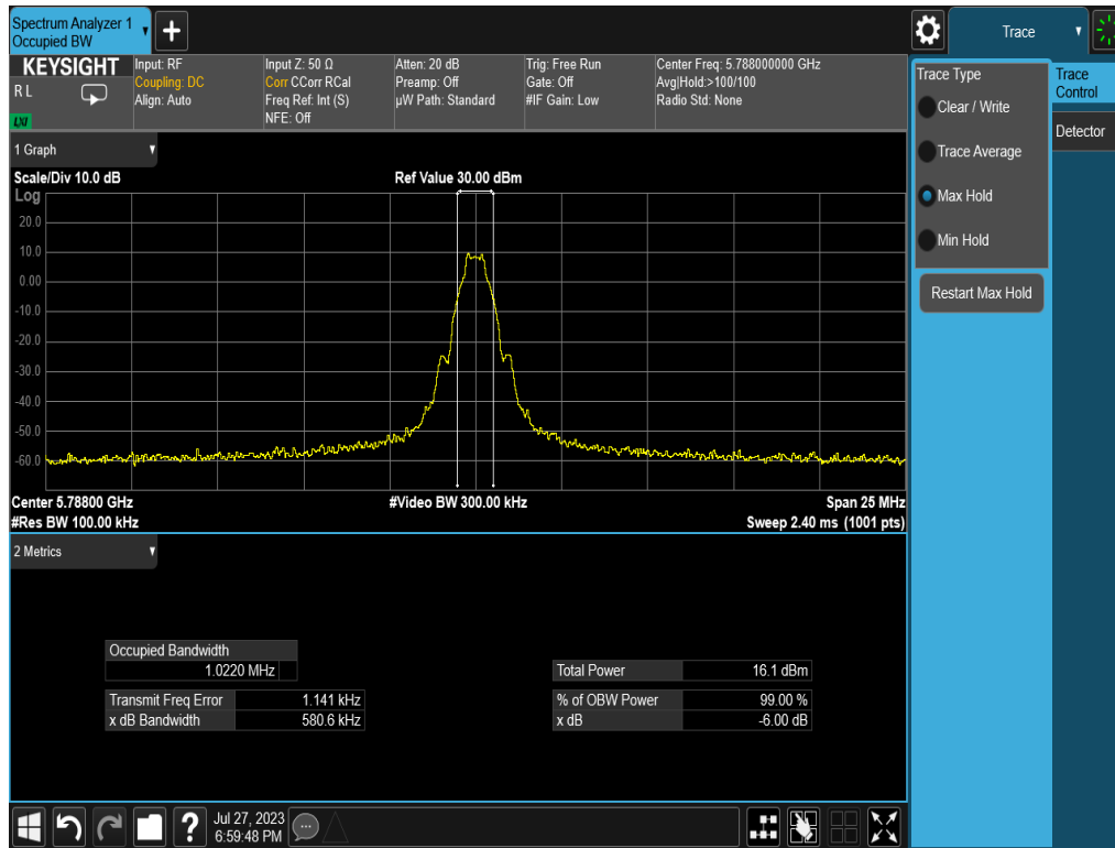
Plot 7-5. 6dB BW & 99% OBW (BDR, 5788MHz)
