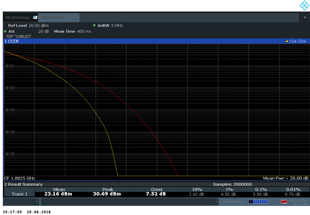
Plot 7-94. PAR Plot (LTE Band 25 - 5MHz QPSK - Full RB Configuration)
