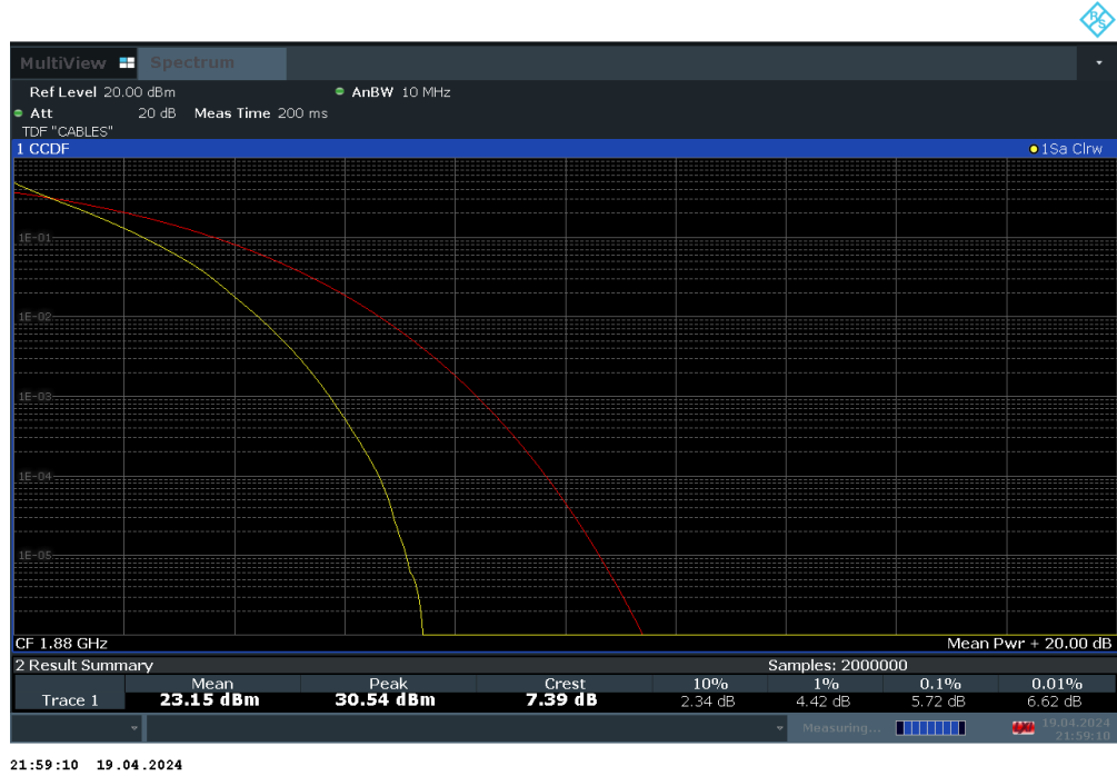
Plot 7-108. PAR Plot (LTE Band 2 - 10MHz QPSK - Full RB Configuration)
