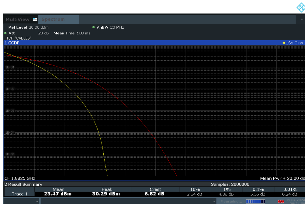
Plot 7-100. PAR Plot (LTE Band 25 - 20MHz QPSK - Full RB Configuration)
