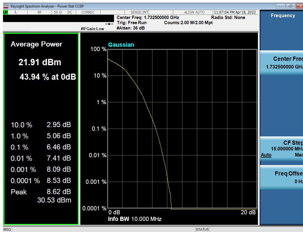
Plot 7-147. PAR Plot (LTE Band 4 - 10MHz 16-QAM - Full RB)
