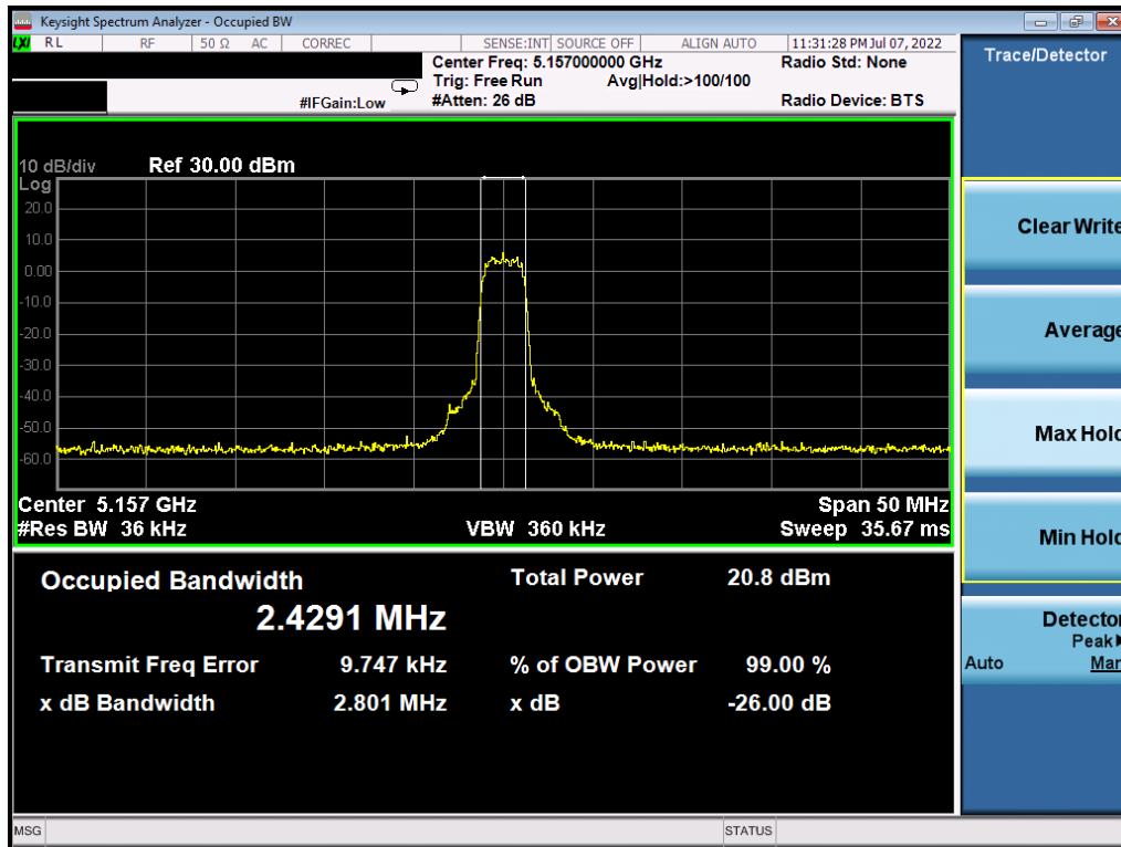
Plot 7-7. 26dB BW & 99% OBW (HDRp4, 5157MHz)
