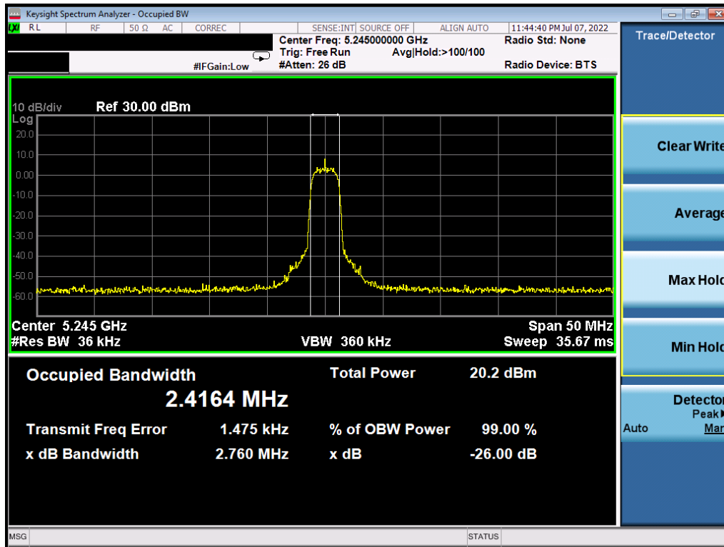
Plot 7-9. 26dB BW & 99% OBW (HDRp4, 5245MHz)
