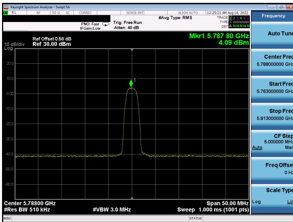
Plot 7-44. PSD (HDRp4, 5788MHz)
