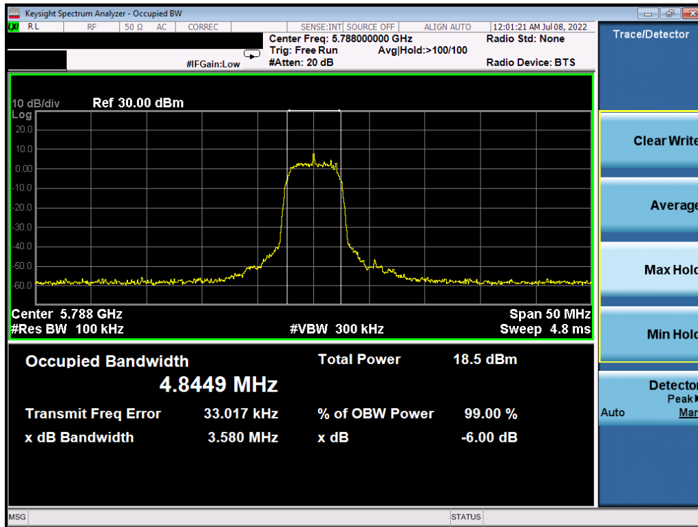
Plot 7-23. 6dB BW & 99% OBW (HDRp8, 5788MHz)
