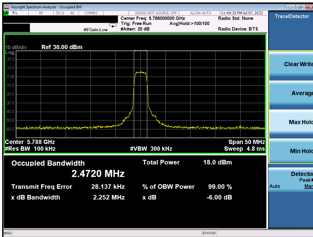
Plot 7-20. 6dB BW & 99% OBW (HDRp4, 5788MHz)
